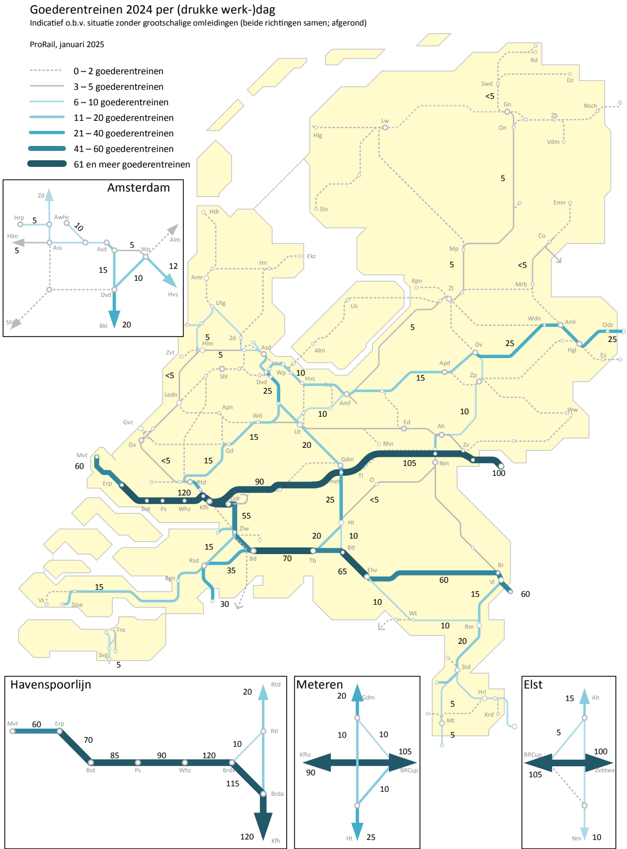
Figuur BI.3: Aantal goederentreinen op een (drukke) werkdag in 2024 in situatie zonder omleidingen vanwege de bouw van het 3e spoor Zevenaar – Oberhausen
