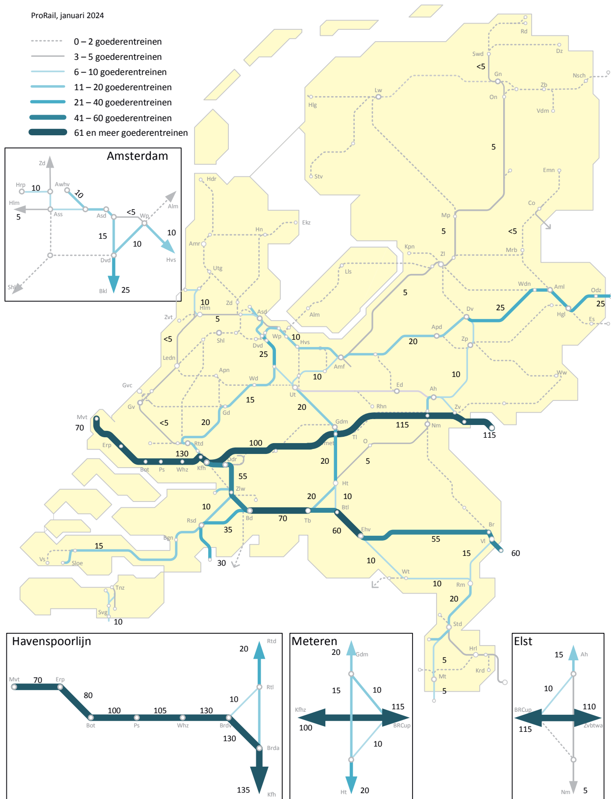
Figuur BI.1: Aantal goederentreinen op een (drukke) werkdag in 2023 in situatie zonder omleidingen vanwege de bouw van het 3e spoor Zevenaar – Oberhausen
