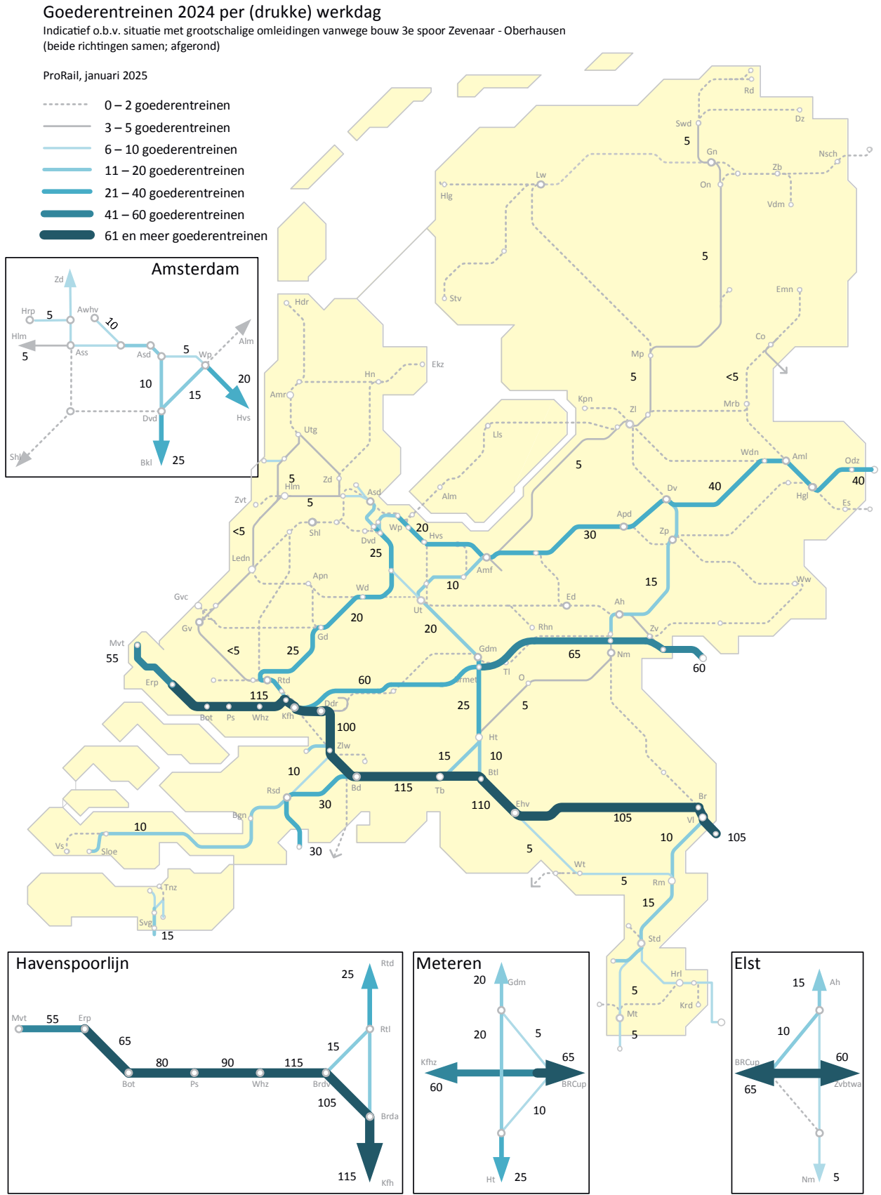
Figuur BI.4: Aantal goederentreinen op een (drukke) werkdag in 2024 in situatie met omleidingen vanwege de bouw van het 3e spoor Zevenaar – Oberhausen
