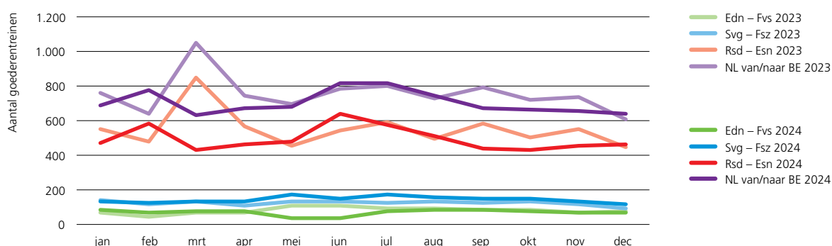
Grafiek 4.5: Ontwikkeling aantal goederentreinen per maand op de drie drukste Noord – Zuid grensovergangen 8 inclusief het totaal op de grens
