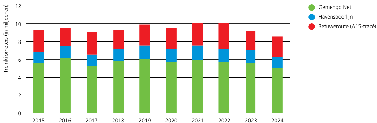
Grafiek B.III.6: Ontwikkeling aantal treinkilometers in de periode 2015-2024
