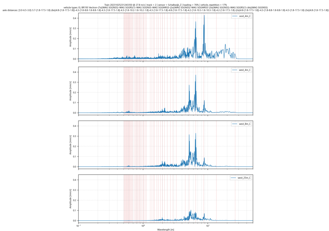
Afbeelding I.32 Amplitude spectrum voor trillingssnelheid in Z-richting op 4 meetpunten in Schalkwijk voor goederentrein passage op spoor 2 op 25-10-2023
