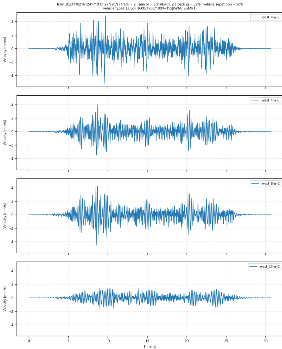
Afbeelding I.46 Trillingssnelheid in Z-richting op 4 meetpunten in Schalkwijk voor goederentrein passage op spoor 2 op 02-11-2023
