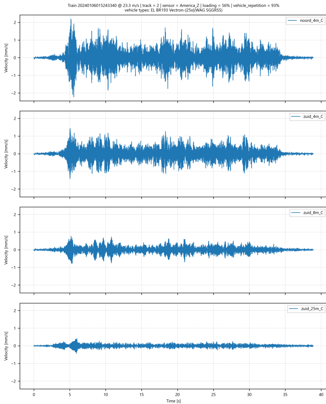
Afbeelding II.58 Trillingssnelheid in Z-richting op 4 meetpunten in America voor goederentrein passage op spoor 2 op 06-01-2024
