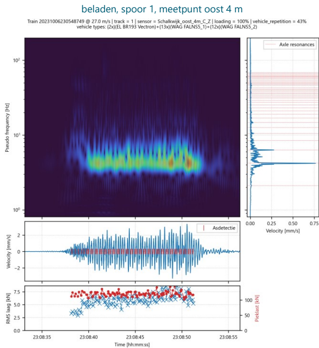
Afbeelding 4.3 Tijd-frequentie plots voor trillingssnelheid in Z-richting op 5 meetpunten in Schalkwijk (onder elkaar) voor twee goederentrein passages met WAG FALNS5_1 en WAG FALNS5_2 wagons, links op spoor 1 met beladen wagons op 6-10-2023 en rechts op spoor 2 met beladen wagons op 8-11-2023
