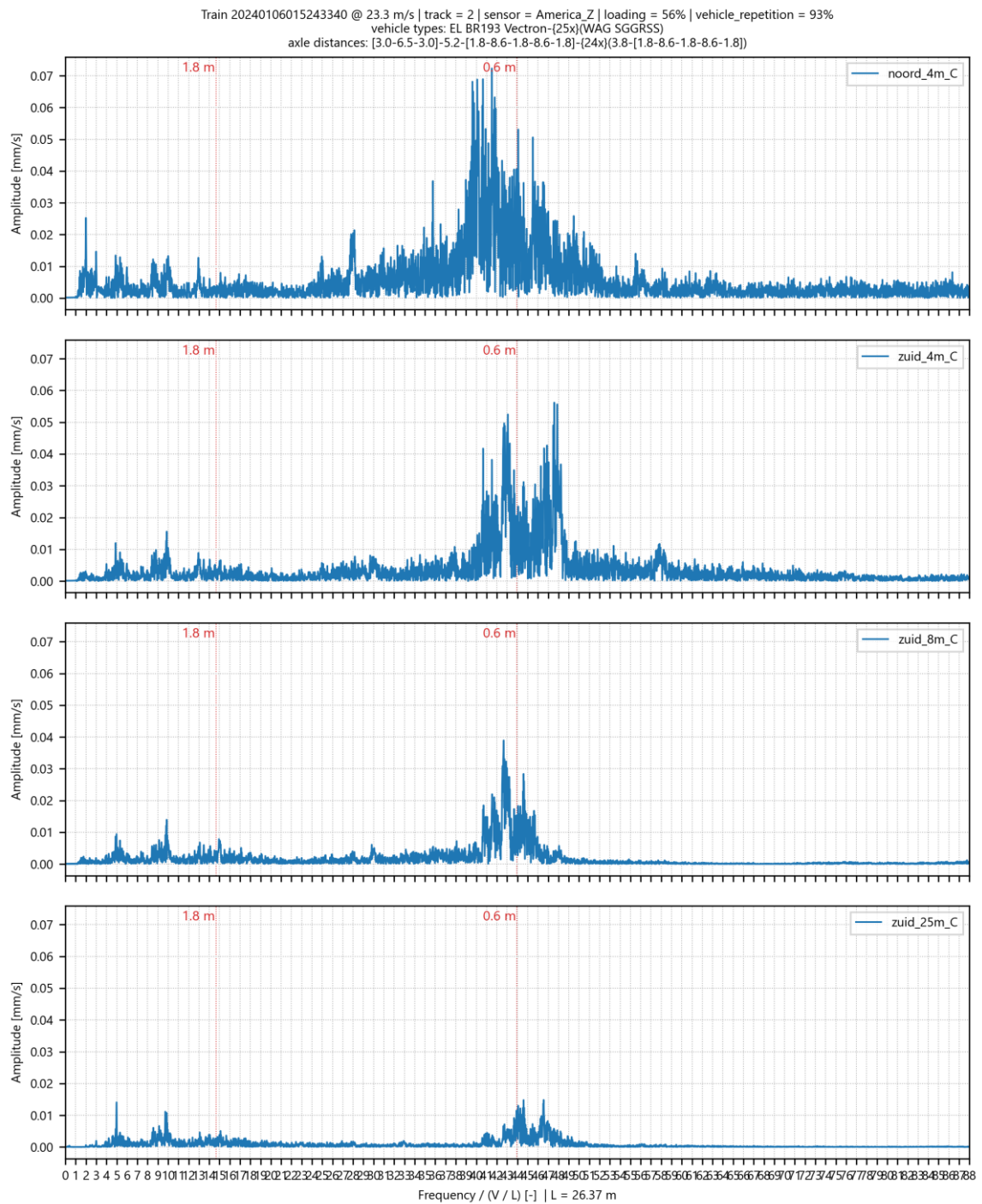
Afbeelding II.60 Genormaliseerd amplitude spectrum voor trillingssnelheid in Z-richting op 4 meetpunten in America voor goederentrein passage op spoor 2 op 06-01-2024
