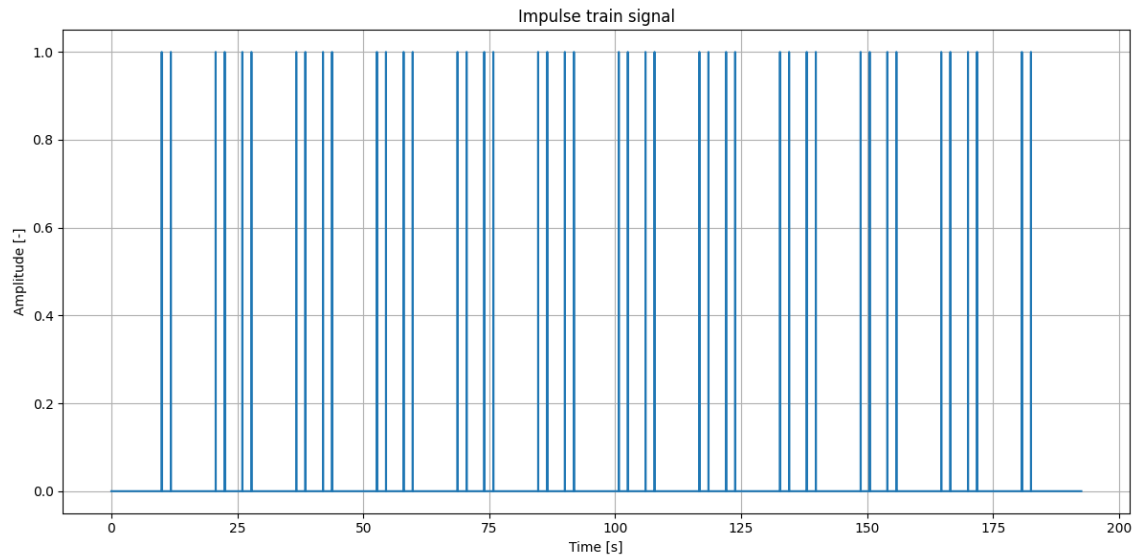
Afbeelding 3.2 Theoretische passage van aslasten van een trein met 10 identieke wagons
