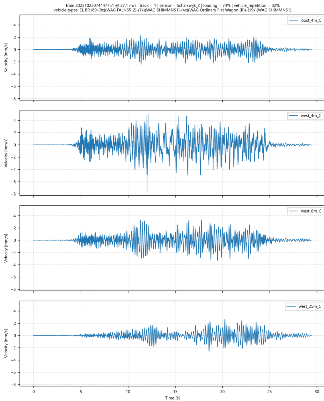
Afbeelding I.19 Trillingssnelheid in Z-richting op 4 meetpunten in Schalkwijk voor goederentrein passage op spoor 1 op 23-10-2023
