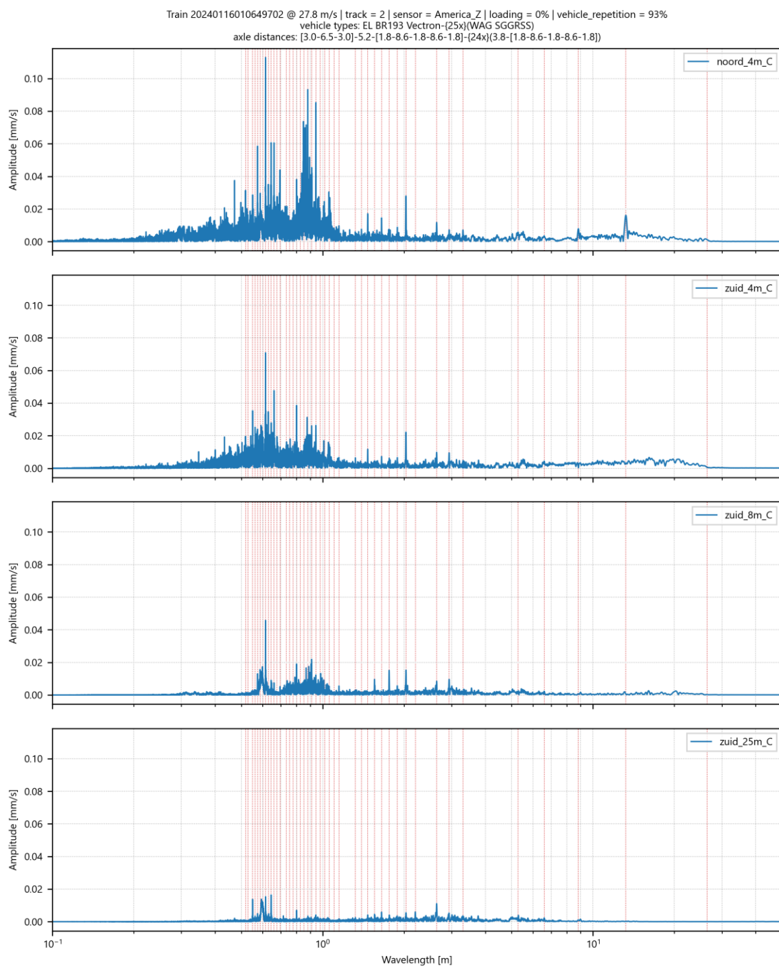
Afbeelding II.56 Amplitude spectrum voor trillingssnelheid in Z-richting op 4 meetpunten in America voor goederentrein passage op spoor 2 op 16-01-2024
