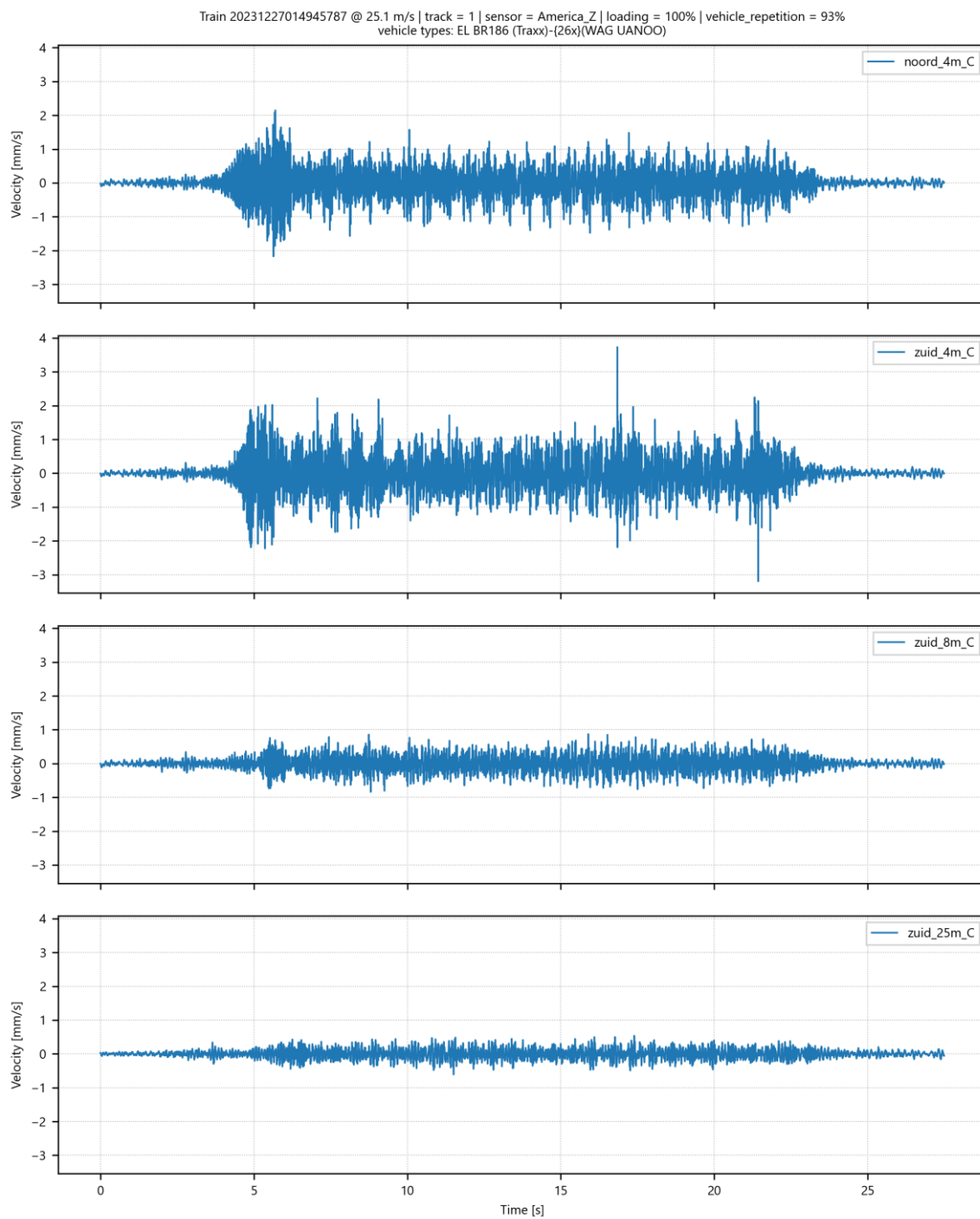
Afbeelding II.31 Trillingssnelheid in Z-richting op 4 meetpunten in America voor goederentrein passage op spoor 1 op 27-12-2023
