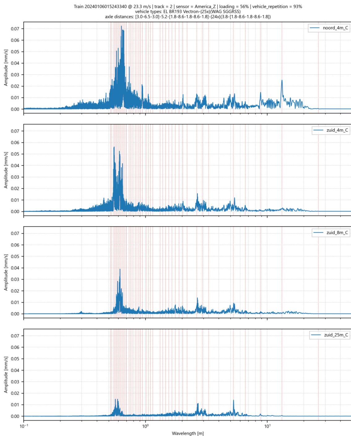
Afbeelding II.59 Amplitude spectrum voor trillingssnelheid in Z-richting op 4 meetpunten in America voor goederentrein passage op spoor 2 op 06-01-2024
