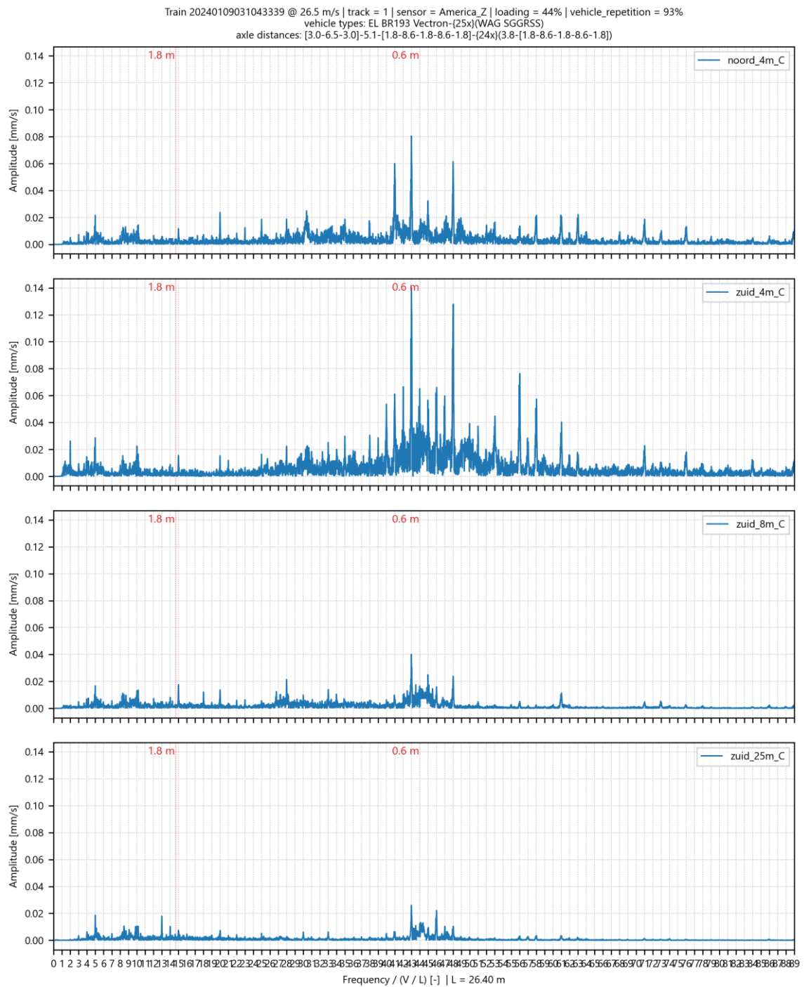
Afbeelding II.39 Genormaliseerd amplitude spectrum voor trillingssnelheid in Z-richting op 4 meetpunten in America voor goederentrein passage op spoor 1 op 09-01-2024
