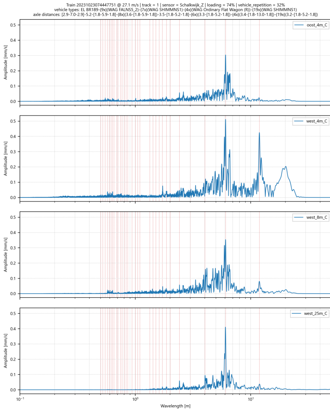
Afbeelding I.20 Amplitude spectrum voor trillingssnelheid in Z-richting op 4 meetpunten in Schalkwijk voor goederentrein passage op spoor 1 op 23-10-2023
