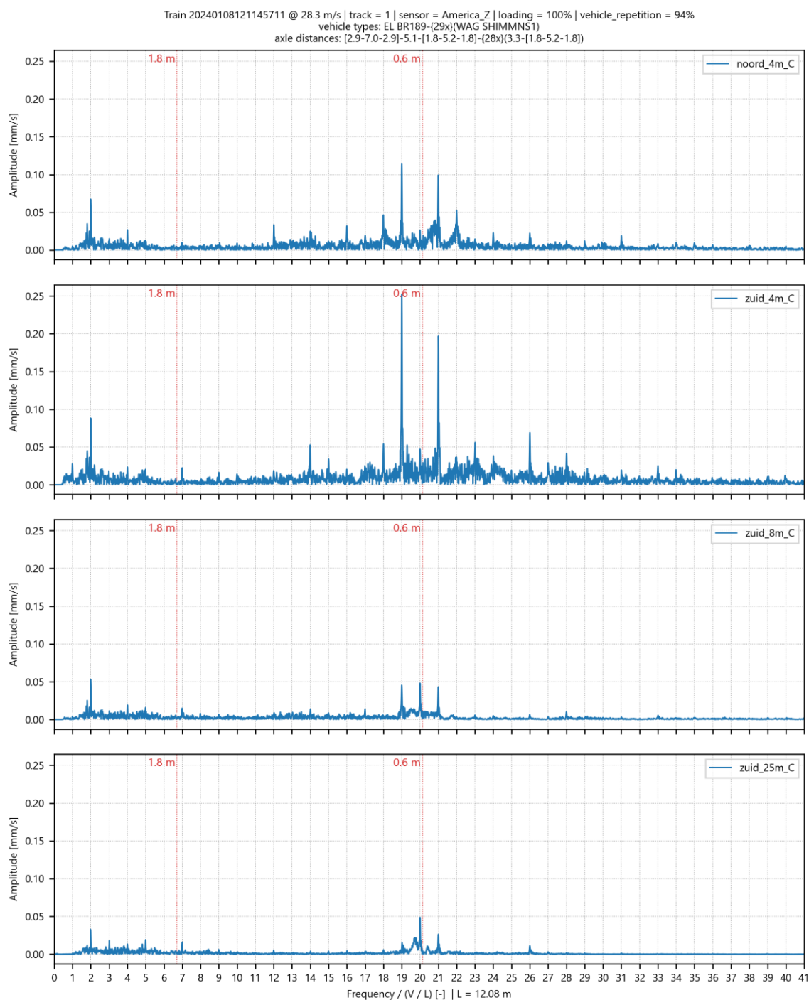
Afbeelding II.30 Genormaliseerd amplitude spectrum voor trillingssnelheid in Z-richting op 4 meetpunten in America voor goederentrein passage op spoor 1 op 08-01-2024
