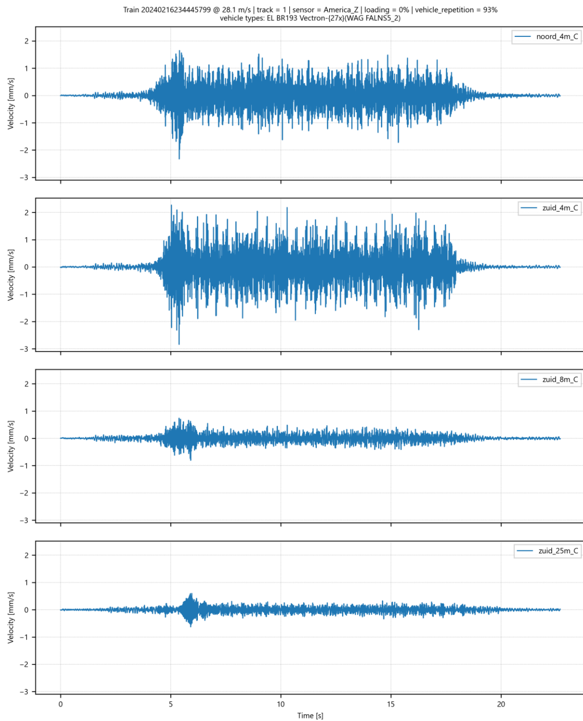
Afbeelding II.22 Trillingssnelheid in Z-richting op 4 meetpunten in America voor goederentrein passage op spoor 1 op 16-02-2024
