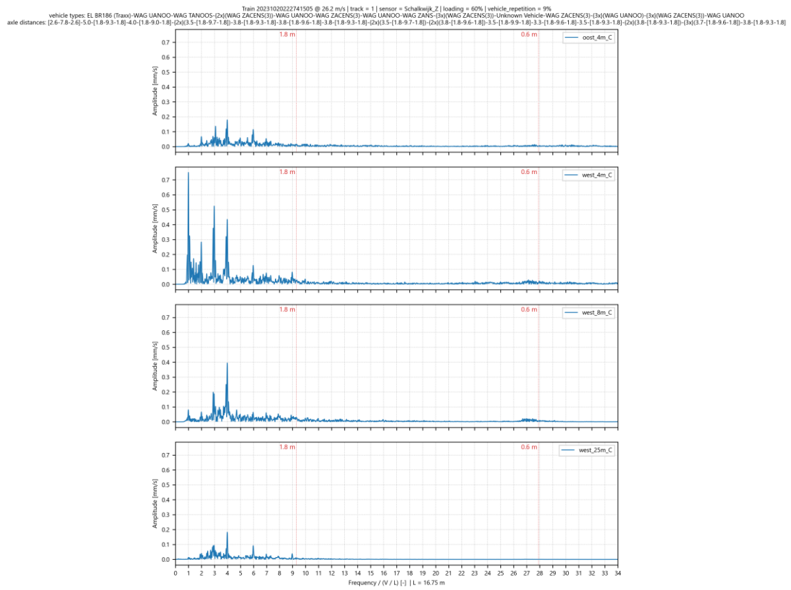
Afbeelding I.15 Genormaliseerd amplitude spectrum voor trillingssnelheid in Z-richting op 4 meetpunten in Schalkwijk voor goederentrein passage op spoor 1 op 20-10-2023
