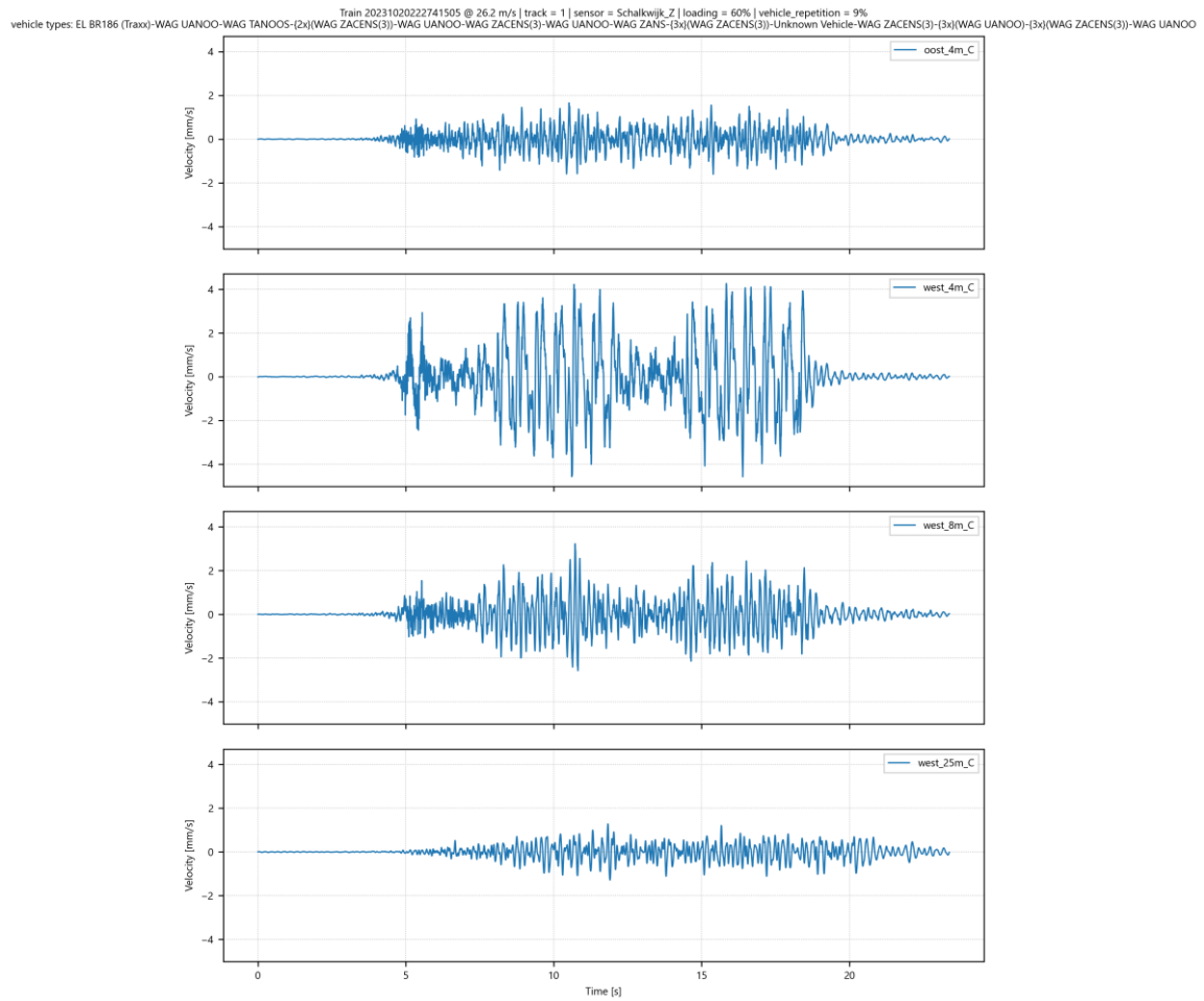
Afbeelding I.13 Trillingssnelheid in Z-richting op 4 meetpunten in Schalkwijk voor goederentrein passage op spoor 1 op 20-10-2023
