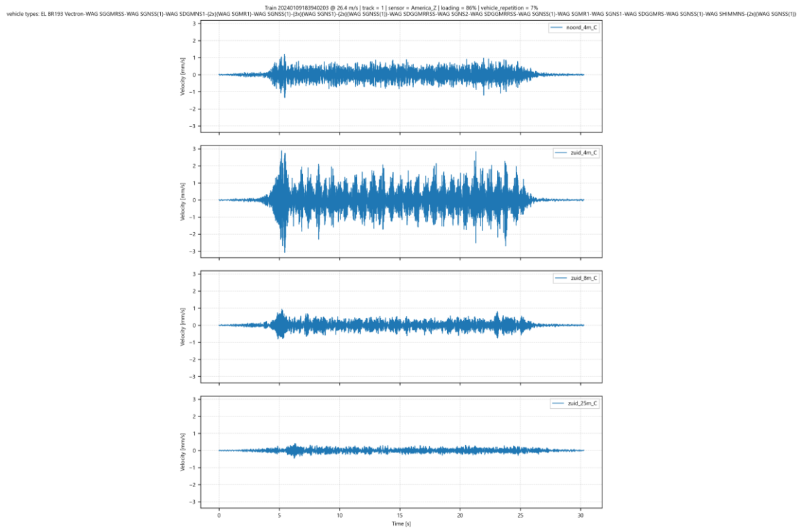
Afbeelding II.13 Trillingssnelheid in Z-richting op 4 meetpunten in America voor goederentrein passage op spoor 1 op 09-01-2024
