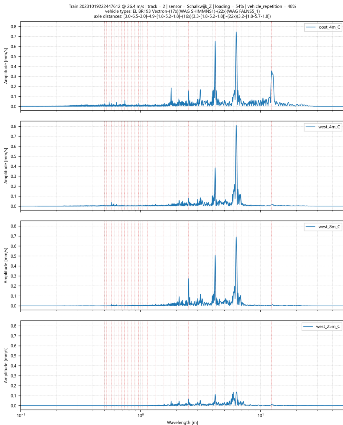
Afbeelding I.35 Amplitude spectrum voor trillingssnelheid in Z-richting op 4 meetpunten in Schalkwijk voor goederentrein passage op spoor 2 op 19-10-2023
