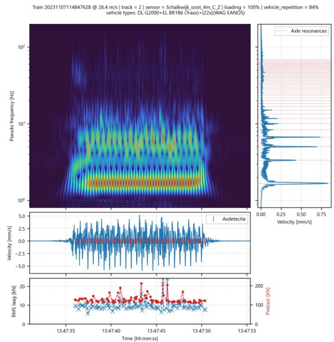
beladen, spoor 2, meetpunt oost 4 m
