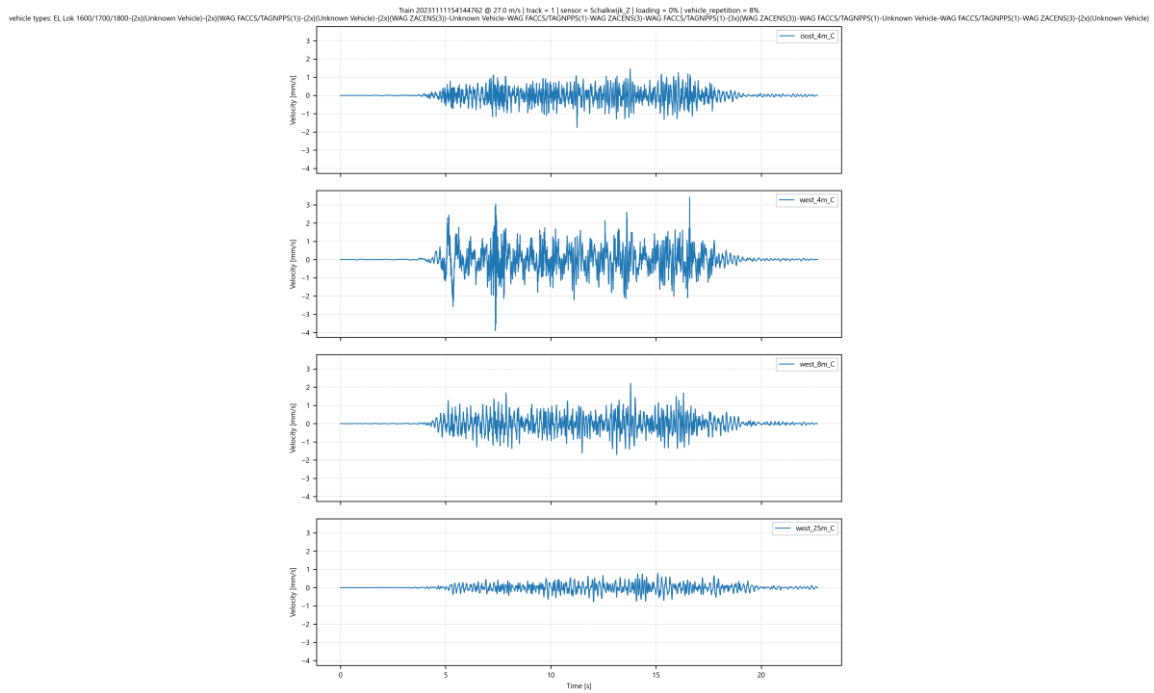
Afbeelding I.7 Trillingssnelheid in Z-richting op 4 meetpunten in Schalkwijk voor goederentrein passage op spoor 1 op 11-11-2023
