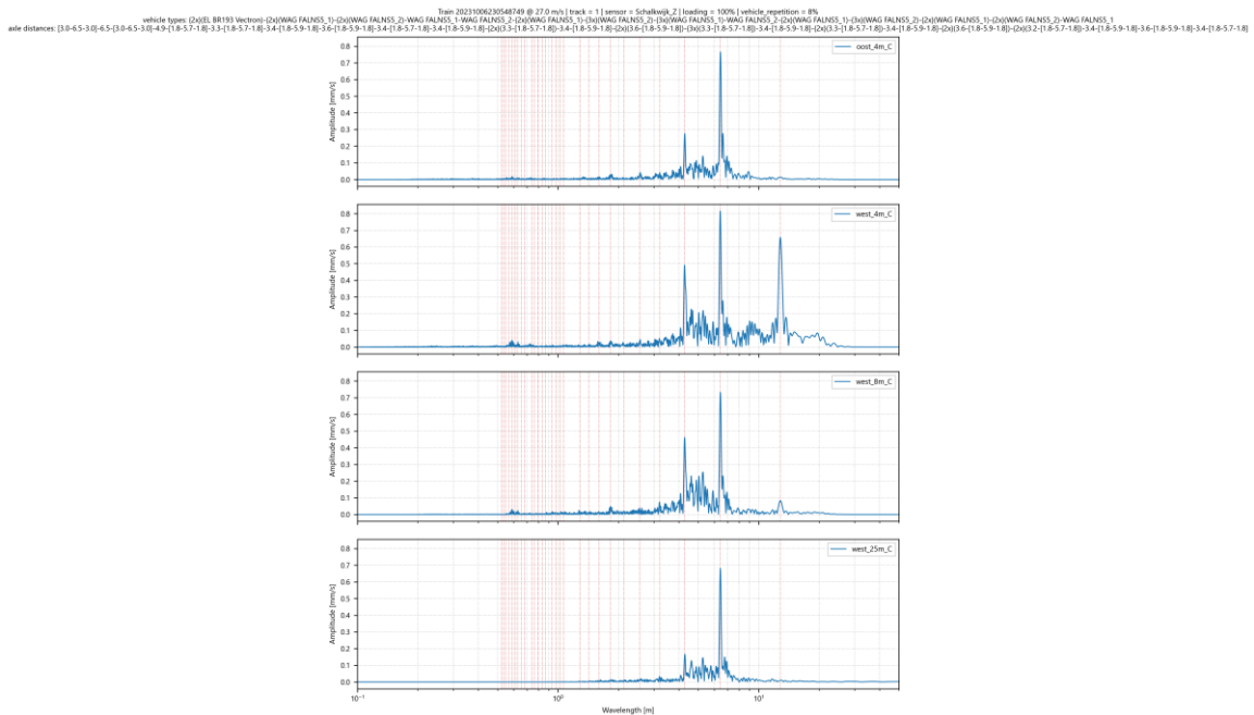
Afbeelding I.17 Amplitude spectrum voor trillingssnelheid in Z-richting op 4 meetpunten in Schalkwijk voor goederentrein passage op spoor 1 op 06-10-2023
