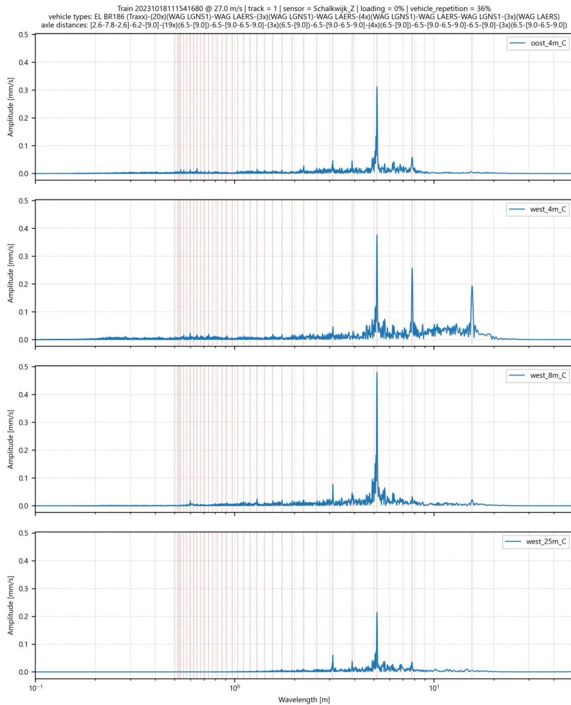
Afbeelding I.2 Amplitude spectrum voor trillingssnelheid in Z-richting op 4 meetpunten in Schalkwijk voor goederentrein passage op spoor 1 op 18-10-2023
