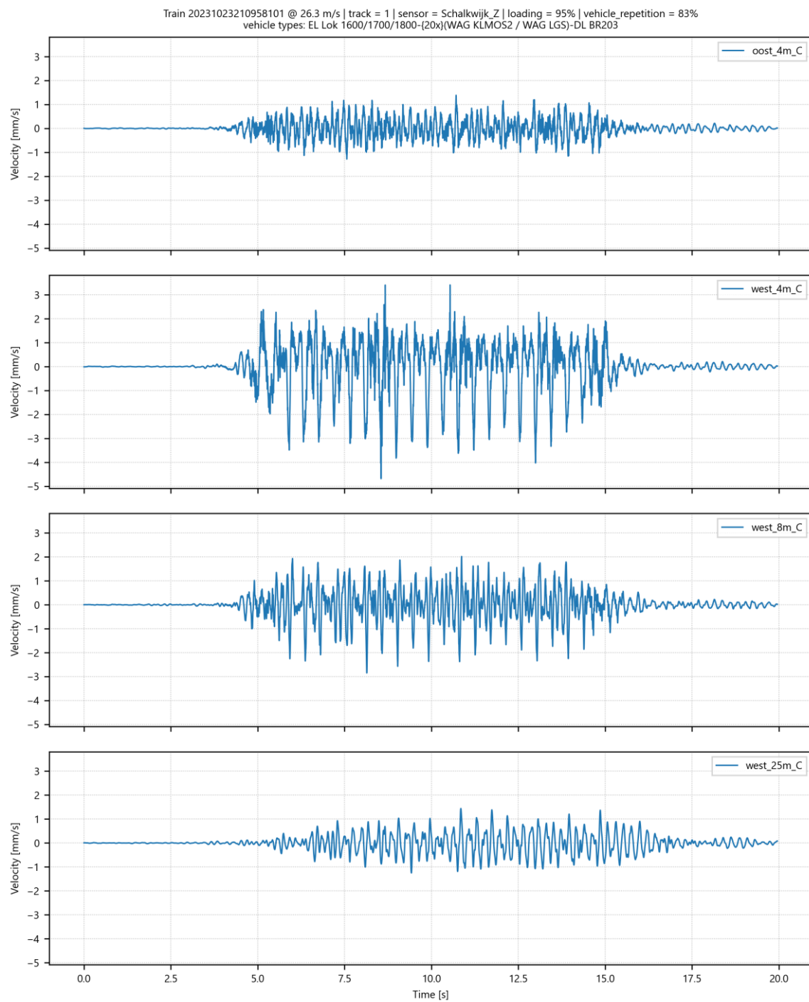
Afbeelding I.4 Trillingssnelheid in Z-richting op 4 meetpunten in Schalkwijk voor goederentrein passage op spoor 1 op 23-10-2023
