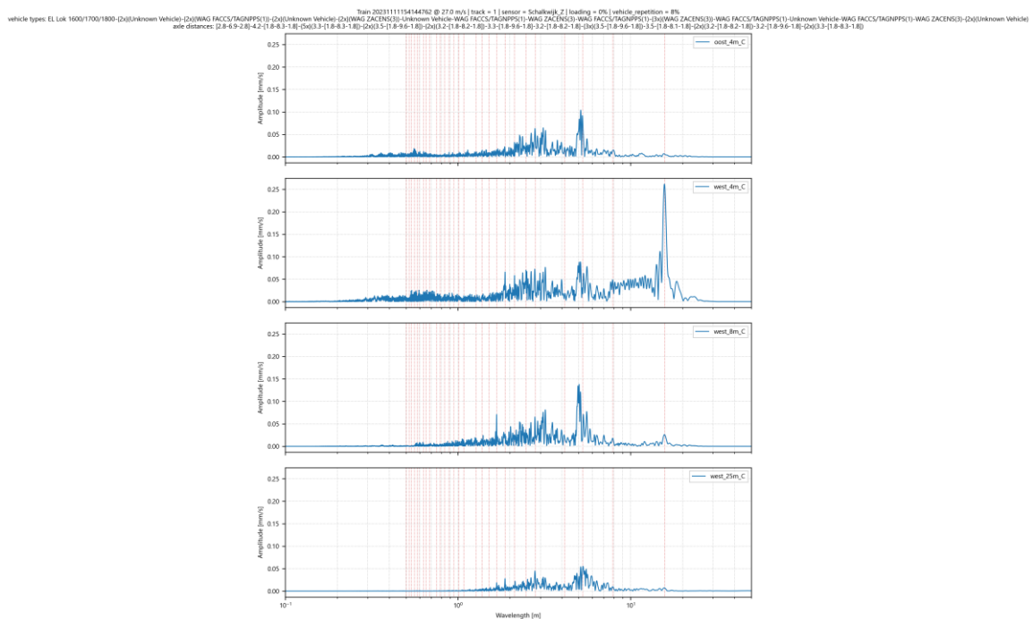
Afbeelding I.8 Amplitude spectrum voor trillingssnelheid in Z-richting op 4 meetpunten in Schalkwijk voor goederentrein passage op spoor 1 op 11-11-2023
