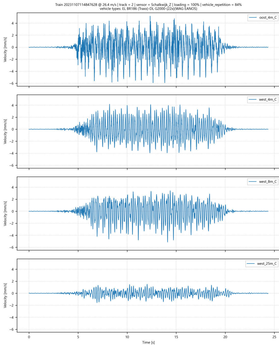
Afbeelding I.37 Trillingssnelheid in Z-richting op 4 meetpunten in Schalkwijk voor goederentrein passage op spoor 2 op 07-11-2023
