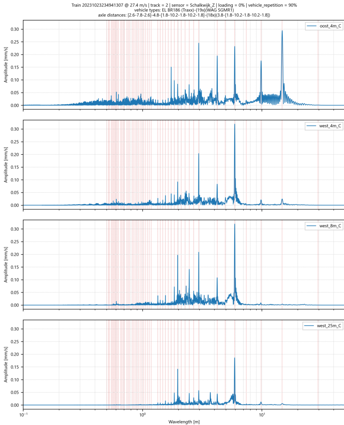
Afbeelding I.44 Amplitude spectrum voor trillingssnelheid in Z-richting op 4 meetpunten in Schalkwijk voor goederentrein passage op spoor 2 op 23-10-2023
