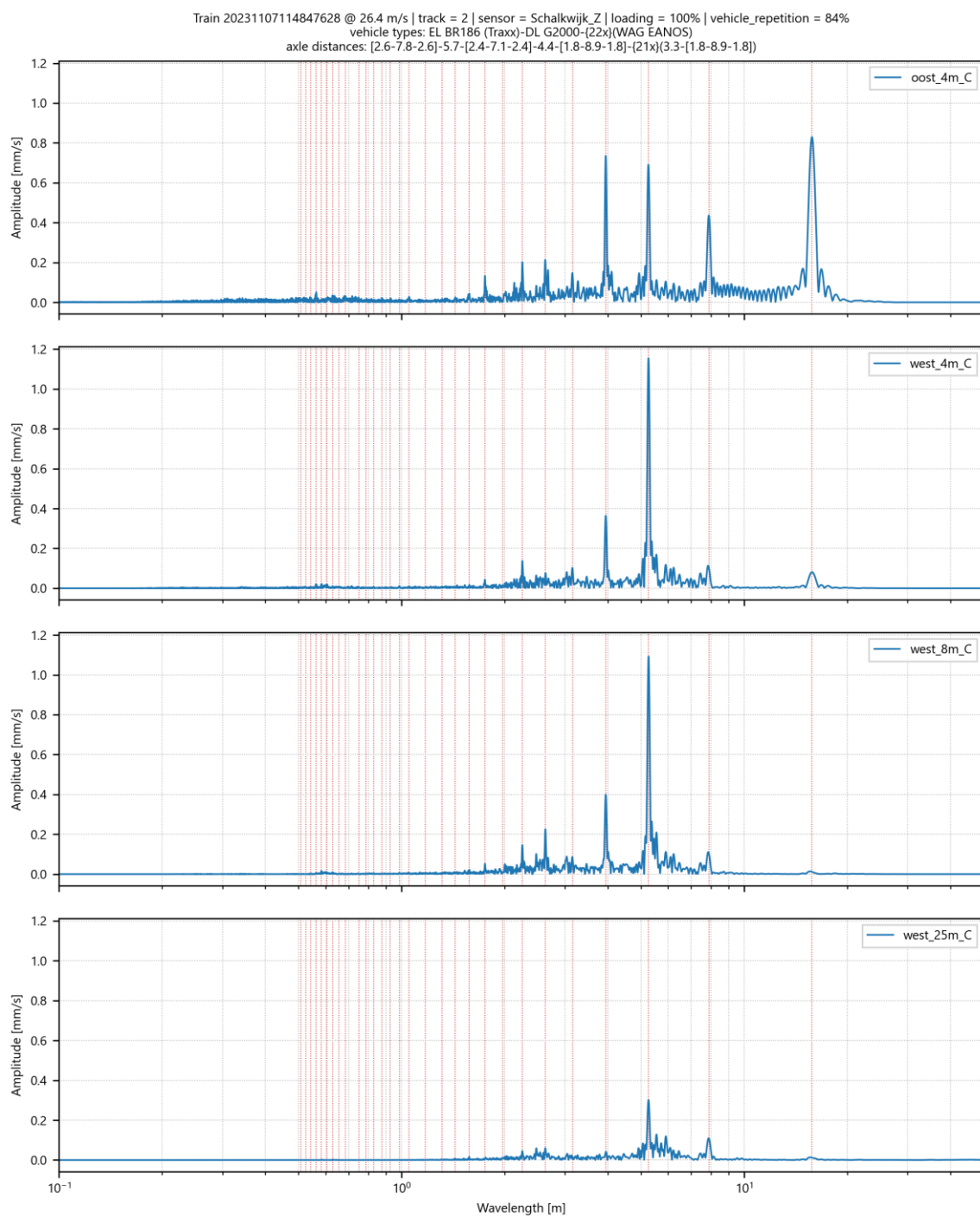
Afbeelding I.38 Amplitude spectrum voor trillingssnelheid in Z-richting op 4 meetpunten in Schalkwijk voor goederentrein passage op spoor 2 op 07-11-2023
