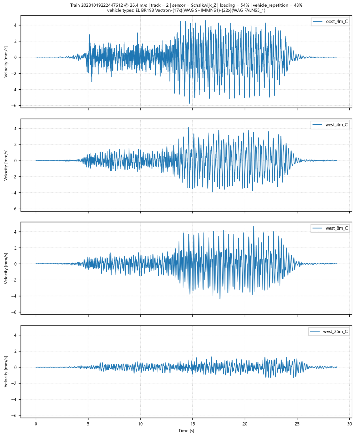
Afbeelding I.34 Trillingssnelheid in Z-richting op 4 meetpunten in Schalkwijk voor goederentrein passage op spoor 2 op 19-10-2023
