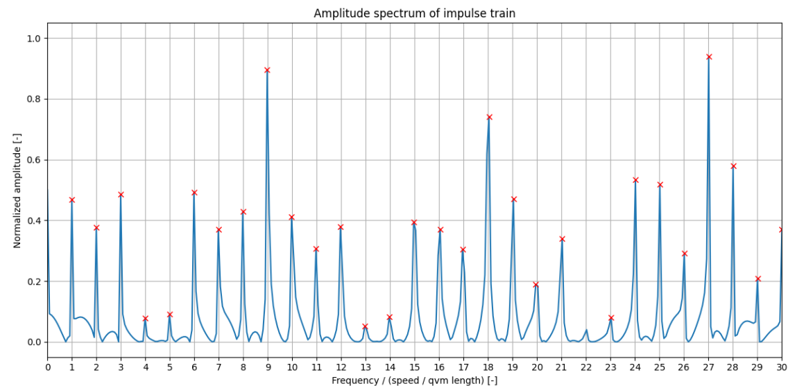
Afbeelding 3.3 Amplitude spectrum van theoretische passages van aslasten van een trein met 10 identieke wagons
