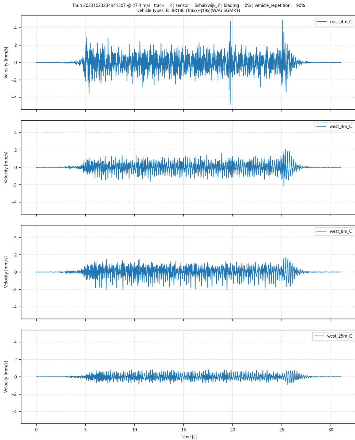
Afbeelding I.43 Trillingssnelheid in Z-richting op 4 meetpunten in Schalkwijk voor goederentrein passage op spoor 2 op 23-10-2023
