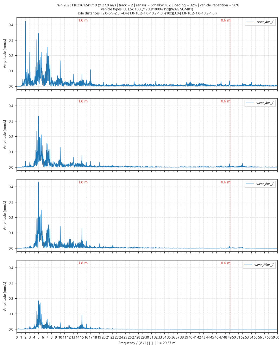
Afbeelding I.48 Genormaliseerd amplitude spectrum voor trillingssnelheid in Z-richting op 4 meetpunten in Schalkwijk voor goederentrein passage op spoor 2 op 02-11-2023
