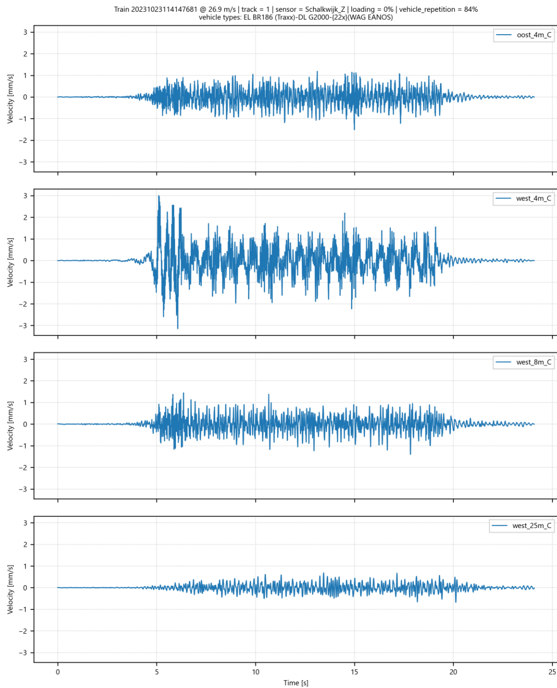
Afbeelding I.25 Trillingssnelheid in Z-richting op 4 meetpunten in Schalkwijk voor goederentrein passage op spoor 1 op 23-10-2023
