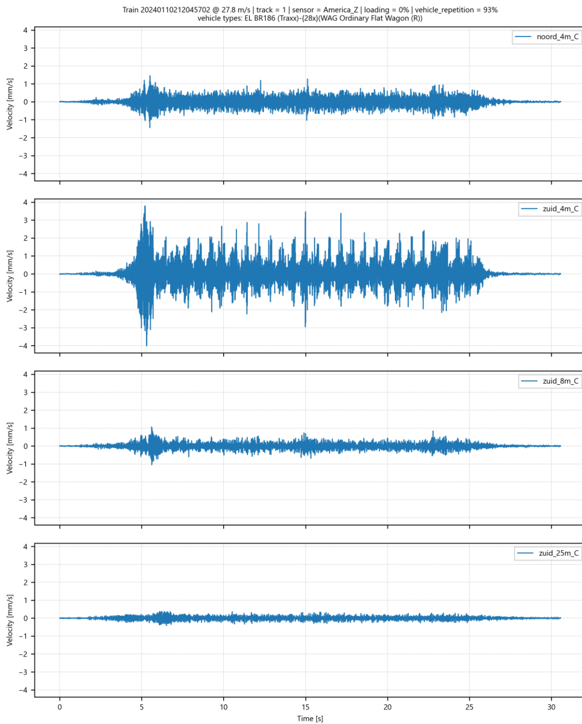
Afbeelding II.25 Trillingsnelheid in Z-richting op 4 meetpunten in America voor goederentrein passage op spoor 1 op 10-01-2024
