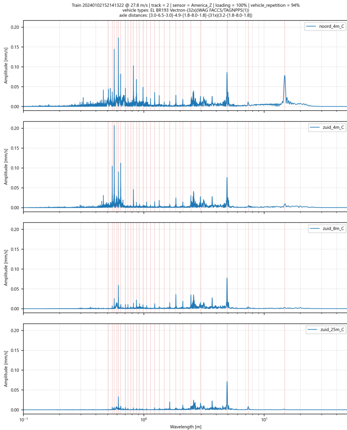
Afbeelding II.53 Amplitude spectrum voor trillingssnelheid in Z-richting op 4 meetpunten in America voor goederentrein passage op spoor 2 op 02-01-2024
