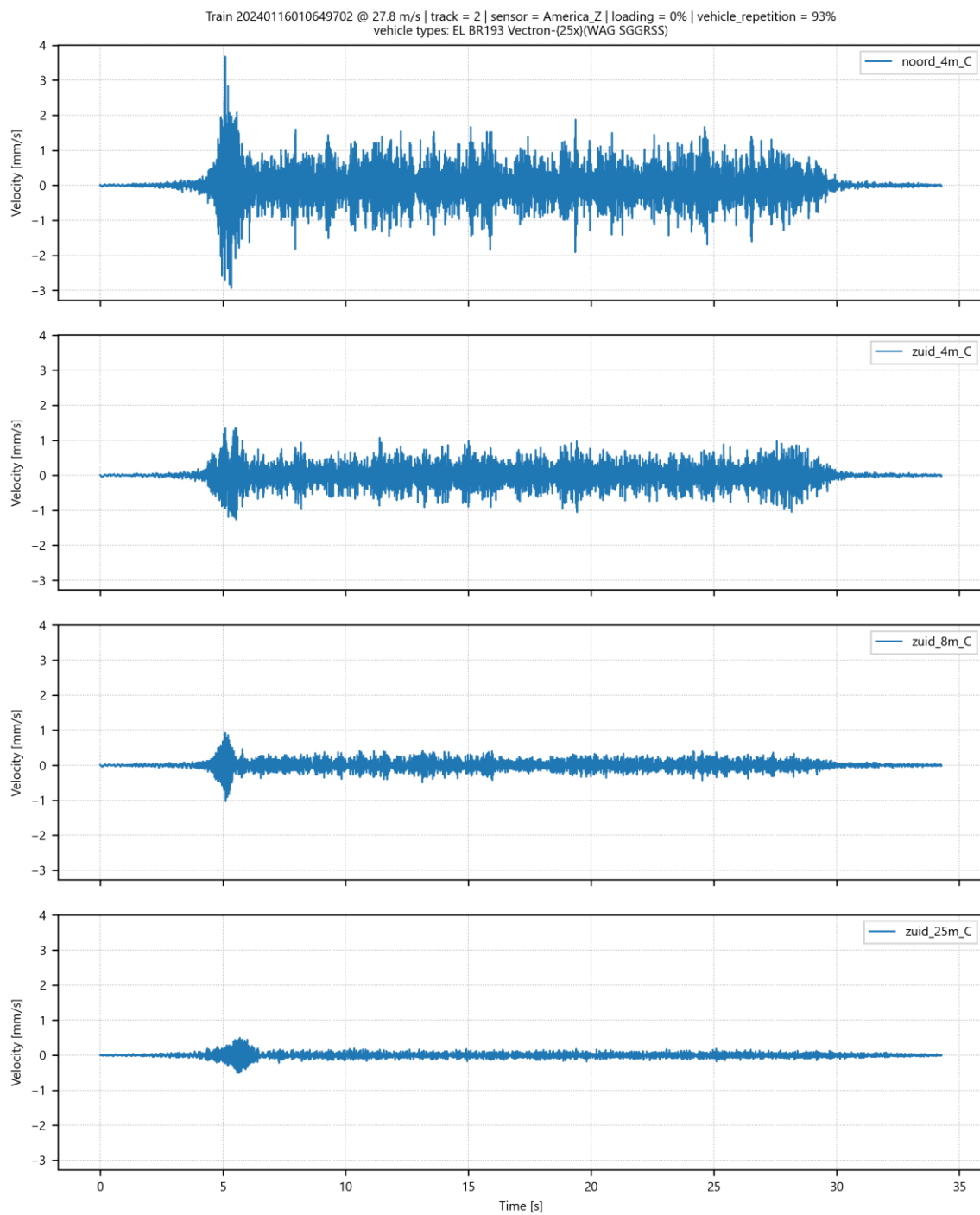
Afbeelding II.55 Trillingssnelheid in Z-richting op 4 meetpunten in America voor goederentrein passage op spoor 2 op 16-01-2024
