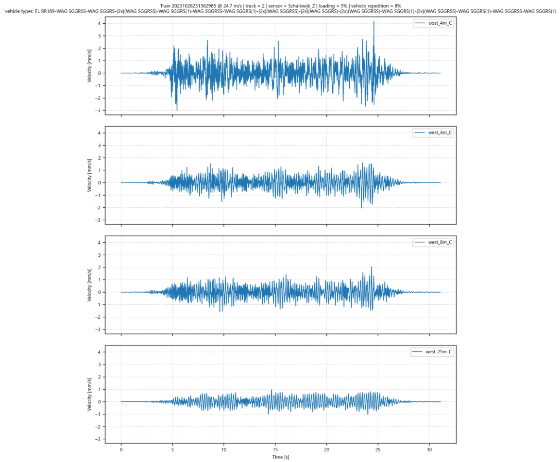
Afbeelding I.40 Trillingssnelheid in Z-richting op 4 meetpunten in Schalkwijk voor goederentrein passage op spoor 2 op 26-10-2023
