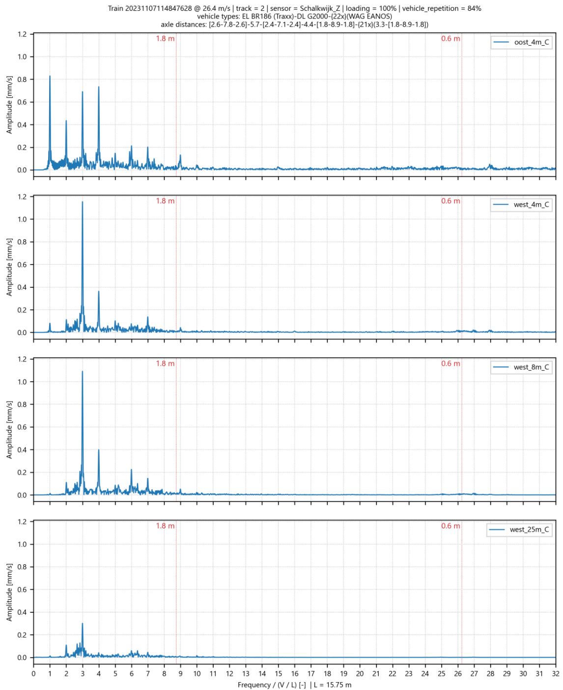
Afbeelding I.39 Genormaliseerd amplitude spectrum voor trillingssnelheid in Z-richting op 4 meetpunten in Schalkwijk voor goederentrein passage op spoor 2 op 07-11-2023
