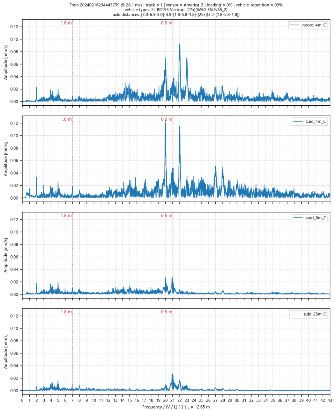
Afbeelding II.24 Genormaliseerd amplitude spectrum voor trillingssnelheid in Z-richting op 4 meetpunten in America voor goederentrein passage op spoor 1 op 16-02-2024
