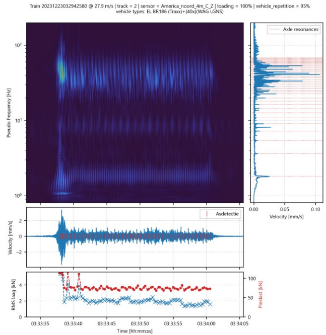
beladen, spoor 2, meetpunt noord 4 m
