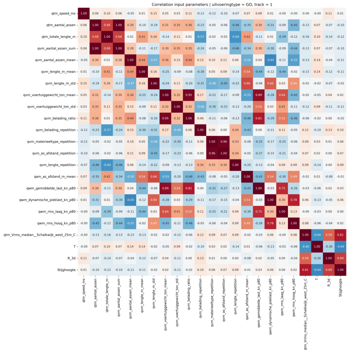
Afbeelding III.13 Correlatie coëfficiënten voor de input parameters voor goederen treinen op spoor 1
