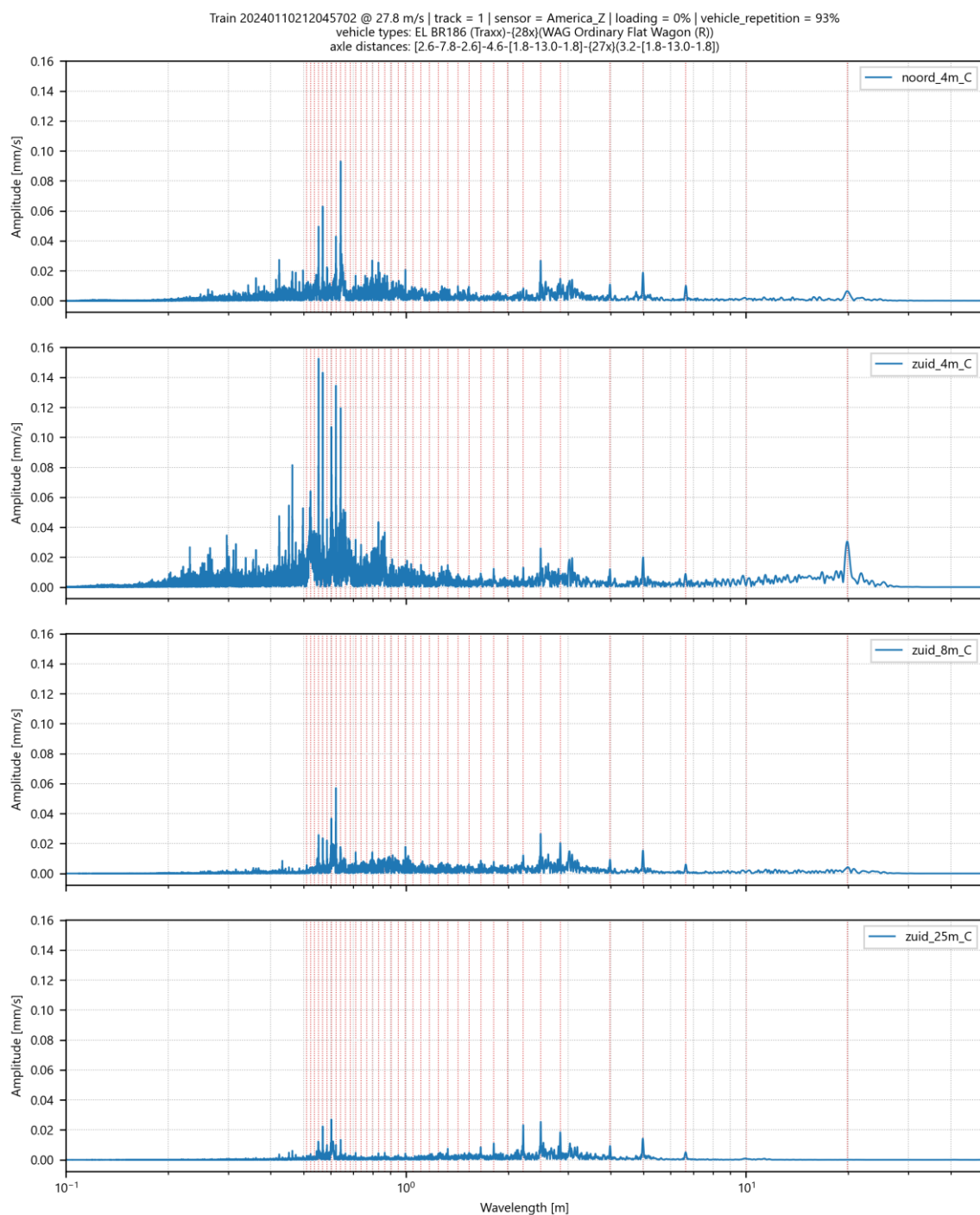
Afbeelding II.26 Amplitude spectrum voor trillingssnelheid in Z-richting op 4 meetpunten in America voor goederentrein passage op spoor 1 op 10-01-2024
