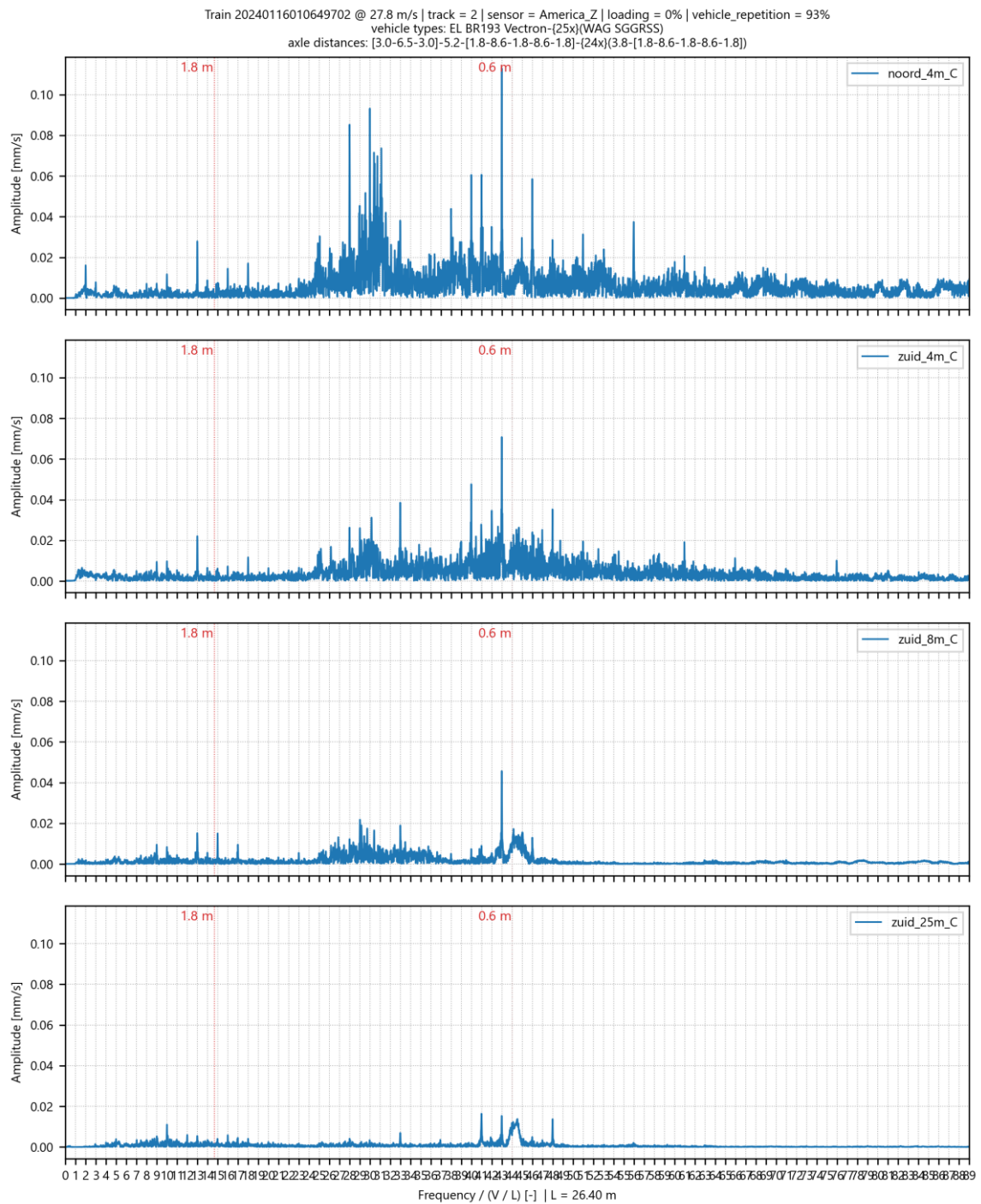
Afbeelding II.57 Genormaliseerd amplitude spectrum voor trillingssnelheid in Z-richting op 4 meetpunten in America voor goederentrein passage op spoor 2 op 16-01-2024
