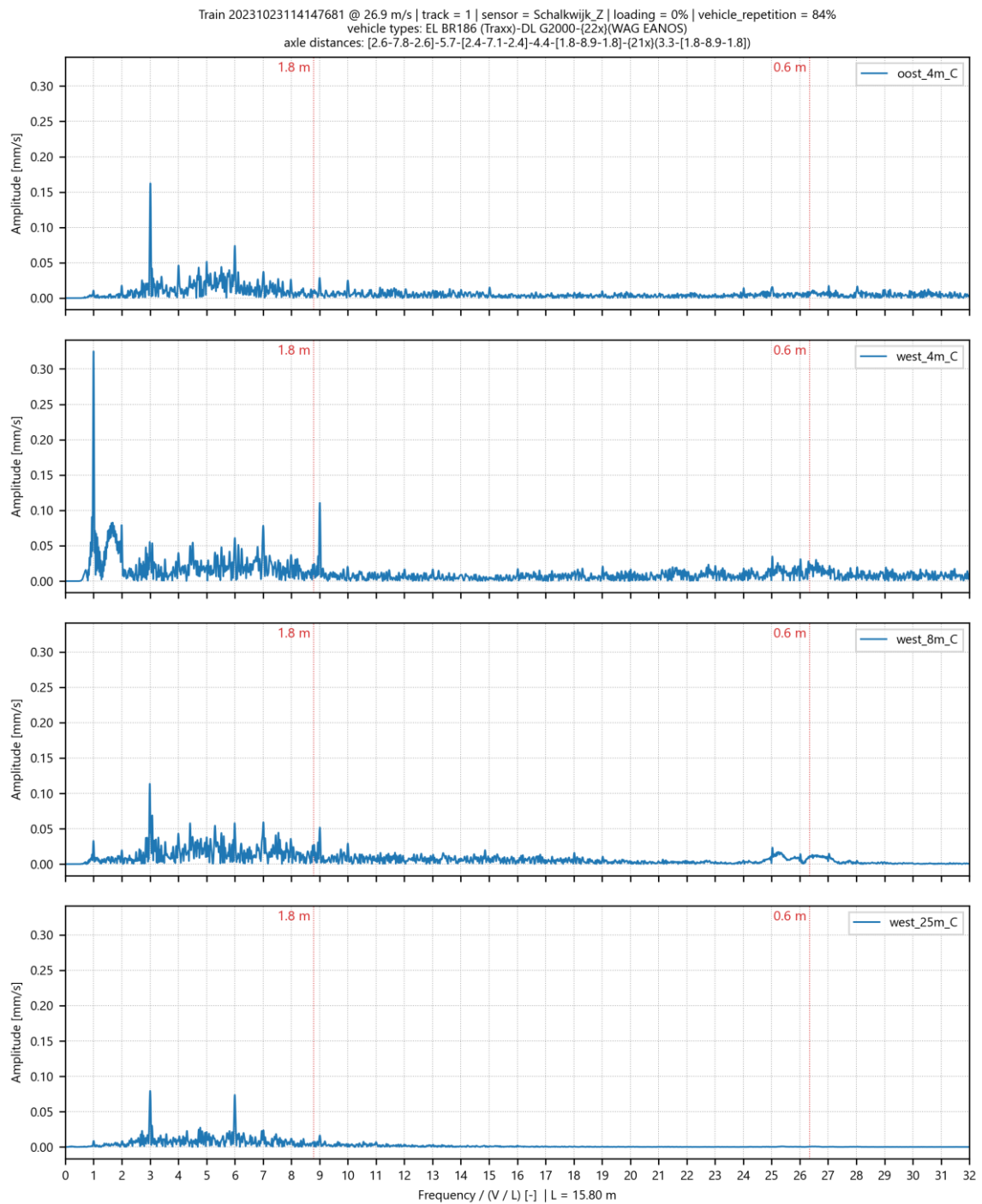
Afbeelding I.27 Genormaliseerd amplitude spectrum voor trillingssnelheid in Z-richting op 4 meetpunten in Schalkwijk voor goederentrein passage op spoor 1 op 23-10-2023
