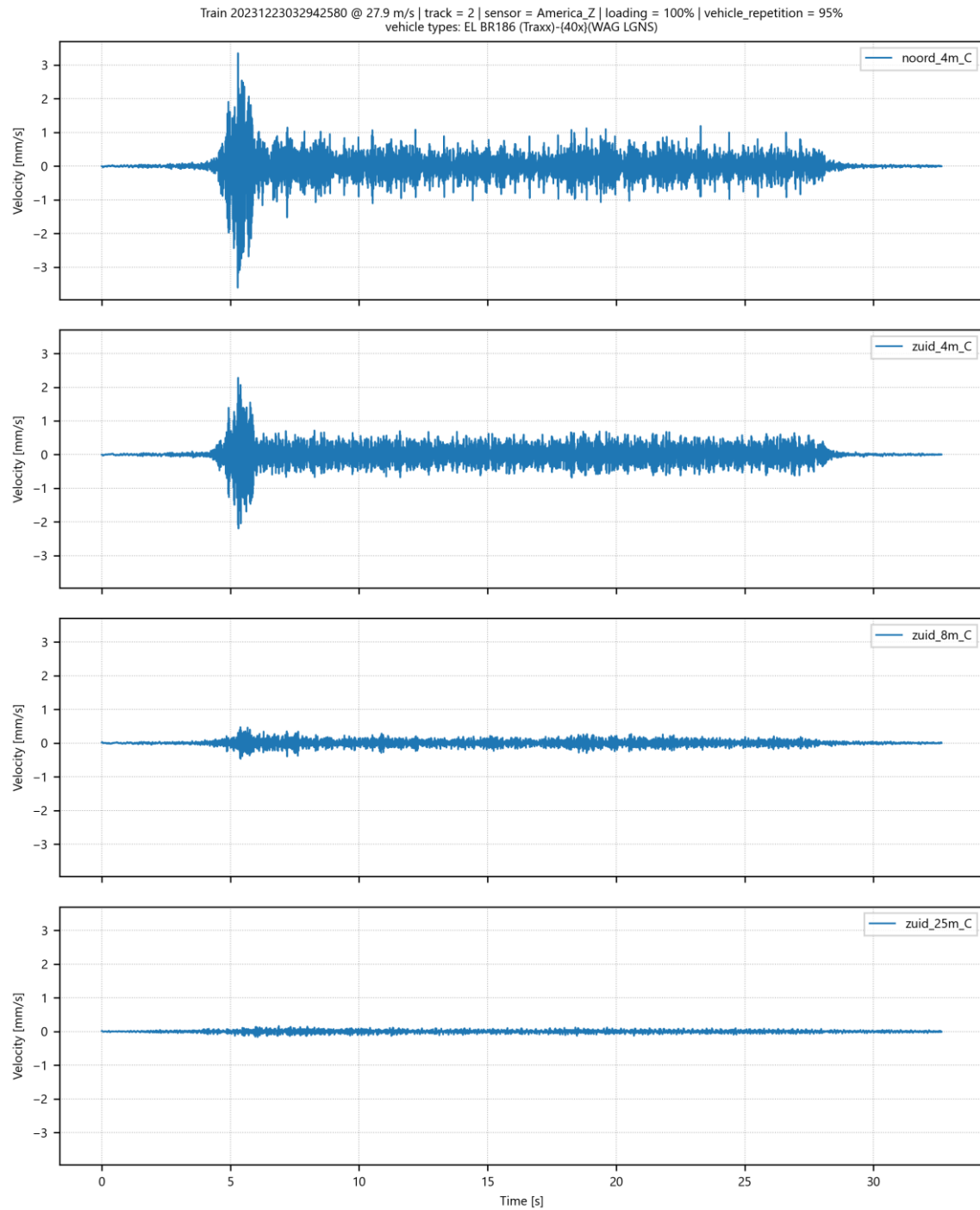
Afbeelding II.40 Trillingsnelheid in Z-richting op 4 meetpunten in America voor goederentrein passage op spoor 2 op 23-12-2023
