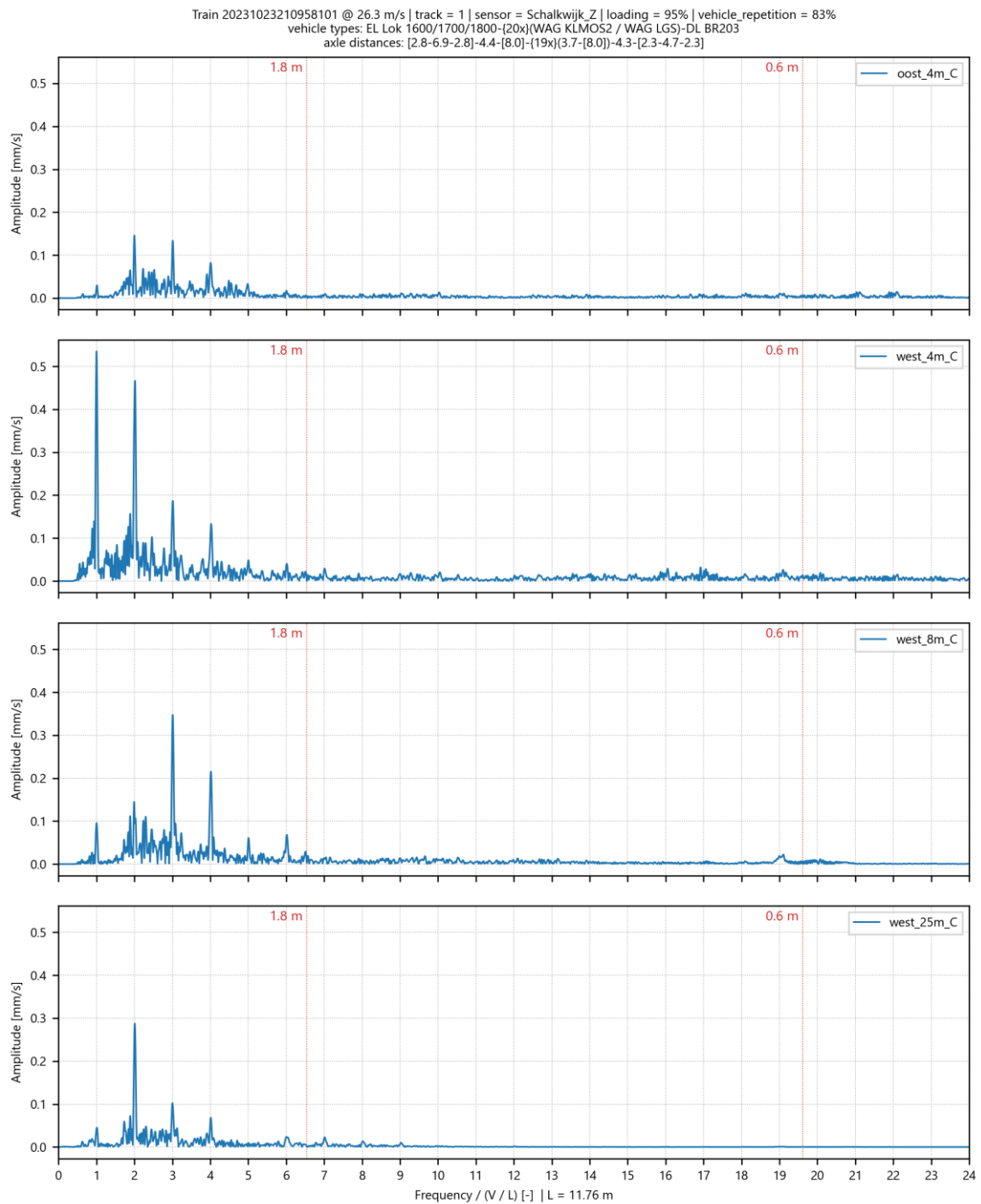
Afbeelding I.6 Genormaliseerd amplitude spectrum voor trillingssnelheid in Z-richting op 4 meetpunten in Schalkwijk voor goederentrein passage op spoor 1 op 23-10-2023
