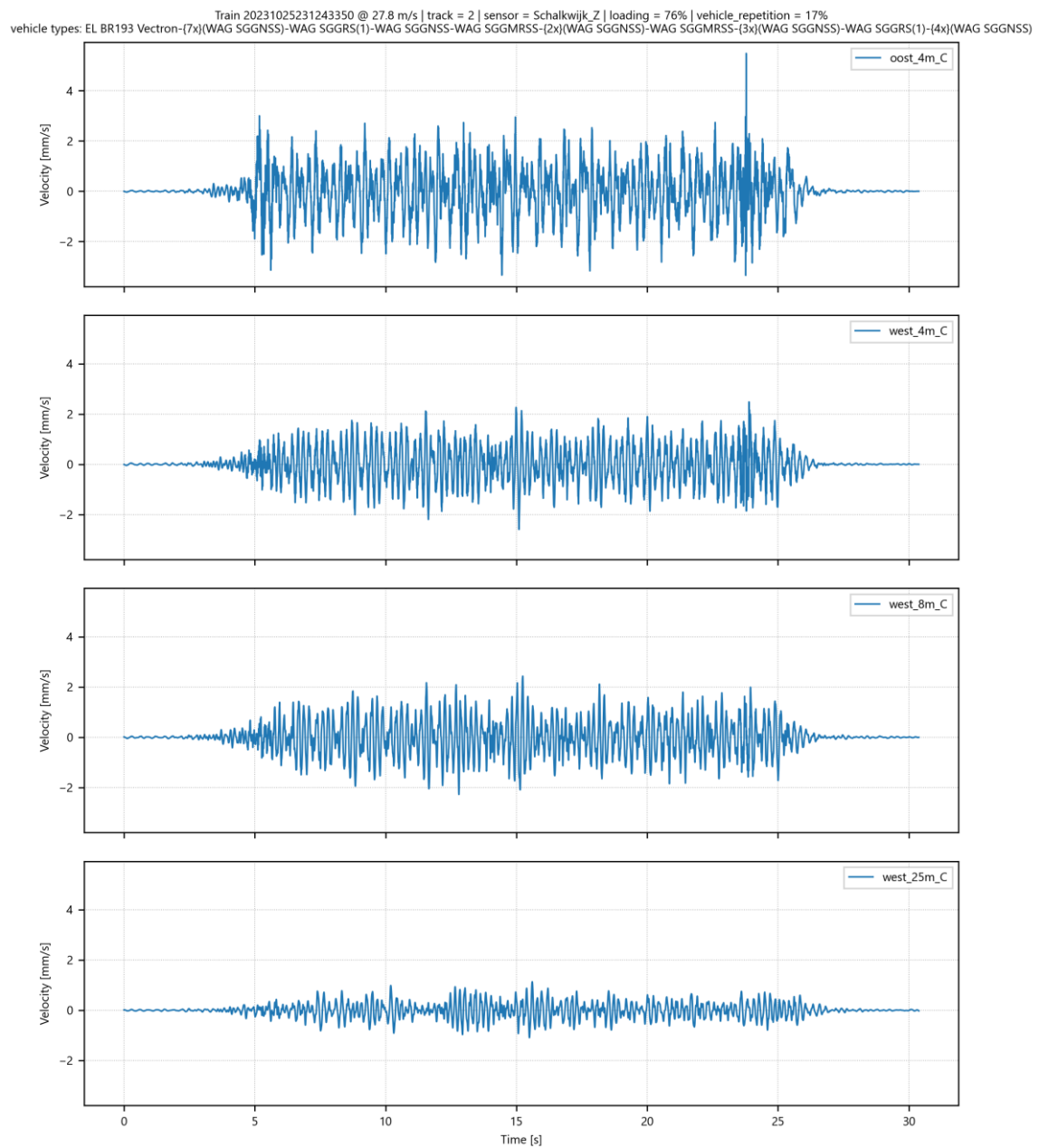
Afbeelding I.31 Trillingssnelheid in Z-richting op 4 meetpunten in Schalkwijk voor goederentrein passage op spoor 2 op 25-10-2023
