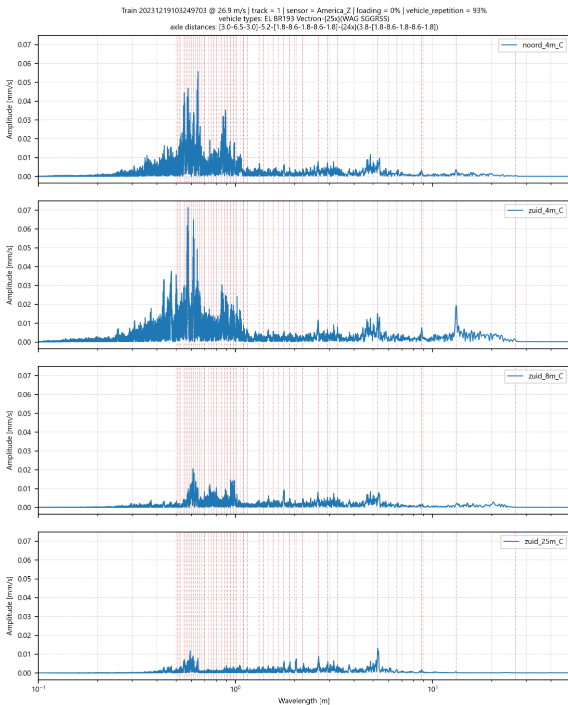
Afbeelding II.35 Amplitude spectrum voor trillingsnelheid in Z-richting op 4 meetpunten in America voor goederentrein passage op spoor 1 op 19-12-2023
