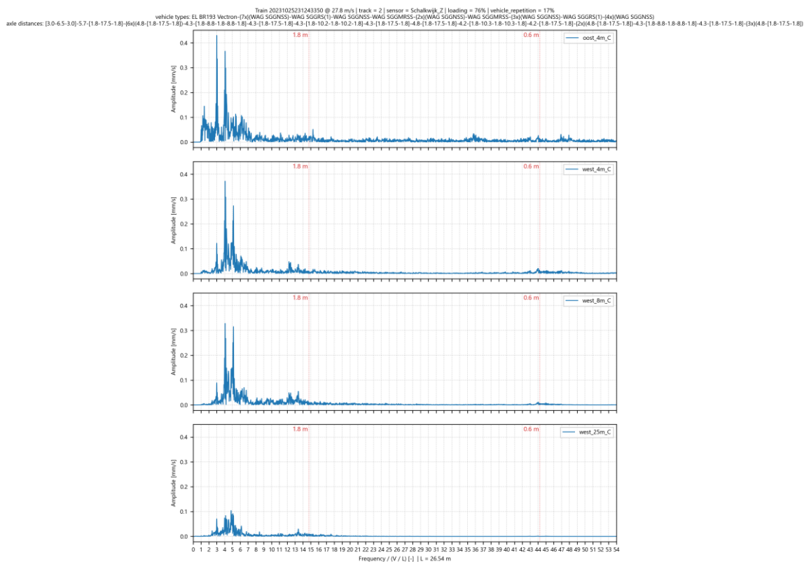
Afbeelding I.33 Genormaliseerd amplitude spectrum voor trillingssnelheid in Z-richting op 4 meetpunten in Schalkwijk voor goederentrein passage op spoor 2 op 25-10-2023
