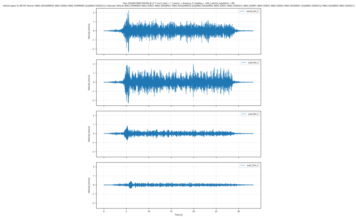
Afbeelding II.7 Trillingssnelheid in Z-richting op 4 meetpunten in America voor goederentrein passage op spoor 1 op 19-04-2024
