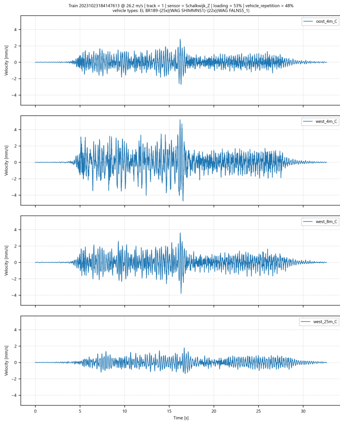
Afbeelding I.22 Trillingssnelheid in Z-richting op 4 meetpunten in Schalkwijk voor goederentrein passage op spoor 1 op 23-10-2023
