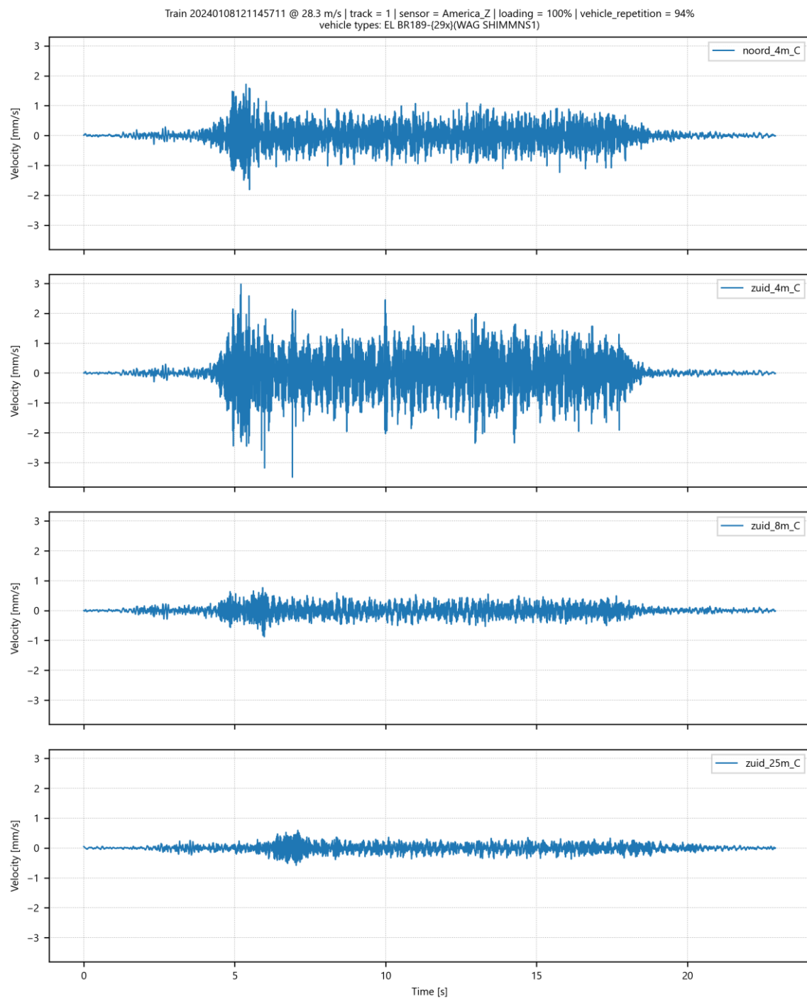
Afbeelding II.28 Trillingssnelheid in Z-richting op 4 meetpunten in America voor goederentrein passage op spoor 1 op 08-01-2024
