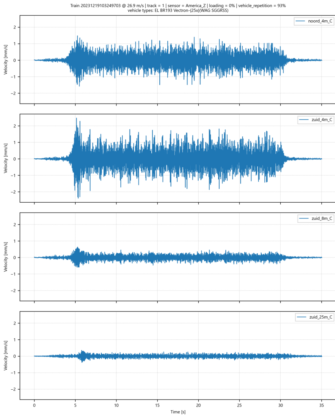
Afbeelding II.34 Trillingssnelheid in Z-richting op 4 meetpunten in America voor goederentrein passage op spoor 1 op 19-12-2023
