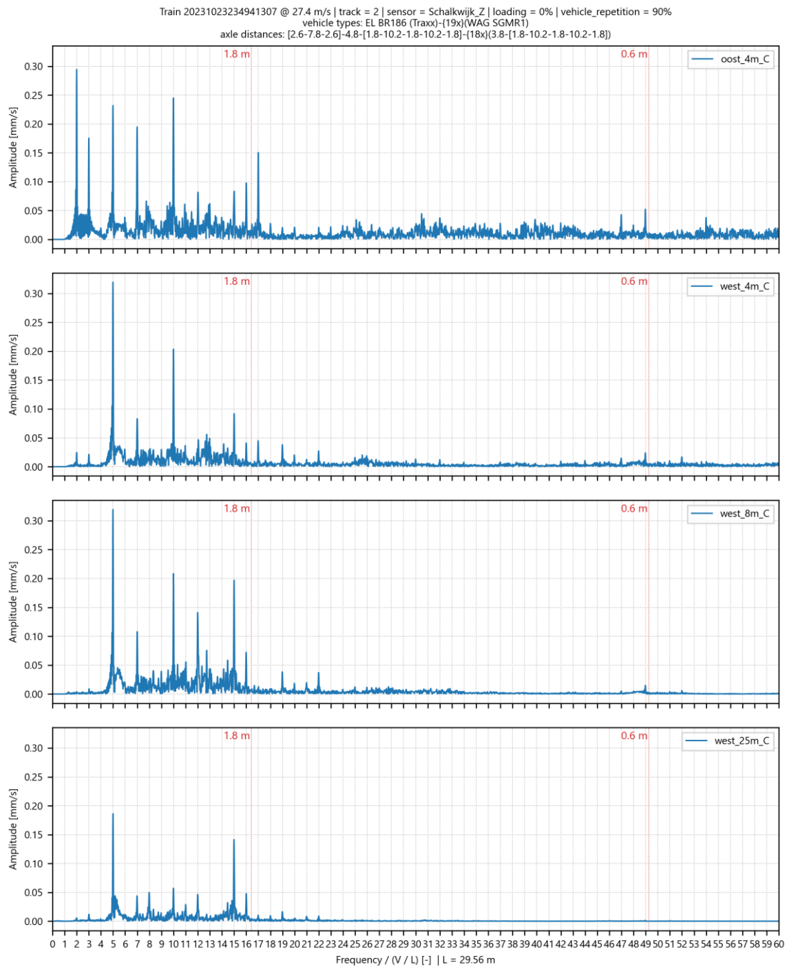
Afbeelding I.45 Genormaliseerd amplitude spectrum voor trillingssnelheid in Z-richting op 4 meetpunten in Schalkwijk voor goederentrein passage op spoor 2 op 23-10-2023
