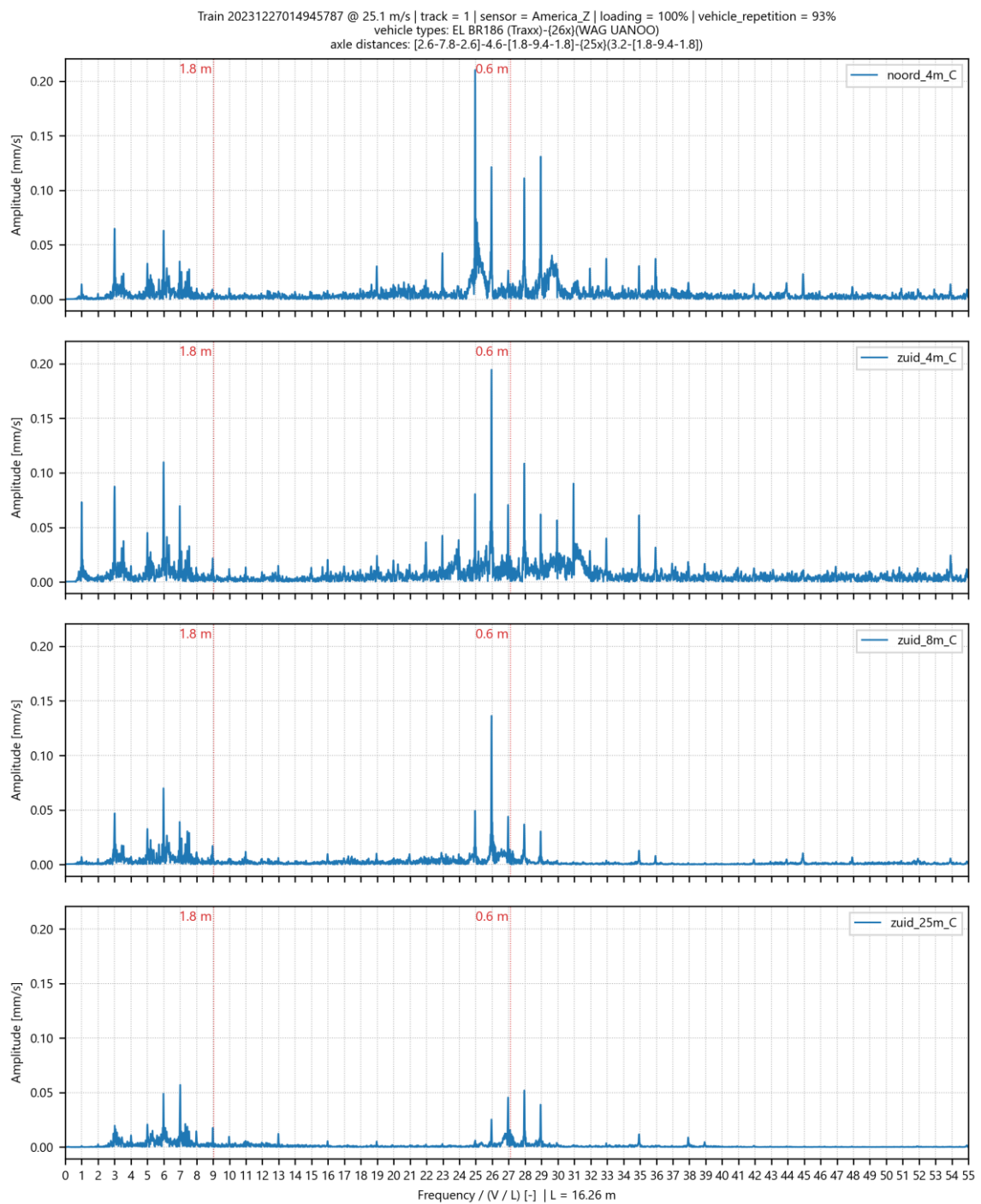
Afbeelding II.33 Genormaliseerd amplitude spectrum voor trillingssnelheid in Z-richting op 4 meetpunten in America voor goederentrein passage op spoor 1 op 27-12-2023
