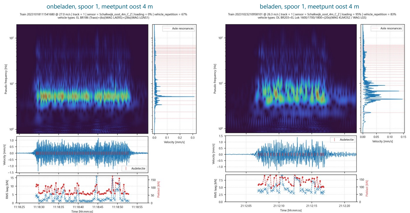
Afbeelding 4.1 Tijd-frequentie plots voor trillingssnelheid in Z-richting op 5 meetpunten in Schalkwijk (onder elkaar) voor twee goederentrein passages, links op spoor 1 met onbeladen WAG LGNS wagons op 18-10-2023 en rechts op spoor 2 met beladen WAG KLMOS2 / WAG LGS wagons op 23-10-2023
