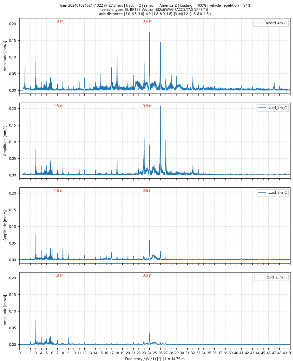
Afbeelding II.54 Genormaliseerd amplitude spectrum voor trillingssnelheid in Z-richting op 4 meetpunten in America voor goederentrein passage op spoor 2 op 02-01-2024
