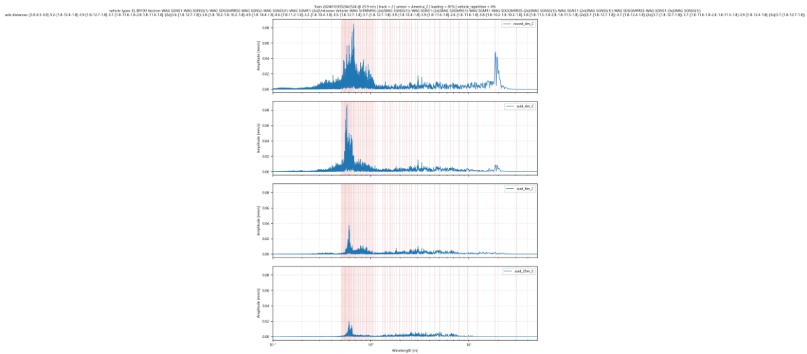
Afbeelding II.47 Amplitude spectrum voor trillingssnelheid in Z-richting op 4 meetpunten in America voor goederentrein passage op spoor 2 op 03-01-2024
