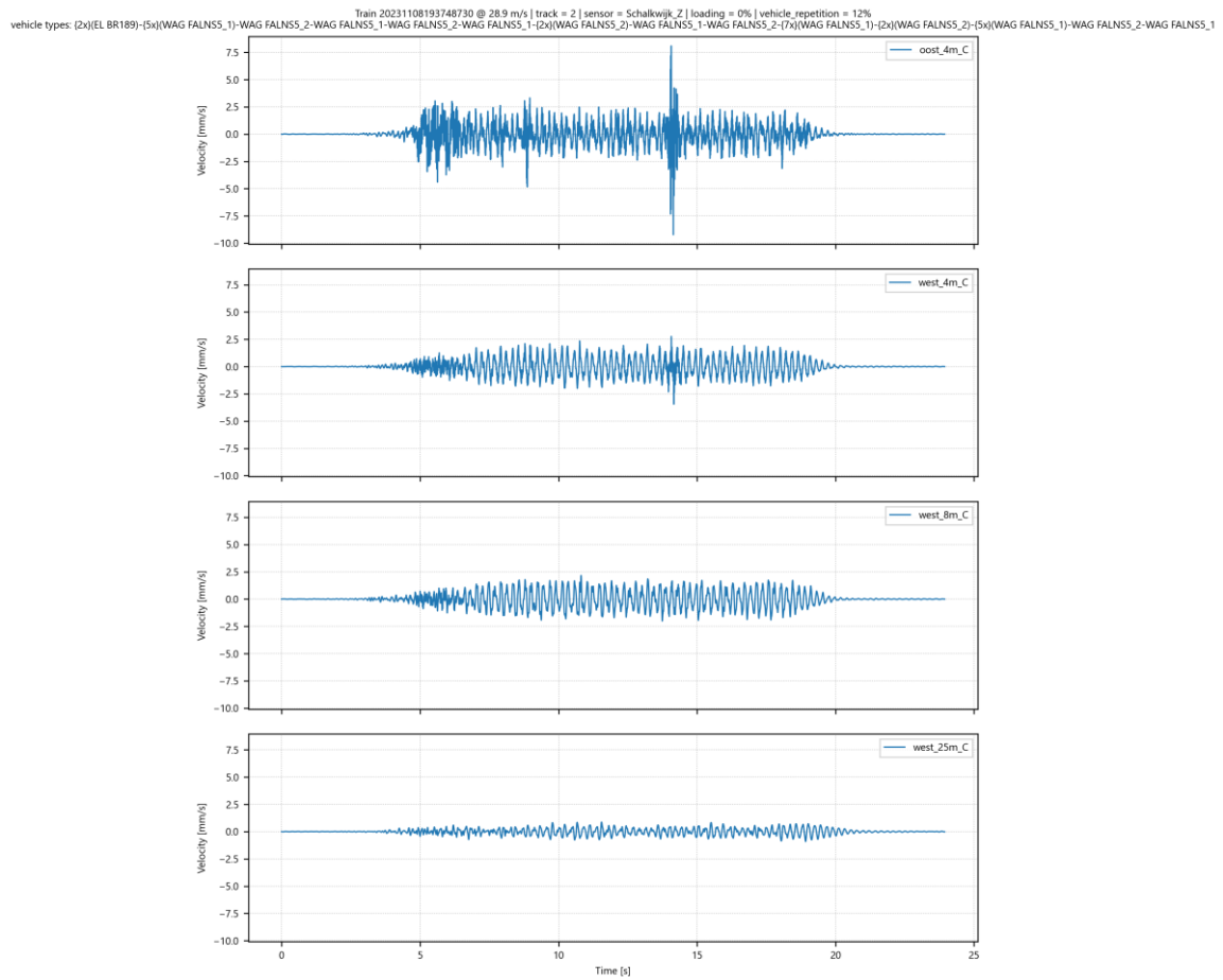
Afbeelding I.28 Trillingssnelheid in Z-richting op 4 meetpunten in Schalkwijk voor goederentrein passage op spoor 2 op 08-11-2023
