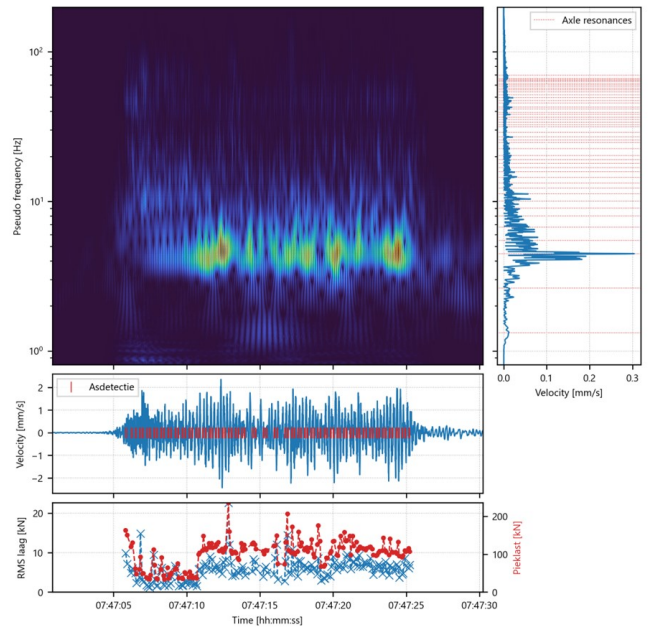
beladen, spoor 1, meetpunt oost 4 m
