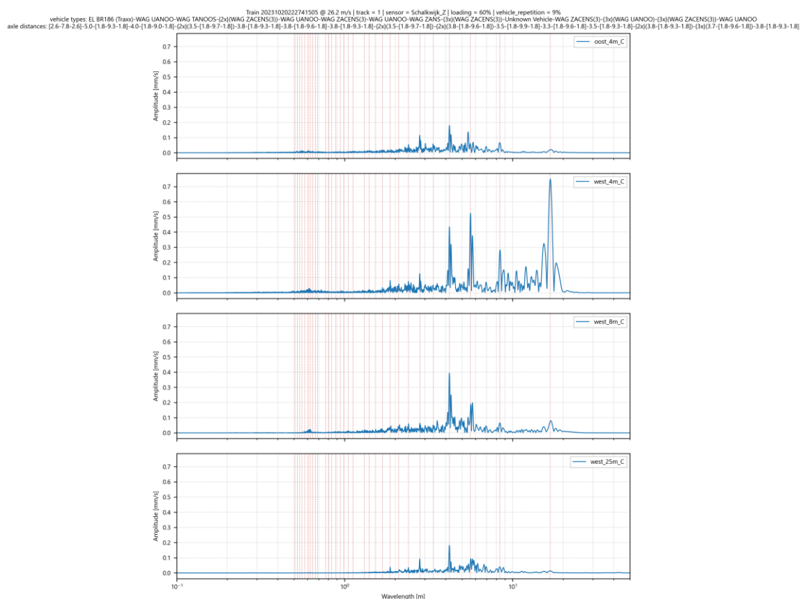
Afbeelding I.14 Amplitude spectrum voor trillingsnelheid in Z-richting op 4 meetpunten in Schalkwijk voor goederentrein passage op spoor 1 op 20-10-2023
