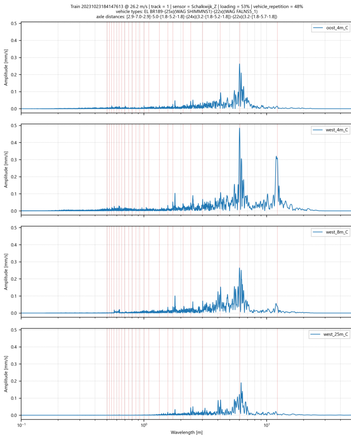
Afbeelding I.23 Amplitude spectrum voor trillingssnelheid in Z-richting op 4 meetpunten in Schalkwijk voor goederentrein passage op spoor 1 op 23-10-2023
