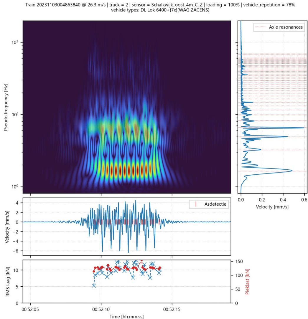
Abbeelding 3.4 Voorbeeld weergave trillingssignaal in tijds- en frequentiedomein inclusief Quo Vadis parameters
