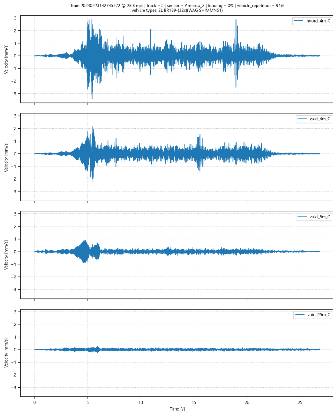
Afbeelding II.49 Trillingssnelheid in Z-richting op 4 meetpunten in America voor goederentrein passage op spoor 2 op 23-02-2024
