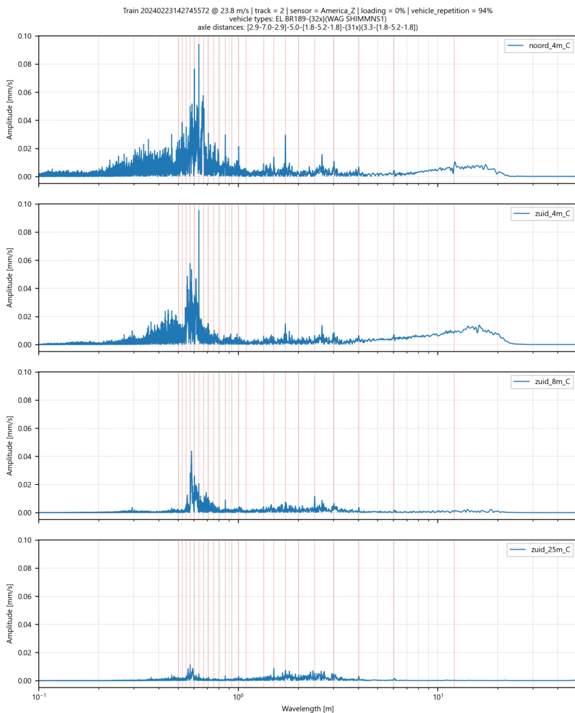
Afbeelding II.50 Amplitude spectrum voor trillingssnelheid in Z-richting op 4 meetpunten in America voor goederentrein passage op spoor 2 op 23-02-2024
