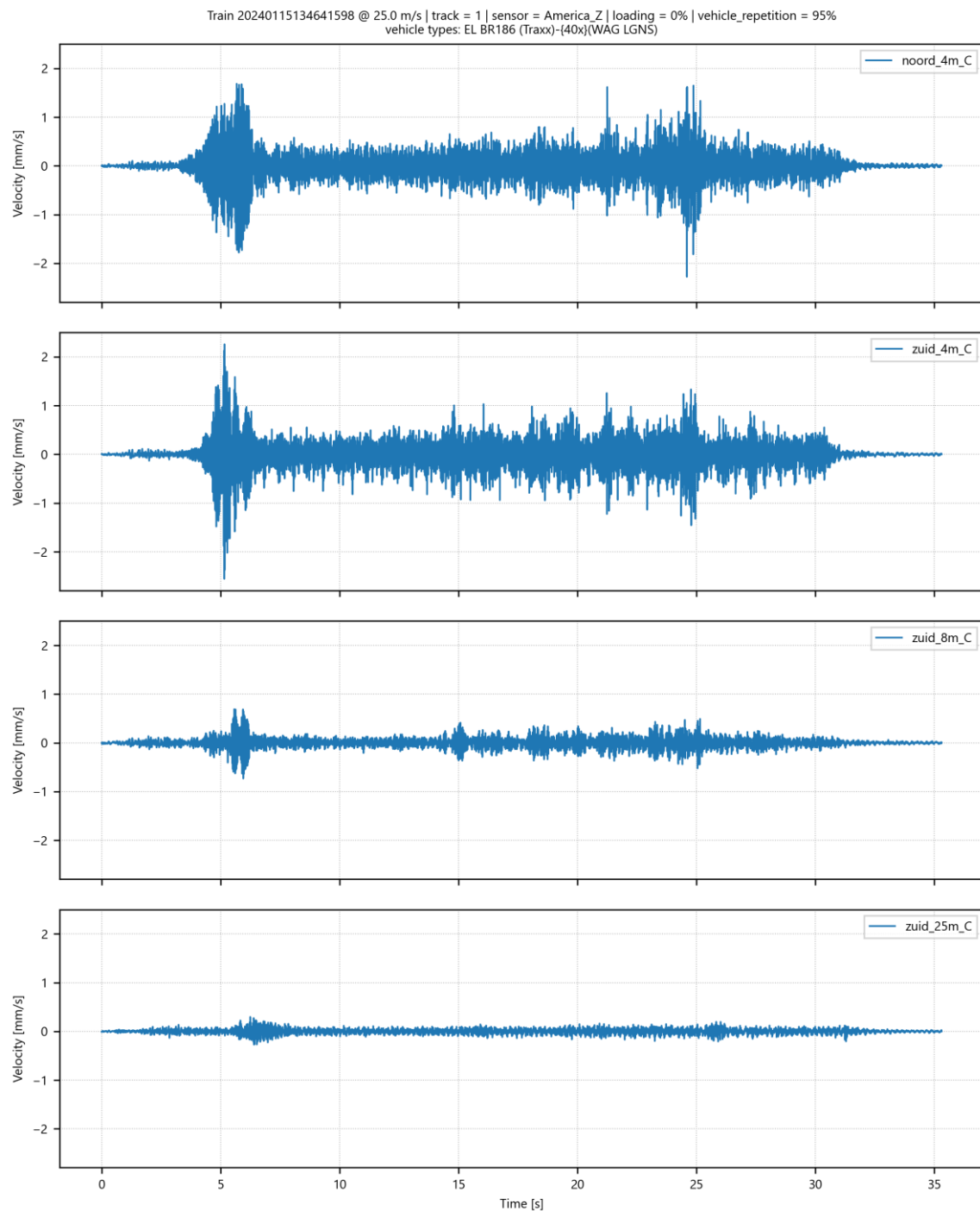
Afbeelding II.1 Trillingssnelheid in Z-richting op 4 meetpunten in America voor goederentrein passage op spoor 1 op 15-01-2024
