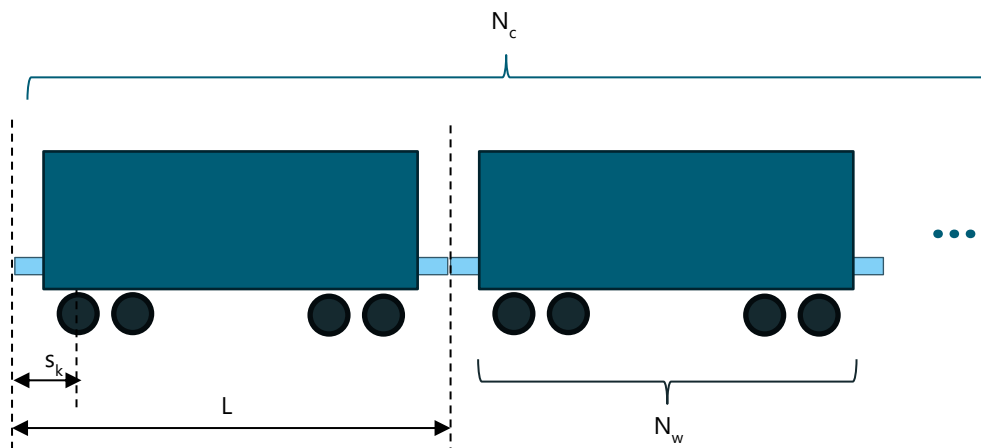
Afbeelding 3.1 Schematisatie aslasten van een reeks wagons
