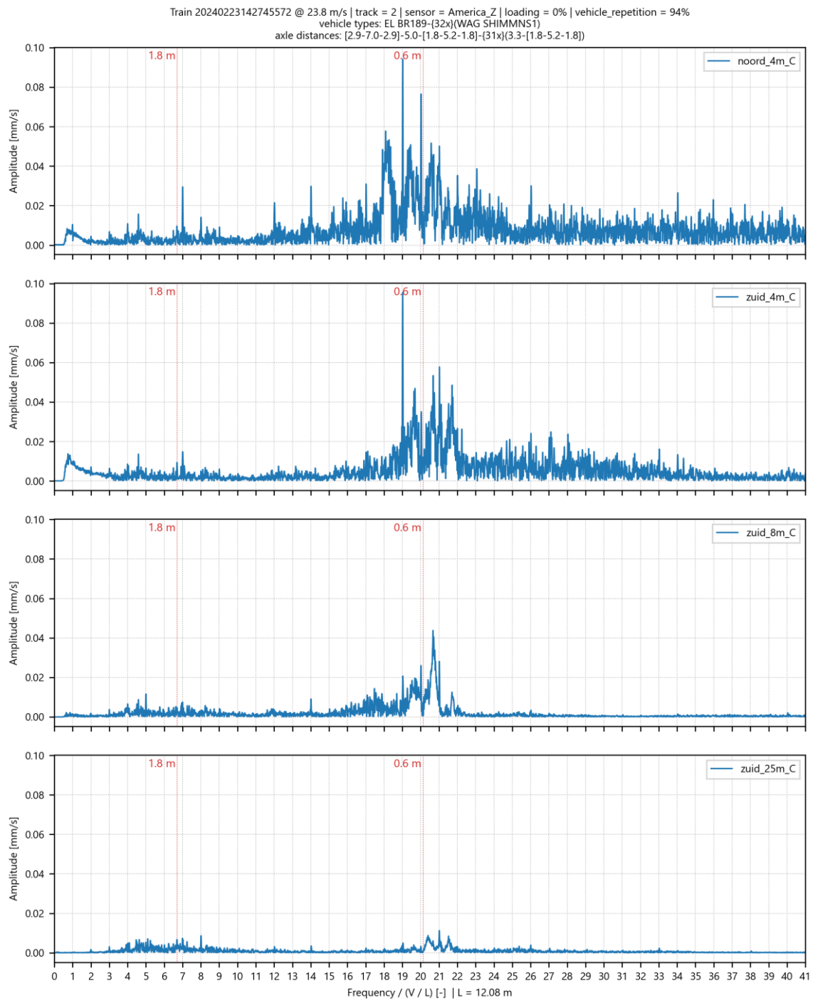
Afbeelding II.51 Genormaliseerd amplitude spectrum voor trillingssnelheid in Z-richting op 4 meetpunten in America voor goederentrein passage op spoor 2 op 23-02-2024
