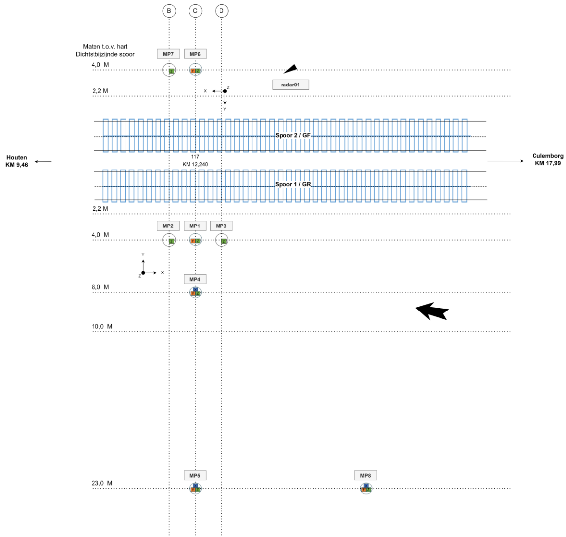
Afbeelding 2.1 Schematische weergave meetopstelling locatie Schalkwijk
