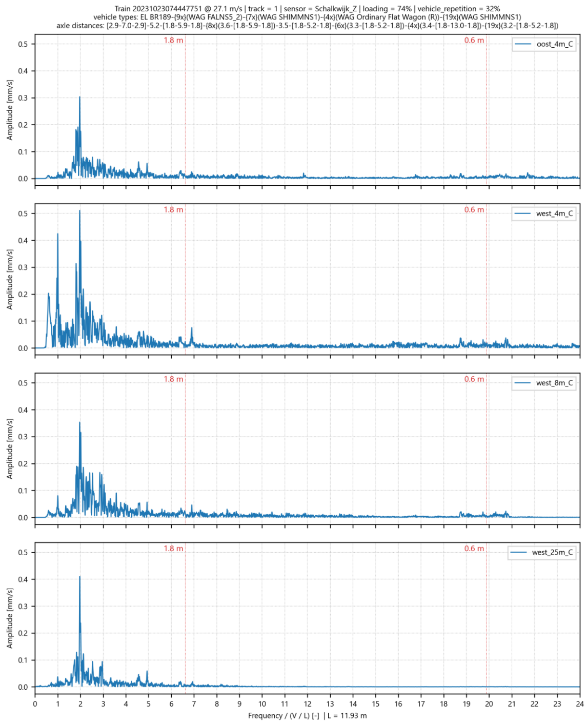
Afbeelding I.21 Genormaliseerd amplitude spectrum voor trillingssnelheid in Z-richting op 4 meetpunten in Schalkwijk voor goederentrein passage op spoor 1 op 23-10-2023
