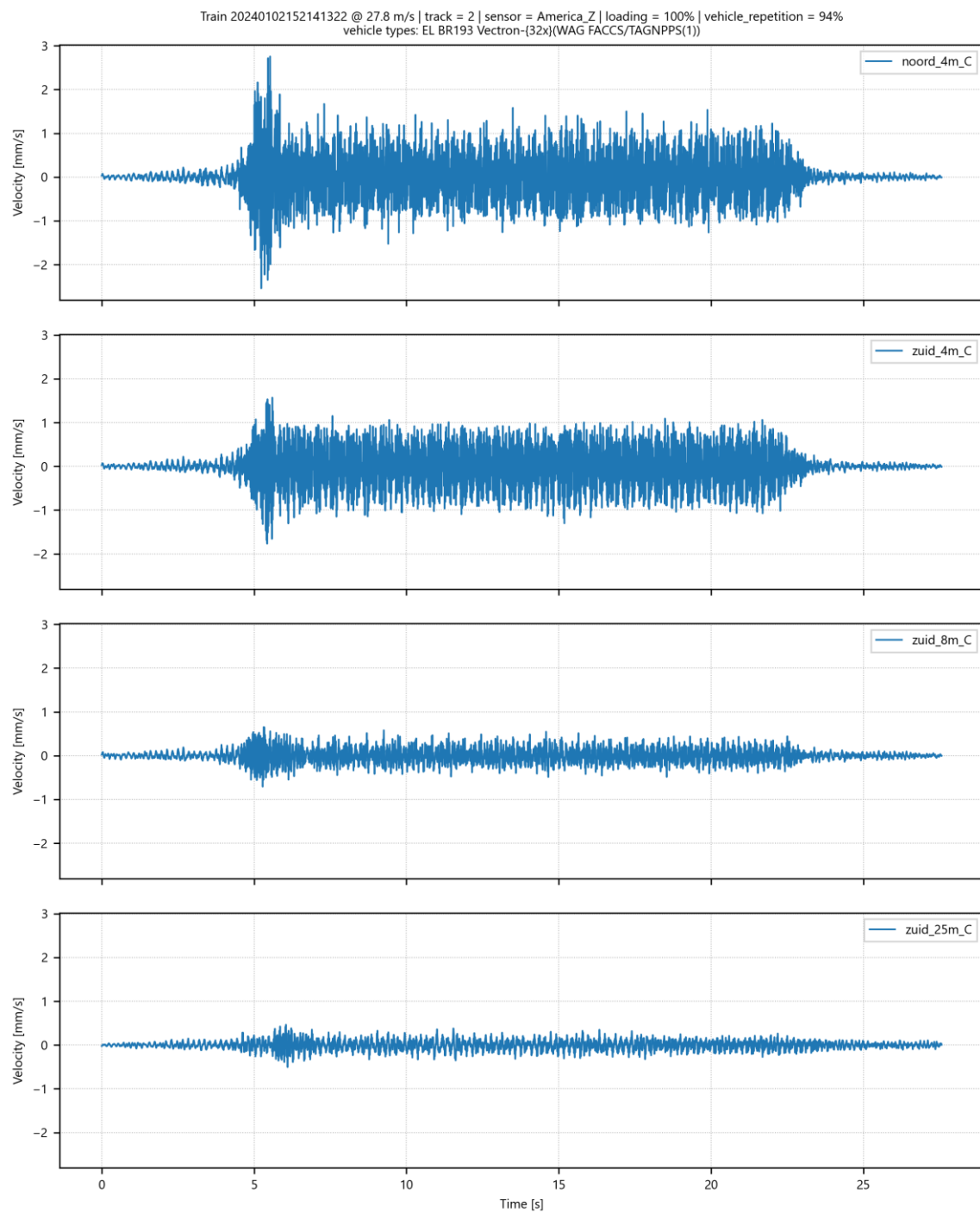
Afbeelding II.52 Trillingssnelheid in Z-richting op 4 meetpunten in America voor goederentrein passage op spoor 2 op 02-01-2024
