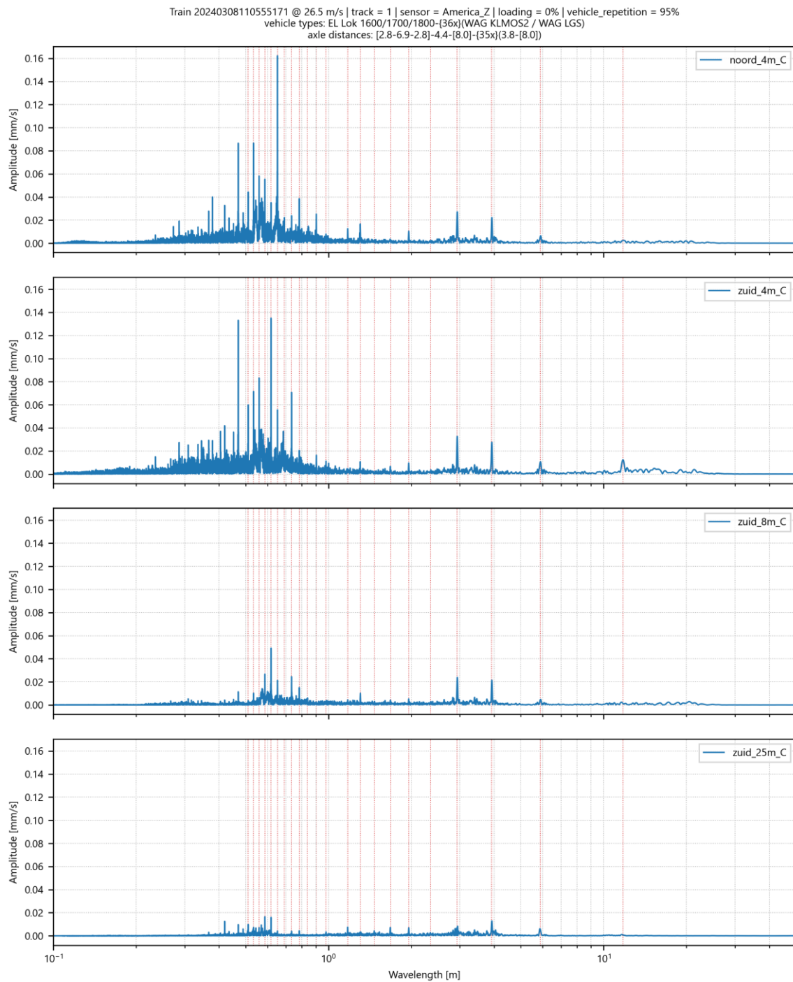
Afbeelding II.5 Amplitude spectrum voor trillingssnelheid in Z-richting op 4 meetpunten in America voor goederentrein passage op spoor 1 op 08-03-2024
