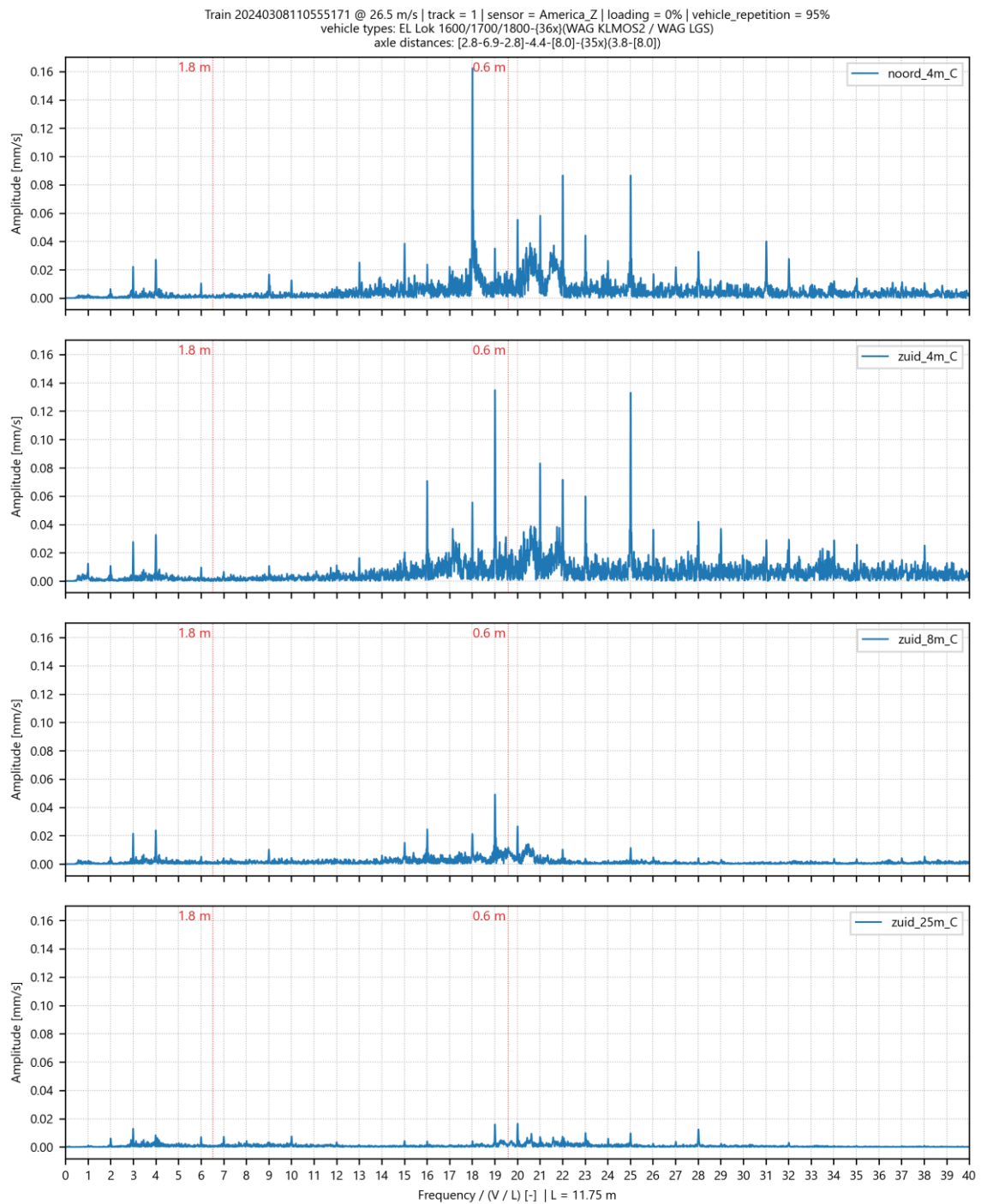
Afbeelding II.6 Genormaliseerd amplitude spectrum voor trillingssnelheid in Z-richting op 4 meetpunten in America voor goederentrein passage op spoor 1 op 08-03-2024
