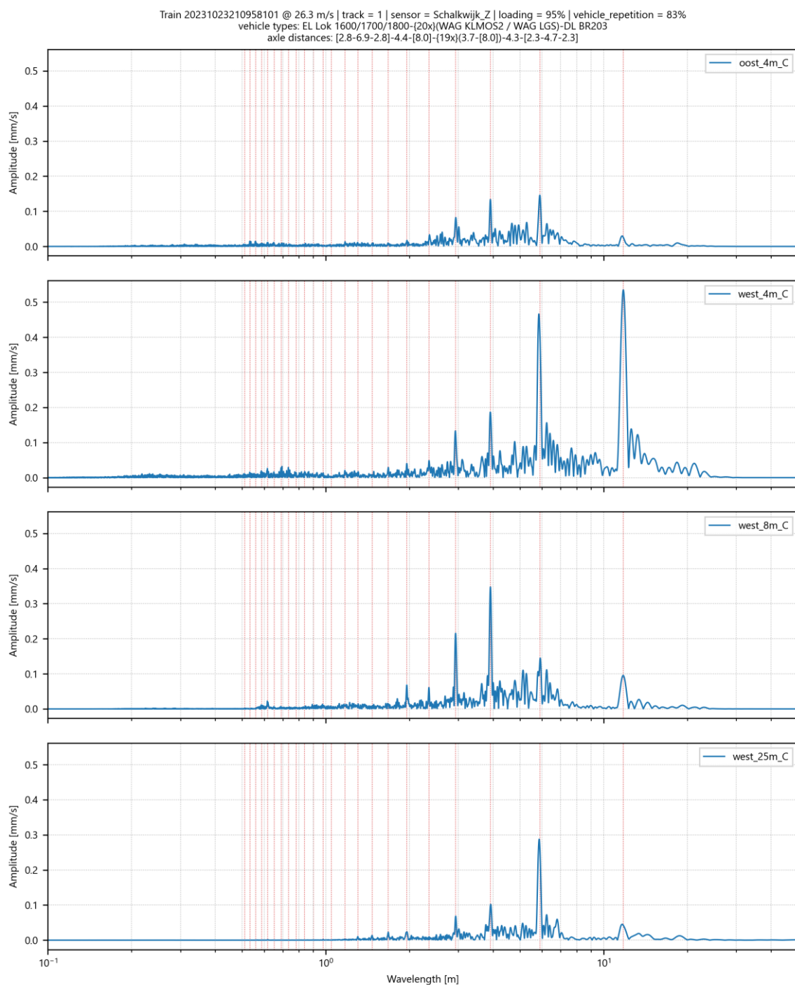
Afbeelding I.5 Amplitude spectrum voor trillingssnelheid in Z-richting op 4 meetpunten in Schalkwijk voor goederentrein passage op spoor 1 op 23-10-2023
