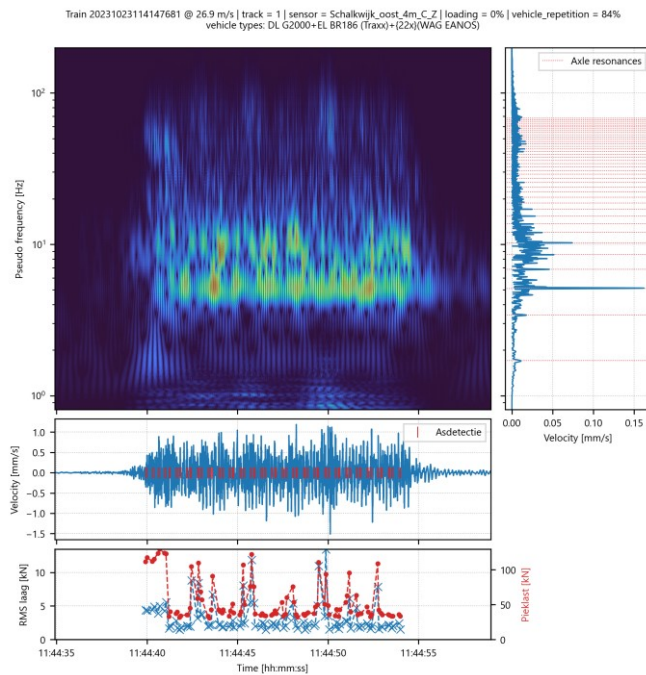
onbeladen, spoor 1, meetpunt oost 4 m
