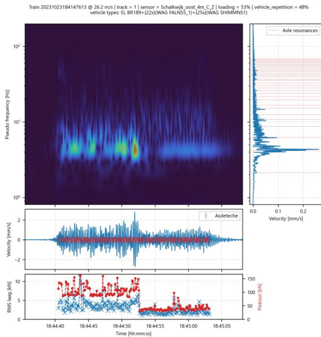
Afbeelding 4.4 Tijd-frequentie plots voor trillingssnelheid in Z-richting op 5 meetpunten in Schalkwijk (onder elkaar) voor twee goederentrein passages met WAG FALNS5_1 en WAG SHIMMNS1 wagons, links op spoor 1 met 53/47 % beladen /onbeladen wagons op 23-10-2023 en rechts op spoor 2 met 46/54 % onbeladen/beladen wagons op 19-10-2023
