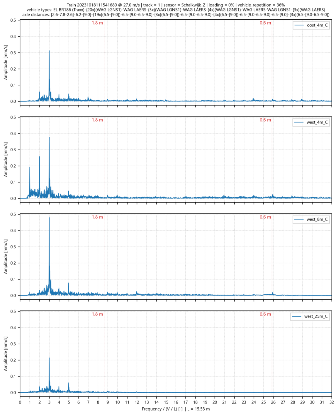
Afbeelding I.3 Genormaliseerd amplitude spectrum voor trillingssnelheid in Z-richting op 4 meetpunten in Schalkwijk voor goederentrein passage op spoor 1 op 18-10-2023
