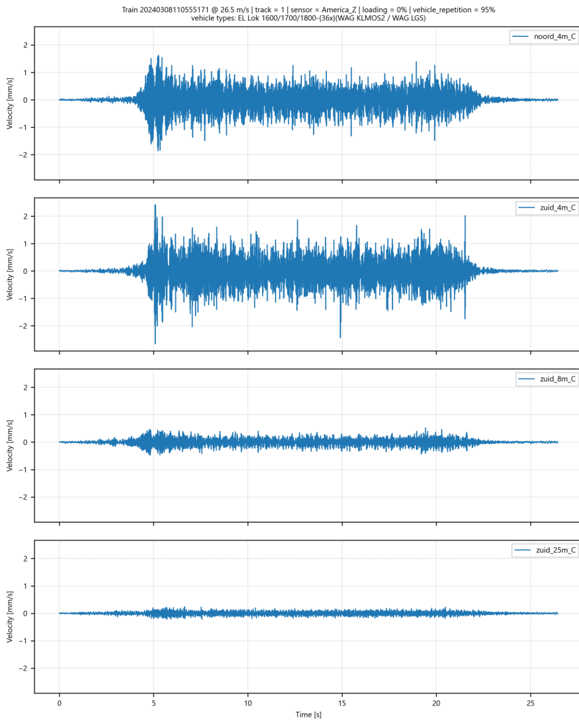
Afbeelding II.4 Trillingssnelheid in Z-richting op 4 meetpunten in America voor goederentrein passage op spoor 1 op 08-03-2024
