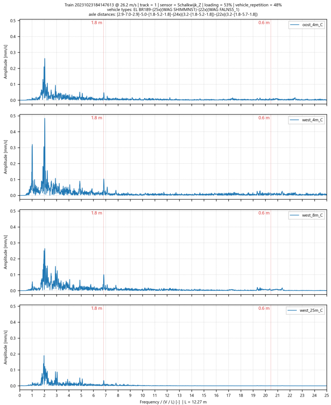
Afbeelding I.24 Genormaliseerd amplitude spectrum voor trillingssnelheid in Z-richting op 4 meetpunten in Schalkwijk voor goederentrein passage op spoor 1 op 23-10-2023
