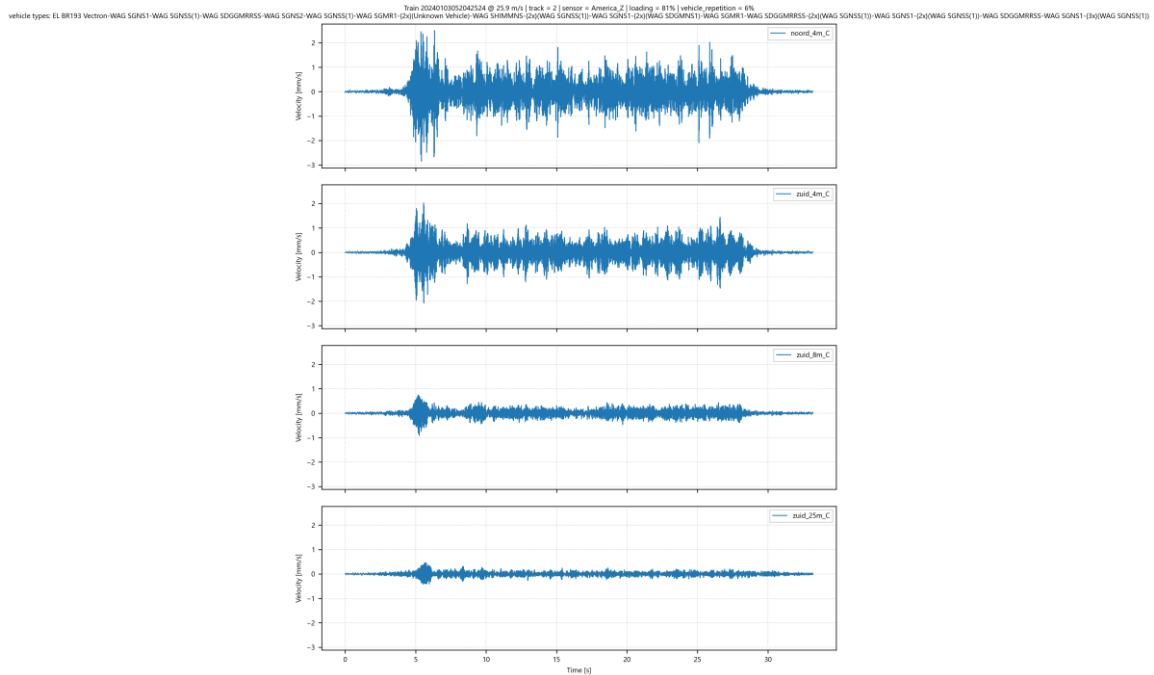
Afbeelding II.46 Trillingssnelheid in Z-richting op 4 meetpunten in America voor goederentrein passage op spoor 2 op 03-01-2024
