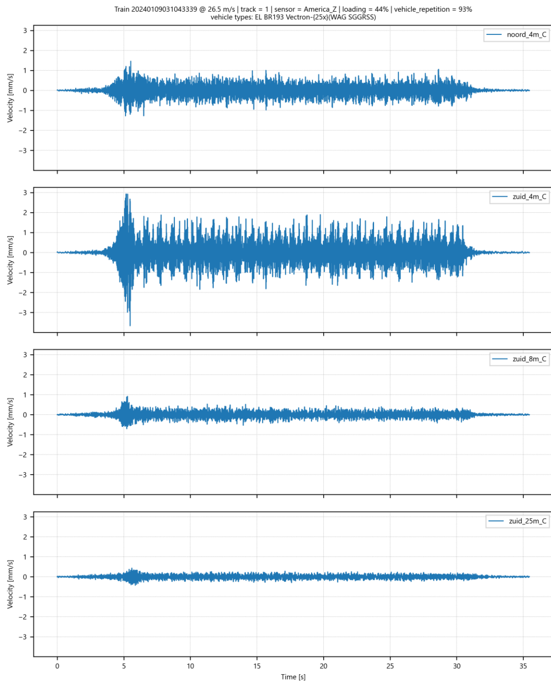
Afbeelding II.37 Trillingssnelheid in Z-richting op 4 meetpunten in America voor goederentrein passage op spoor 1 op 09-01-2024
