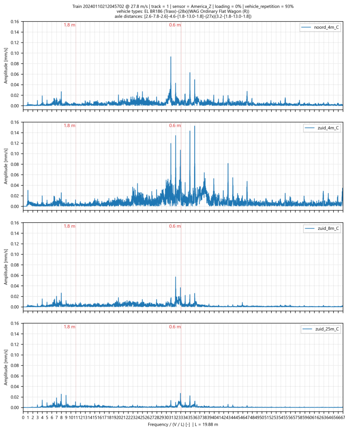
Afbeelding II.27 Genormaliseerd amplitude spectrum voor trillingssnelheid in Z-richting op 4 meetpunten in America voor goederentrein passage op spoor 1 op 10-01-2024
