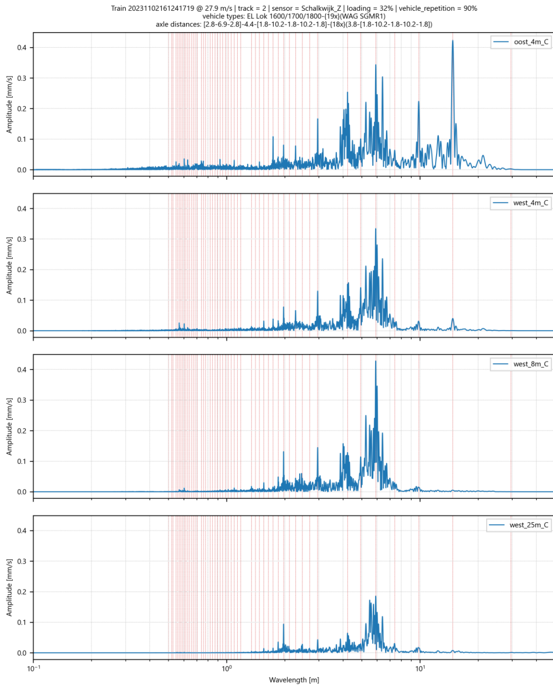
Afbeelding I.47 Amplitude spectrum voor trillingssnelheid in Z-richting op 4 meetpunten in Schalkwijk voor goederentrein passage op spoor 2 op 02-11-2023
