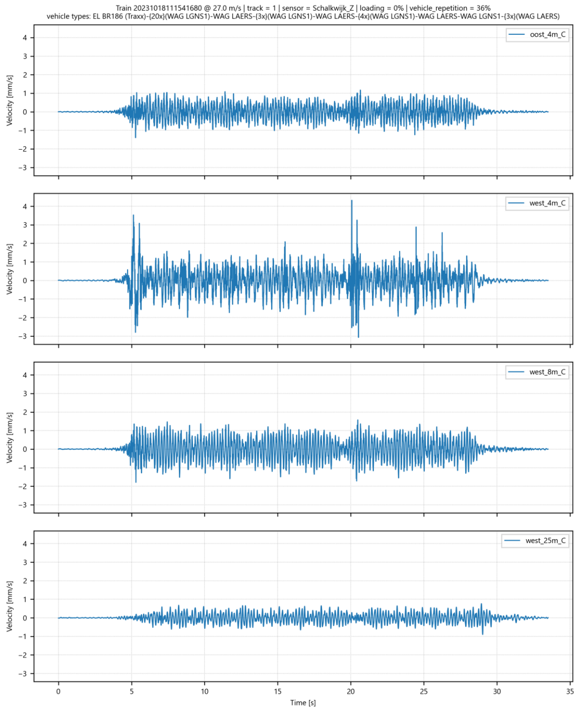
Afbeelding I.1 Trillingssnelheid in Z-richting op 4 meetpunten in Schalkwijk voor goederentrein passage op spoor 1 op 18-10-2023
