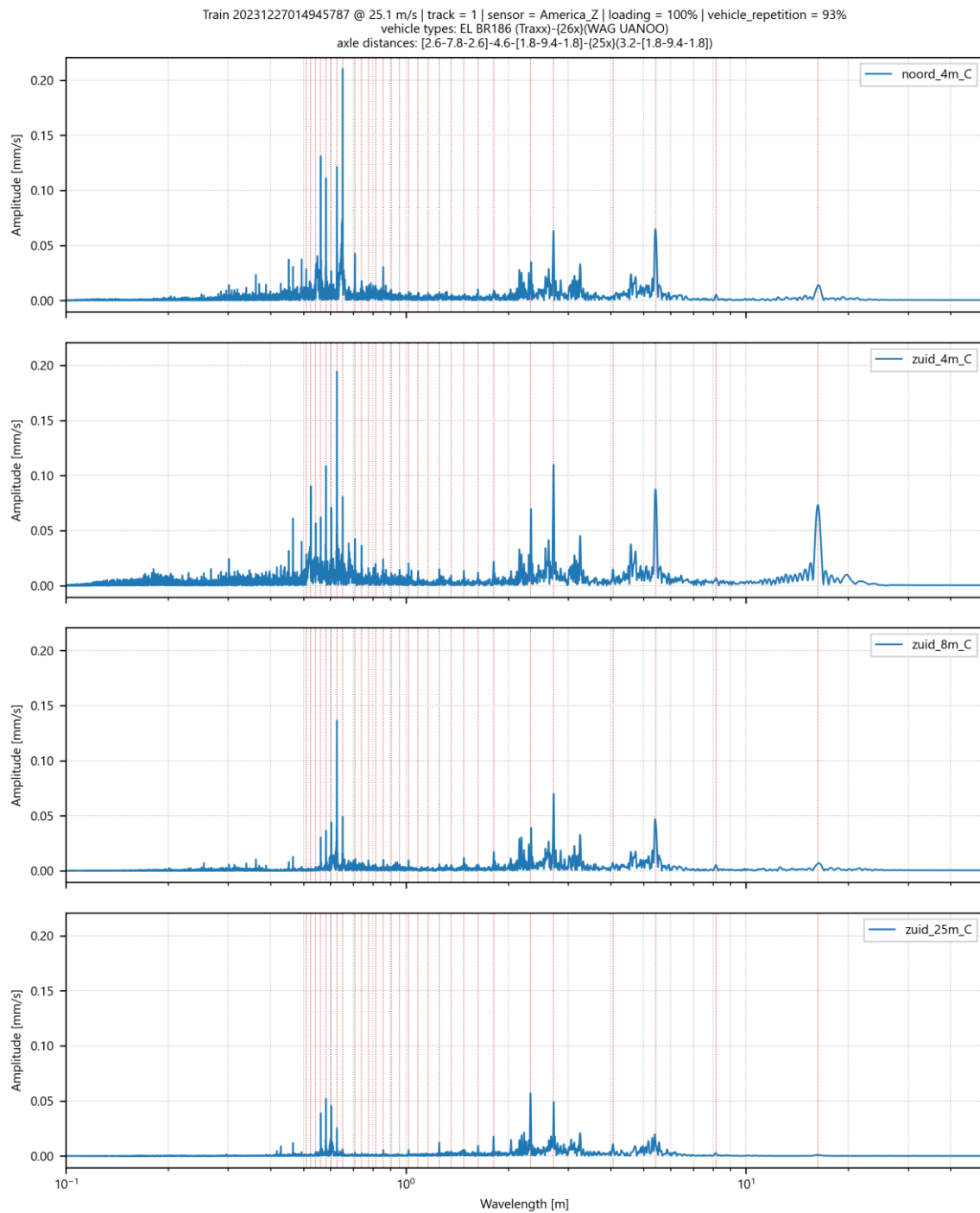
Afbeelding II.32 Amplitude spectrum voor trillingssnelheid in Z-richting op 4 meetpunten in America voor goederentrein passage op spoor 1 op 27-12-2023
