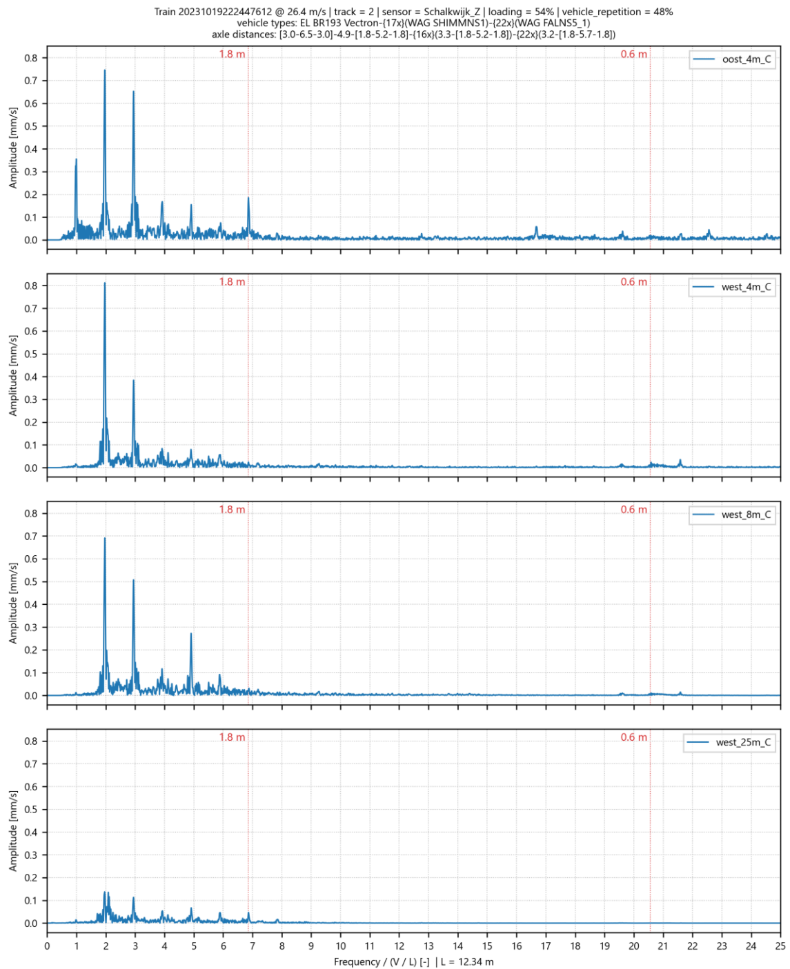
Afbeelding I.36 Genormaliseerd amplitude spectrum voor trillingssnelheid in Z-richting op 4 meetpunten in Schalkwijk voor goederentrein passage op spoor 2 op 19-10-2023
