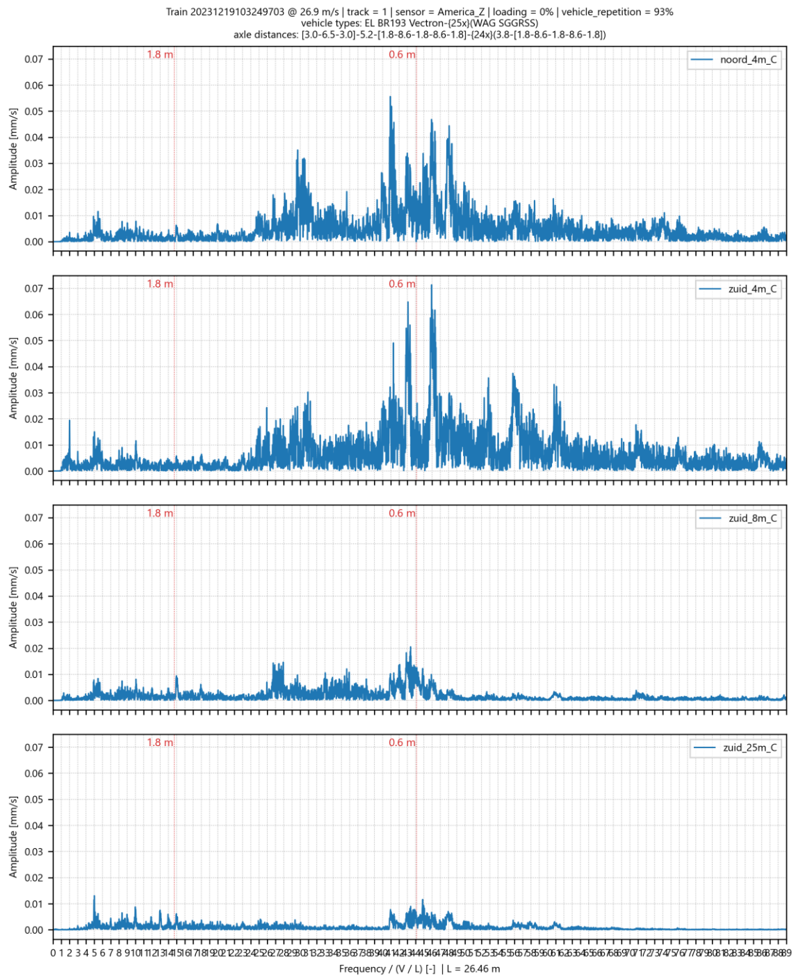
Afbeelding II.36 Genormaliseerd amplitude spectrum voor trillingssnelheid in Z-richting op 4 meetpunten in America voor goederentrein passage op spoor 1 op 19-12-2023
