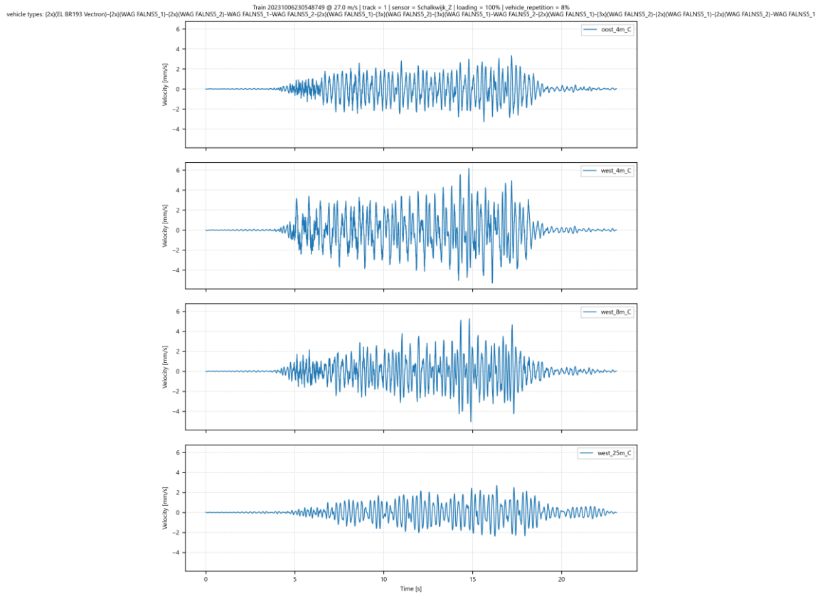
Afbeelding I.16 Trillingssnelheid in Z-richting op 4 meetpunten in Schalkwijk voor goederentrein passage op spoor 1 op 06-10-2023
