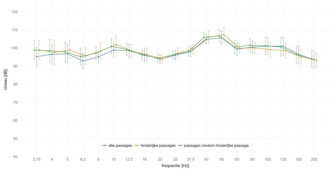
locatie Holten : gemiddeld spectrum passage met GO op spoor 1 meetlocatie: noord 4m C | meetrichting: Z | voetbalk met +/- standaard afwijking
