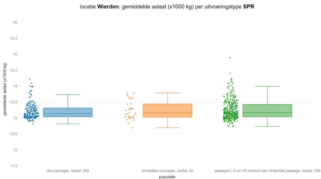
figuur 144 Gemiddelde aslast voor sprinters per populatie
