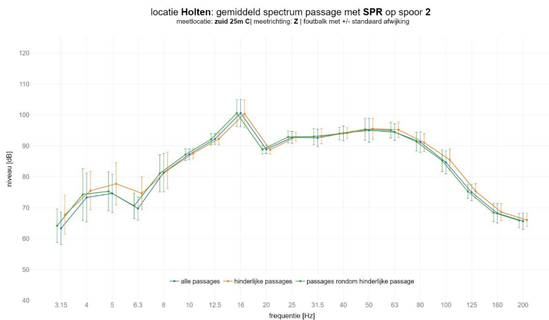
figuur 86 Gemiddeld spectrum 25m zuid, Z richting voor sprinters
