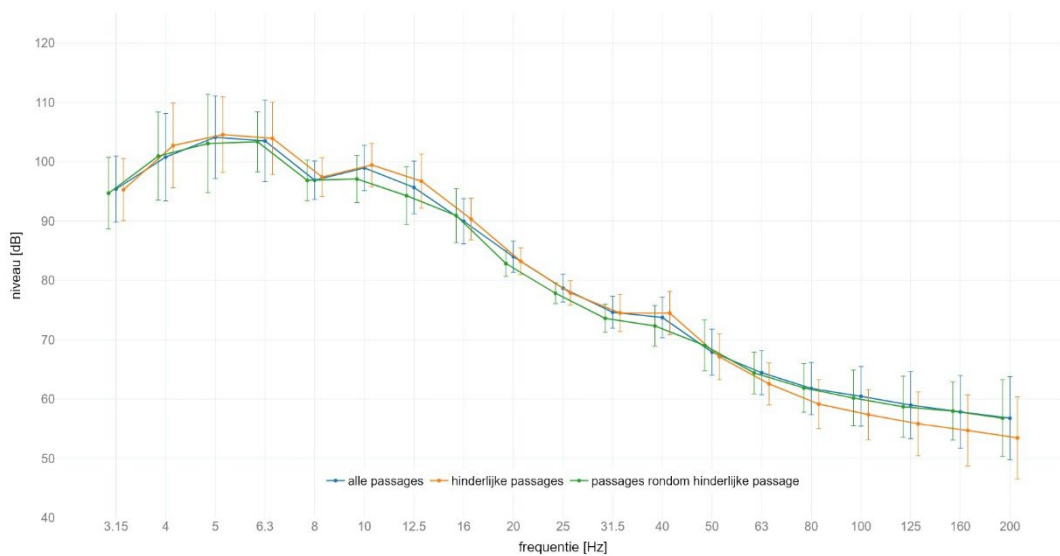
locatie Schalkwijk : gemiddeld spectrum passage met GO op spoor 1 meetlocatie: west 25m C | meetrichting: Y | voetbalk met +/- standaard afwijking
