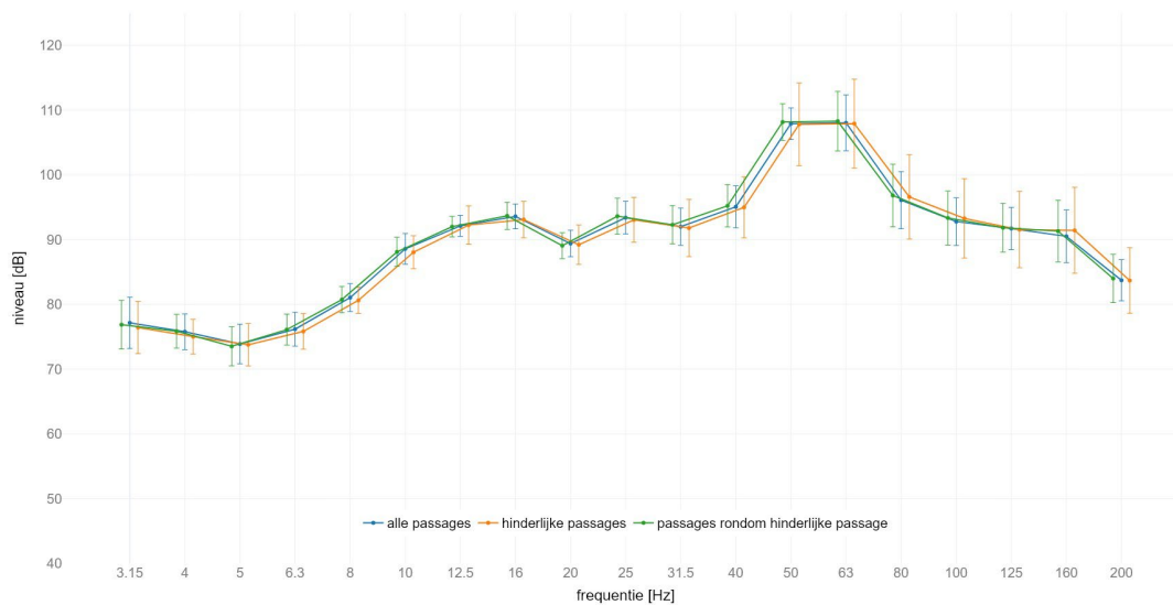
locatie Holten : gemiddeld spectrum passage met SPR op spoor 1 meetlocatie: zuid 8m C | meetrichting: X | voetbalk met +/- standaard afwijking
