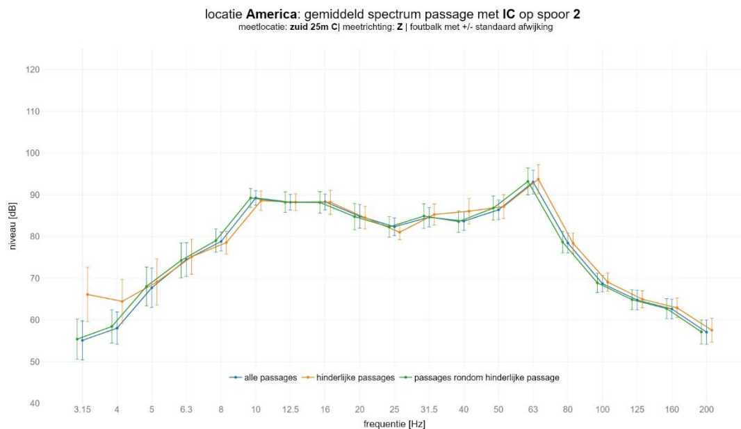
figuur 56 Gemiddeld spectrum 25m zuid, Z richting voor intercity's
