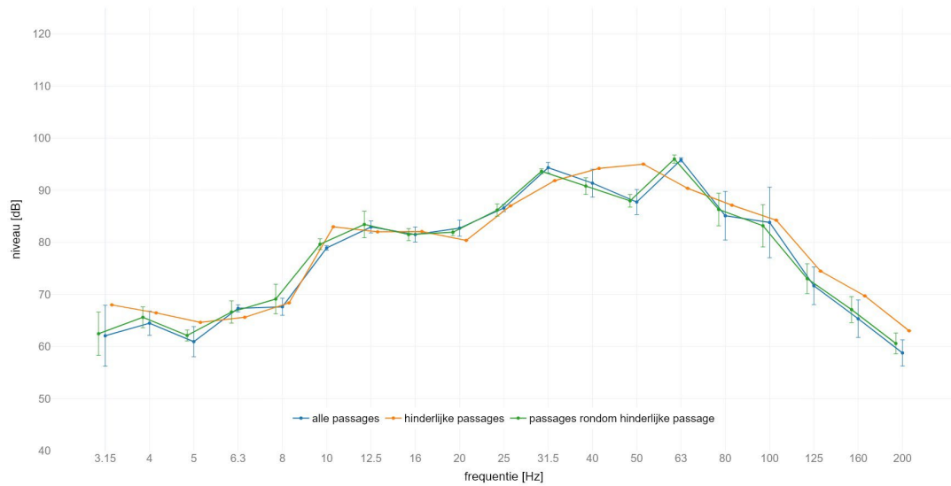
locatie America : gemiddeld spectrum passage met SPR op spoor 1 meetlocatie: zuid 8m C | meetrichting: Z | foutbalk met +/- standaard afwijking
