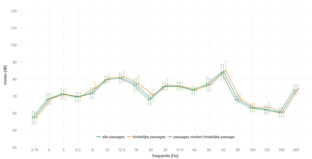
locatie Holten : gemiddeld spectrum passage met IC op spoor 2 meetlocatie: gebouw | meetrichting: Y | foutbalk met +/- standaard afwijking
