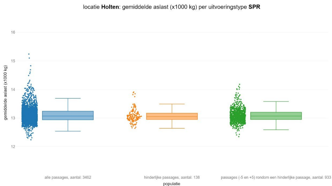
figuur 132 Gemiddelde aslast voor sprinters per populatie
