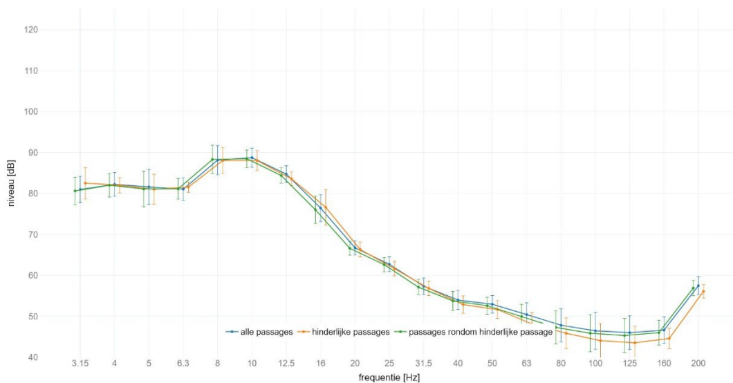
locatie Schalkwijk : gemiddeld spectrum passage met SPR op spoor 1 meetlocatie: gebouw | meetrichting: Y | foutbalk met +/- standaard afwijking
