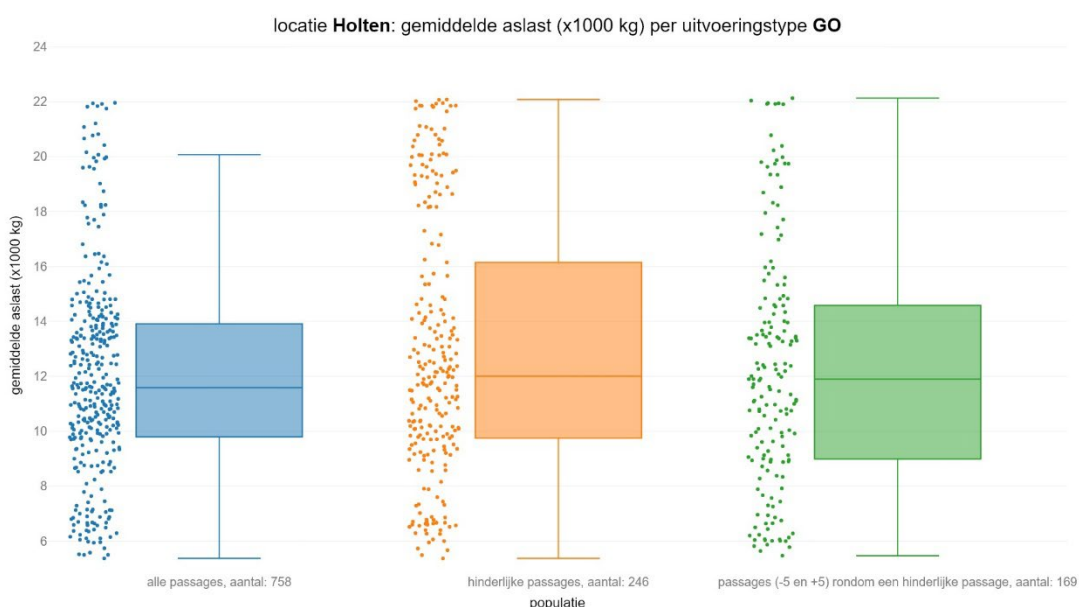
figuur 66 Gemiddelde aslast voor goederentreinen per populatie
