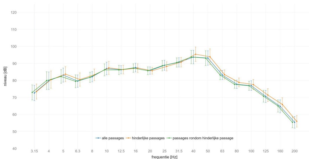
locatie America : gemiddeld spectrum passage met GO op spoor 2 meetlocatie: zuid 25m C | meetrichting: Z | foutbalk met +/- standaard afwijking
