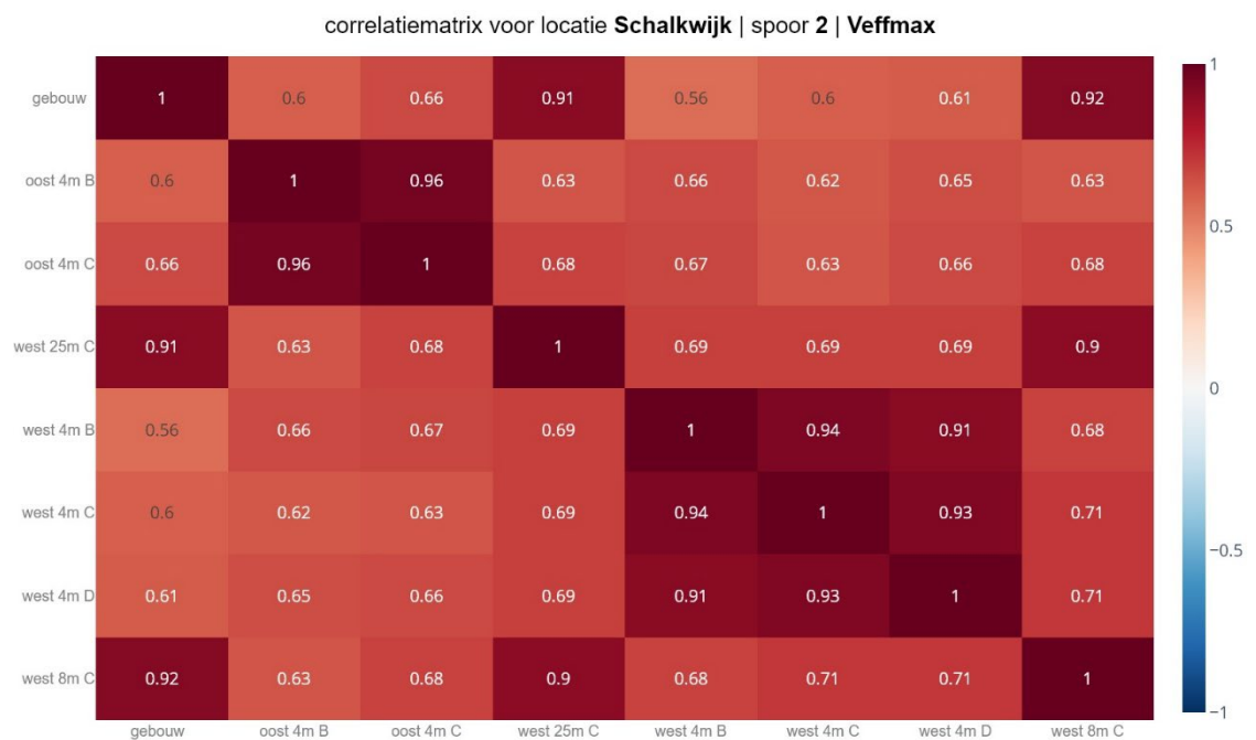
Correlatie matrix V_{eff,max} spoor 2
