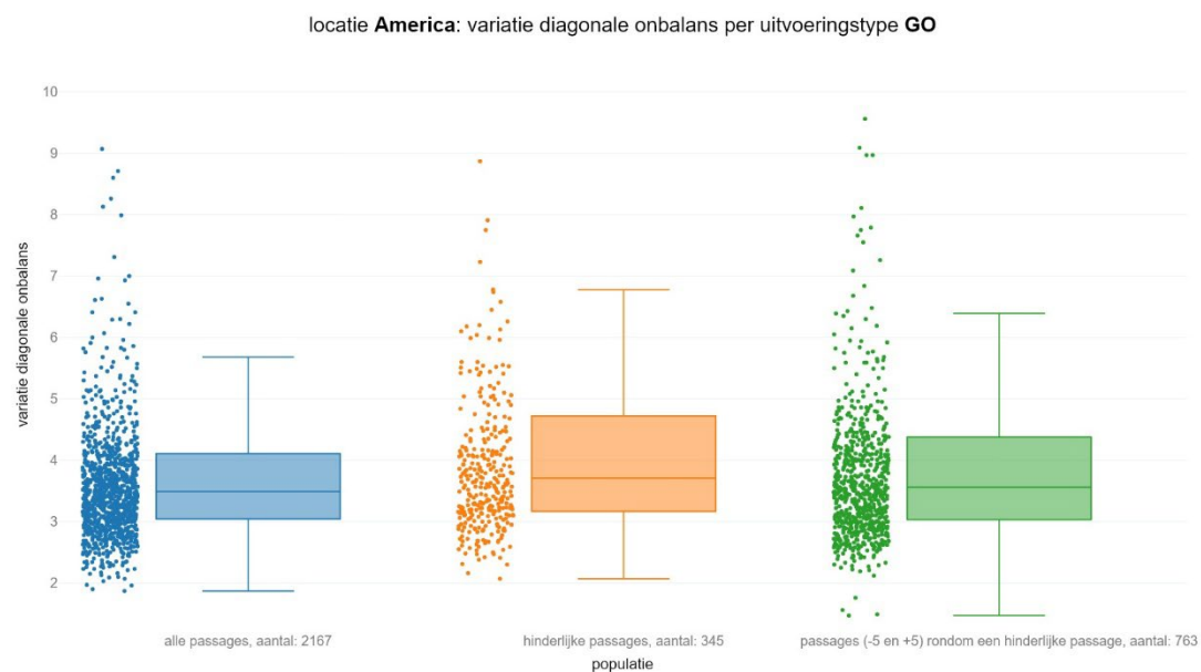
figuur 126 Variatie diagonale onbalans voor goederentreinen per populatie
