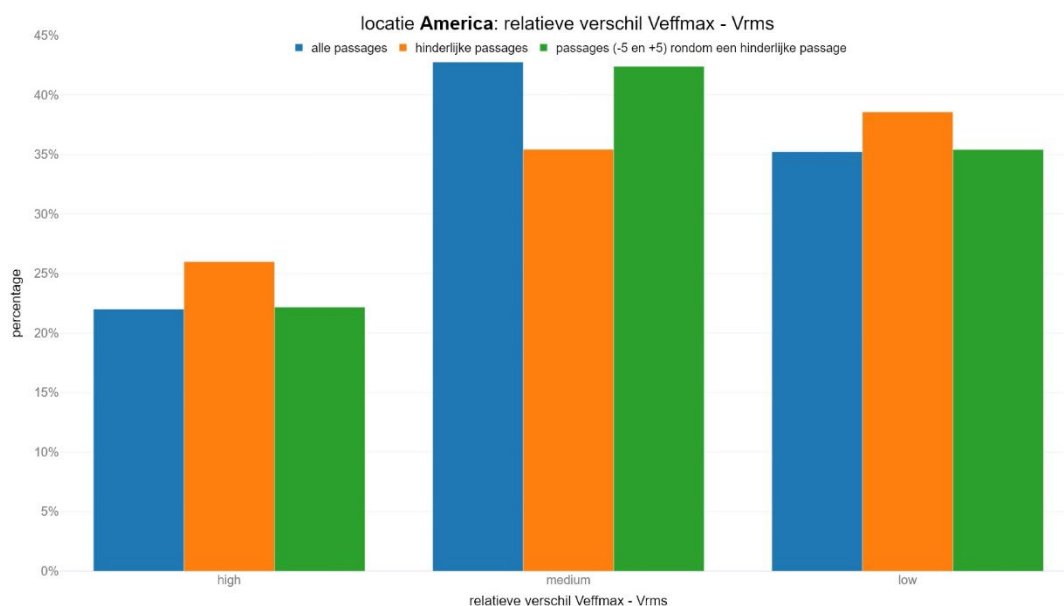
figuur 52 Relatieve verschil V_{eff,max} - V_{rms} verschil per populatie
