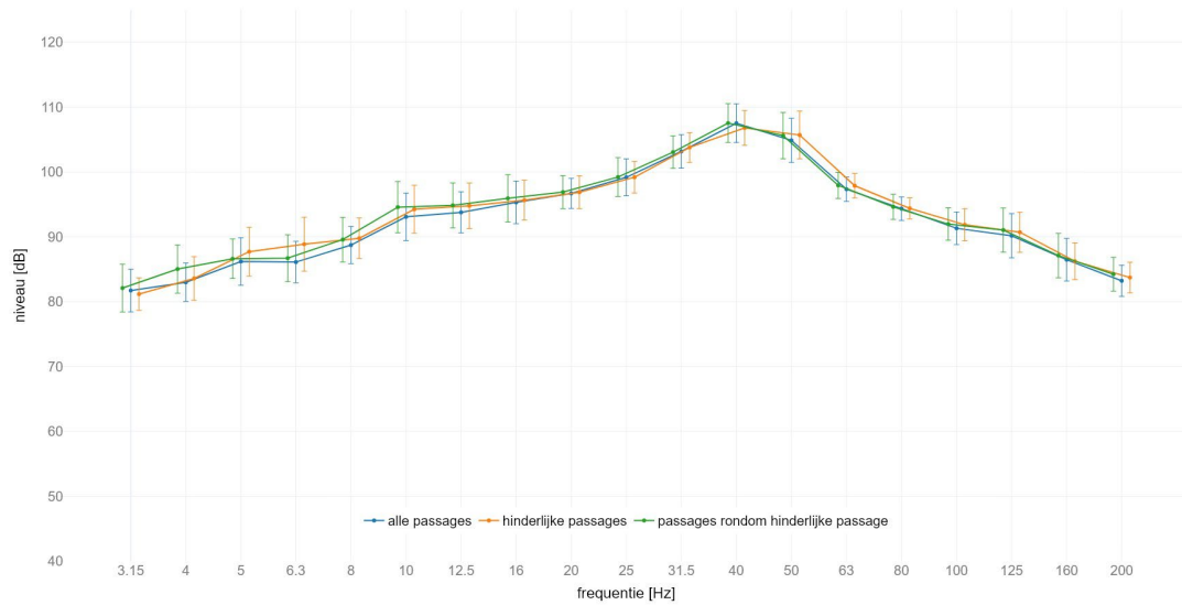
locatie Holten : gemiddeld spectrum passage met GO op spoor 2 meetlocatie: noord 4m C | meetrichting: Y | voetbalk met +/- standaard afwijking
