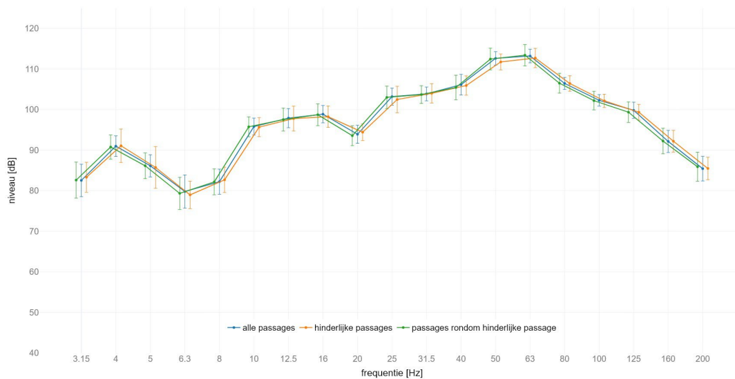
locatie Holten : gemiddeld spectrum passage met IC op spoor 2 meetlocatie: zuid 4m C | meetrichting: Y | voetbalk met +/- standaard afwijking
