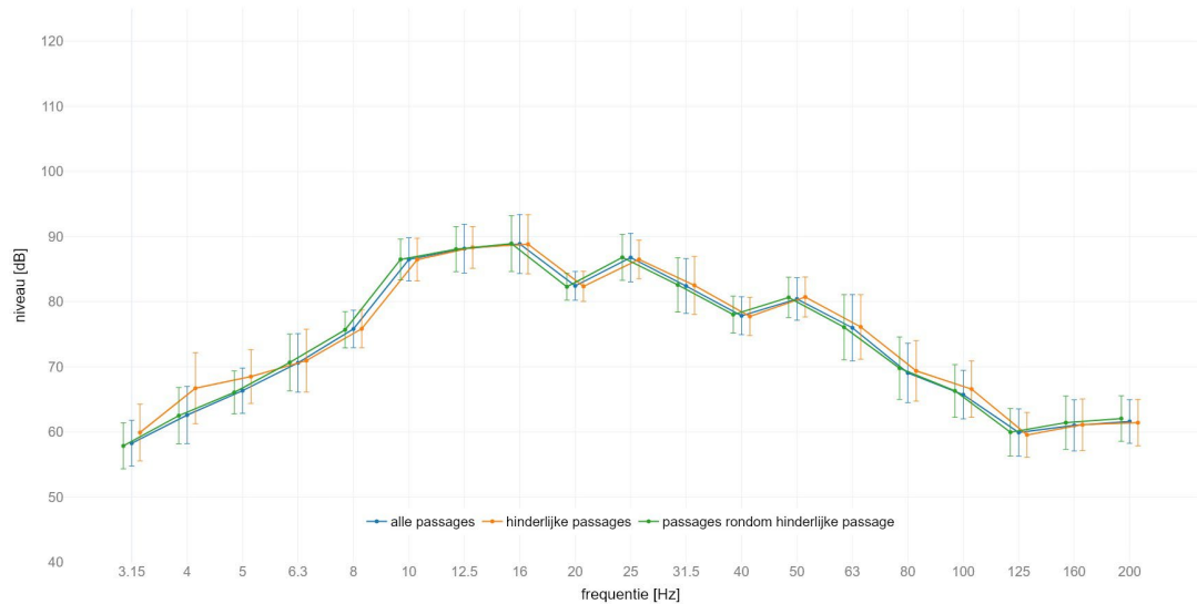
locatie Holten : gemiddeld spectrum passage met SPR op spoor 1 meetlocatie: noord 4m C | meetrichting: X | voetbalk met +/- standaard afwijking
