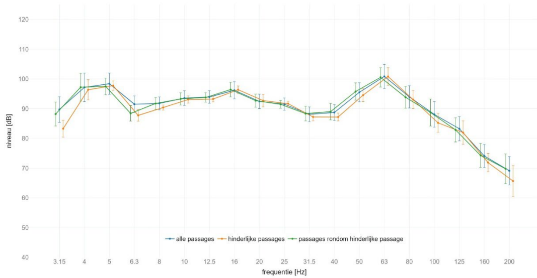
locatie Schalkwijk : gemiddeld spectrum passage met IC op spoor 2 meetlocatie: west 4m C | meetrichting: Y | foutbalk met +/- standaard afwijking
