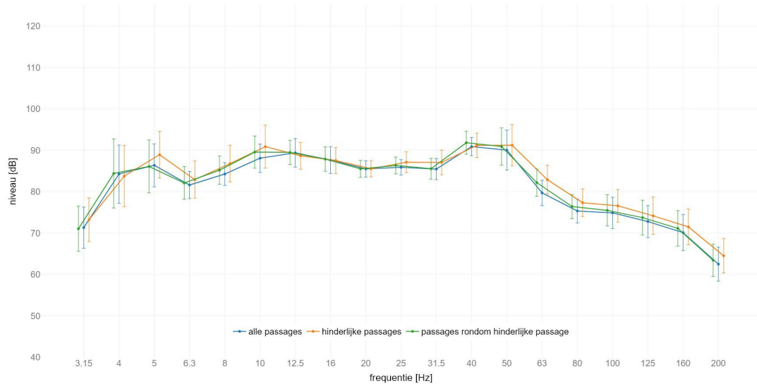
locatie Holten : gemiddeld spectrum passage met GO op spoor 1 meetlocatie: zuid 25m C | meetrichting: Y | foutbalk met +/- standaard afwijking
