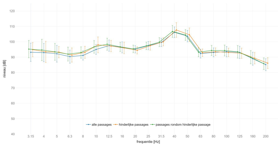
locatie Holten : gemiddeld spectrum passage met GO op spoor 1 meetlocatie: noord 4m C | meetrichting: X | voetbalk met +/- standaard afwijking
