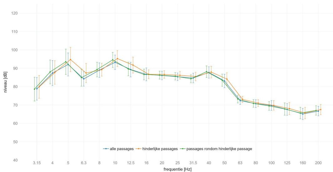
locatie Holten : gemiddeld spectrum passage met GO op spoor 2 meetlocatie: gebouw | meetrichting: Z | foutbalk met +/- standaard afwijking
