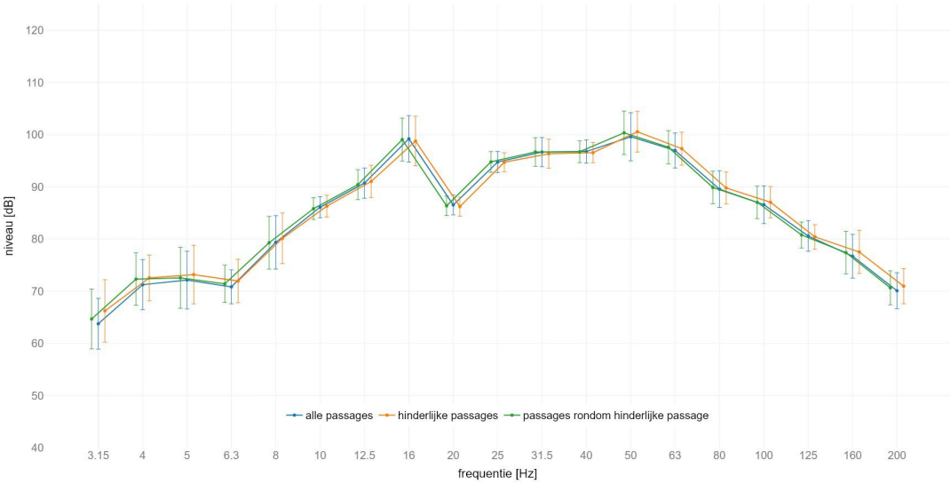
locatie Holten : gemiddeld spectrum passage met SPR op spoor 2 meetlocatie: zuid 25m C | meetrichting: Z | foutbalk met +/- standaard afwijking
