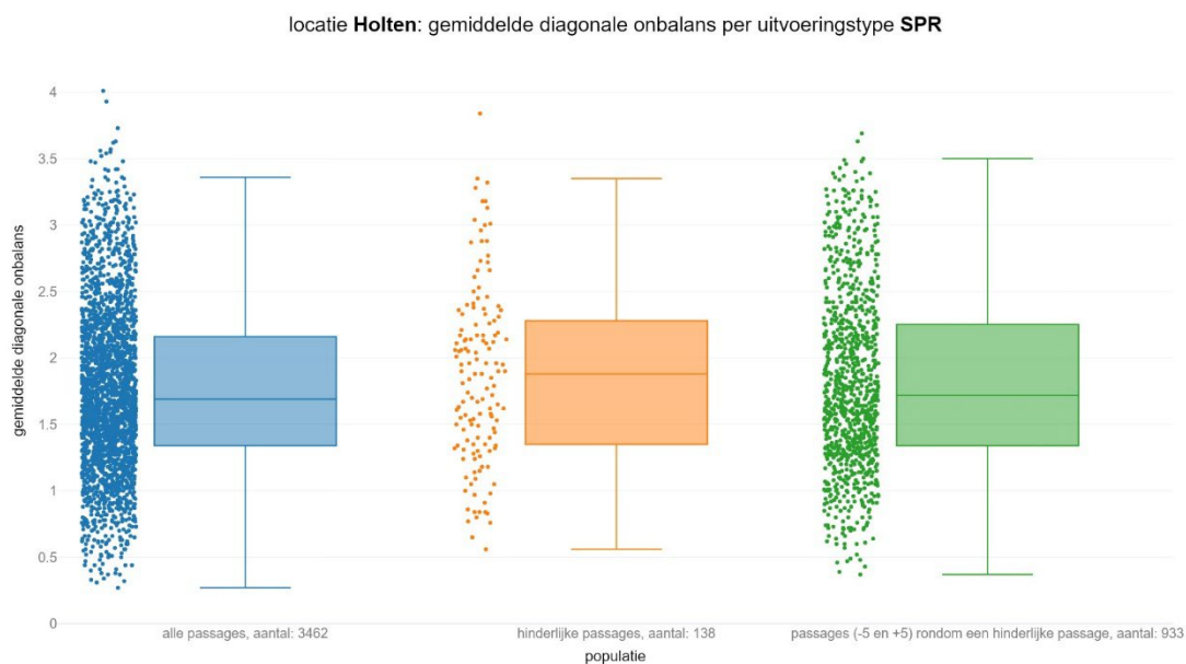
figuur 136 Gemiddelde diagonale onbalans voor sprinters per populatie
