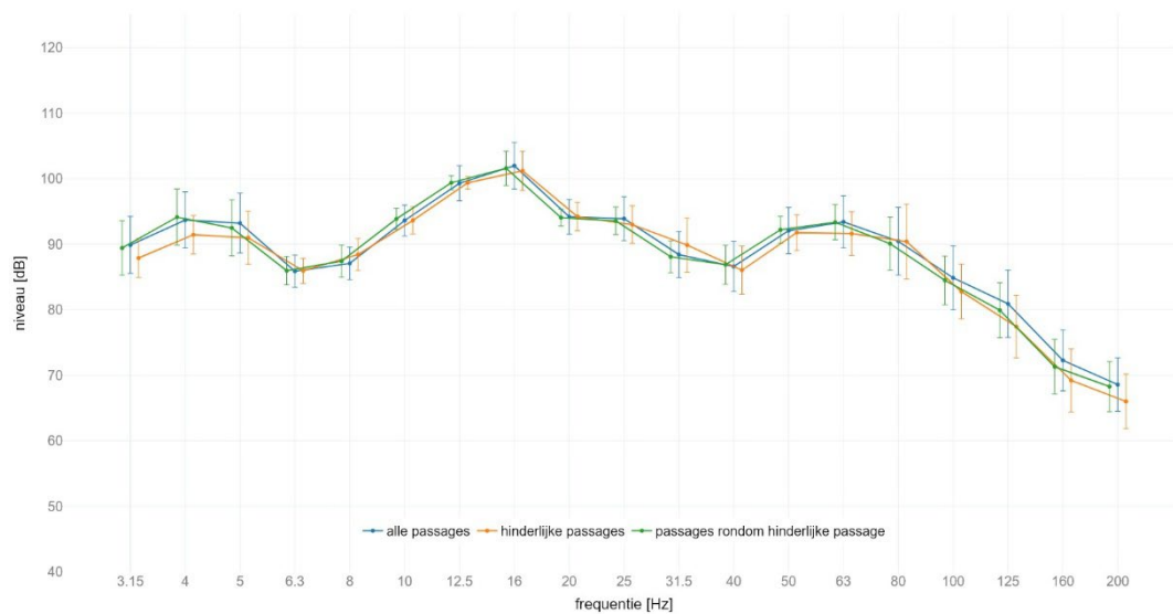
locatie Schalkwijk : gemiddeld spectrum passage met SPR op spoor 1 meetlocatie: west 4m C | meetrichting: Y | foutbalk met +/- standaard afwijking
