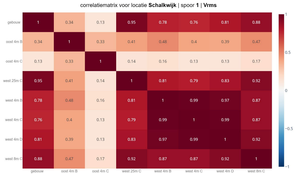
figuur 14 Correlatie matrix V_{rms} voor passage op spoor 1
