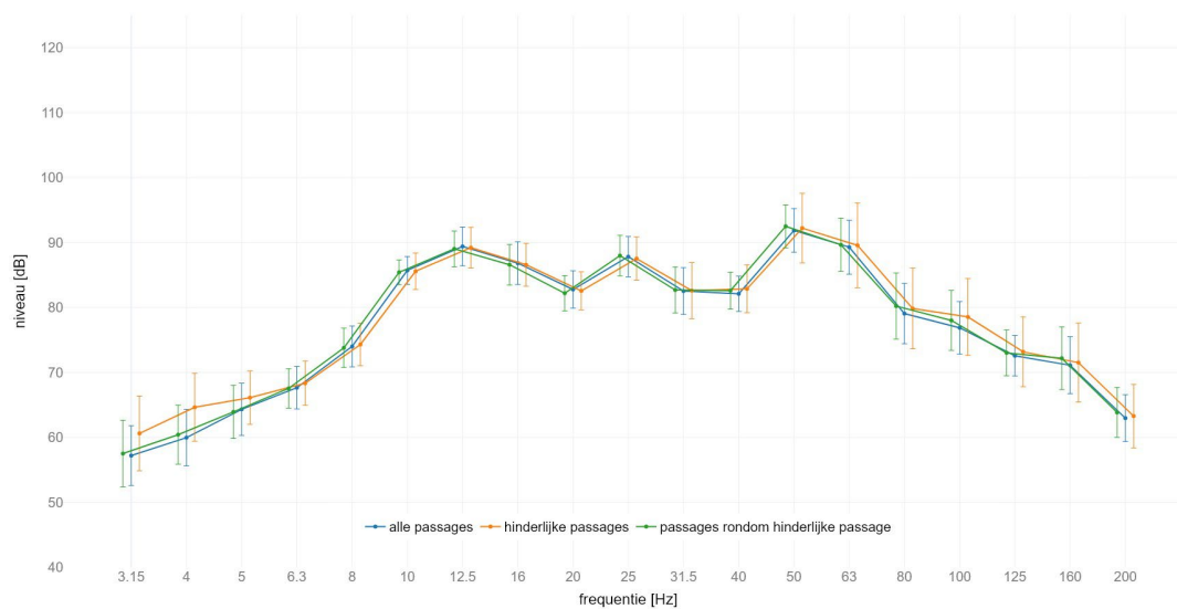
locatie Holten : gemiddeld spectrum passage met SPR op spoor 1 meetlocatie: zuid 25m C | meetrichting: Y | foutbalk met +/- standaard afwijking
