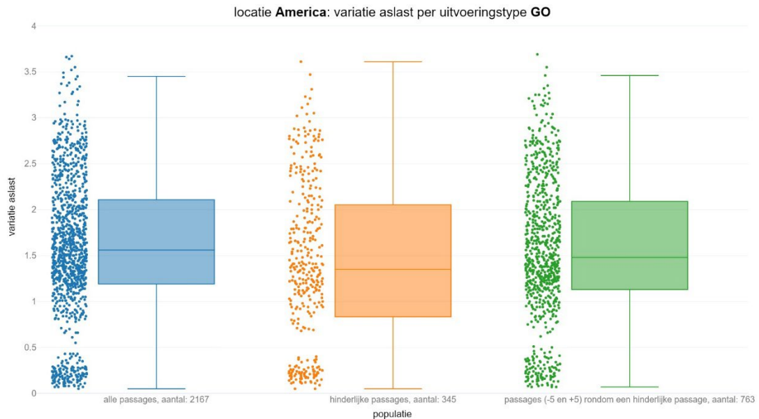
figuur 41 Variatie aslast voor goederentreinen per populatie
