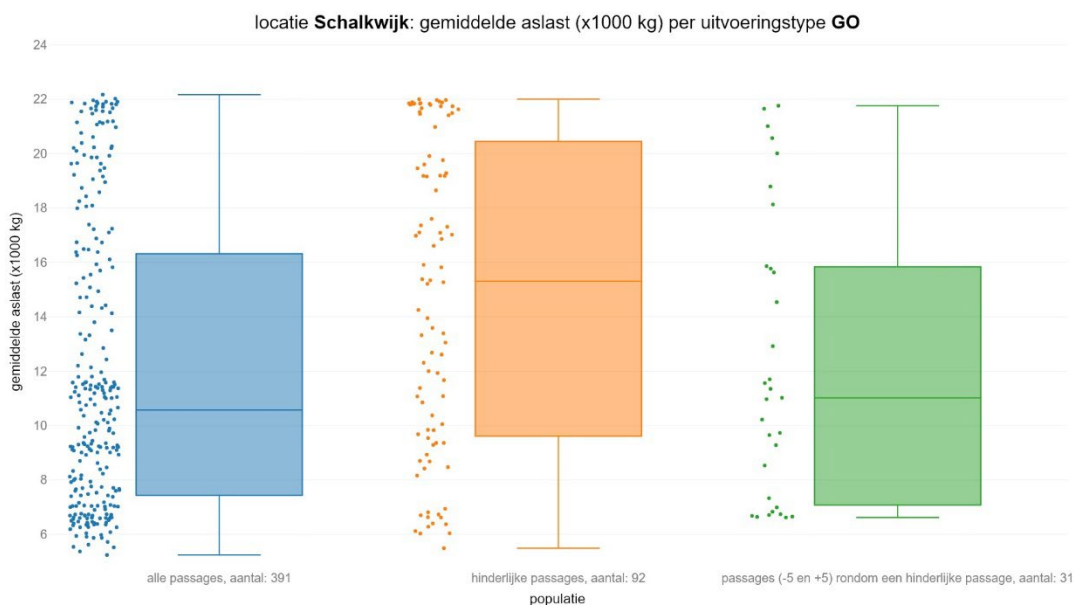
figuur 10 Gemiddelde aslast voor goederentreinen per populatie
