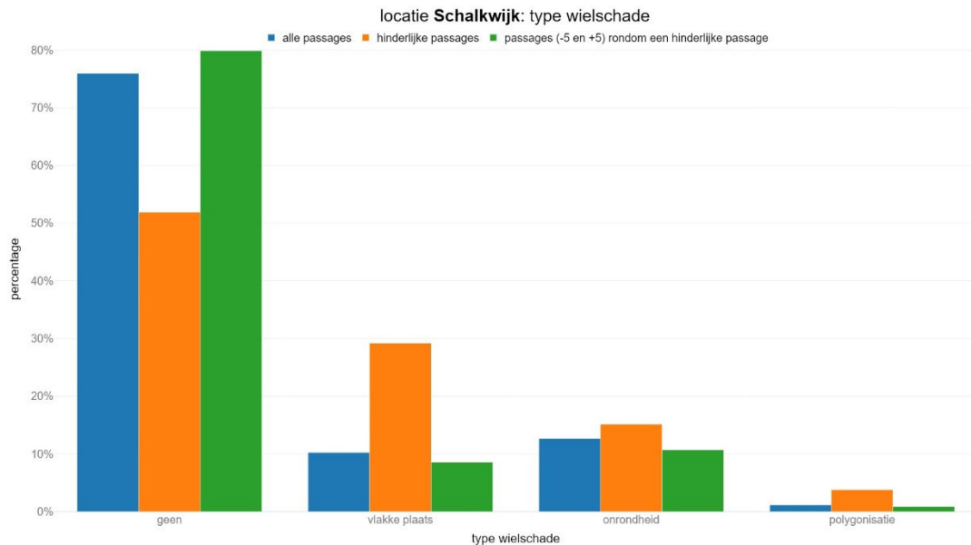
figuur 9 Type wielschade per populatie
