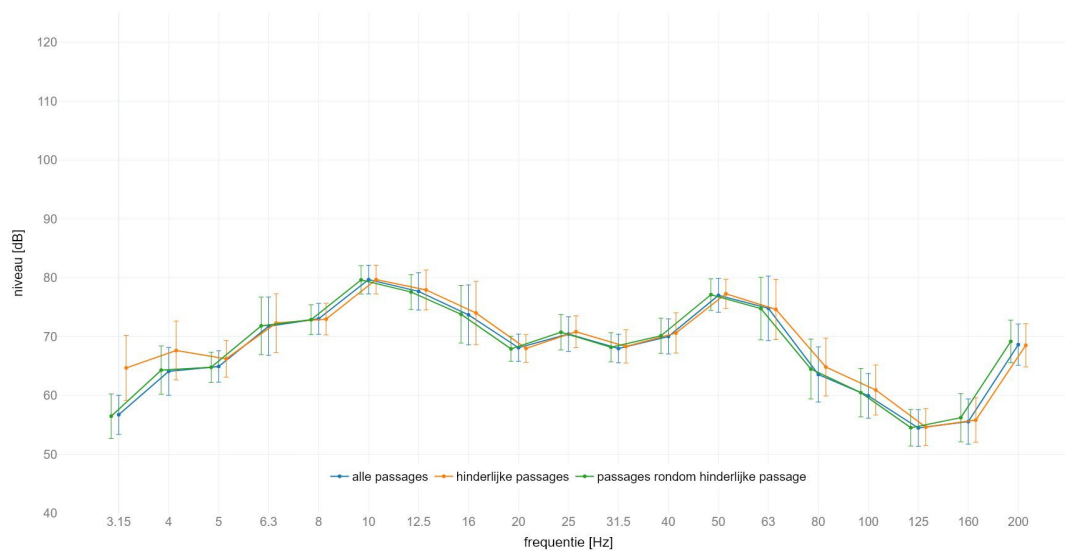
locatie Holten : gemiddeld spectrum passage met SPR op spoor 1 meetlocatie: gebouw | meetrichting: Y | foutbalk met +/- standaard afwijking
