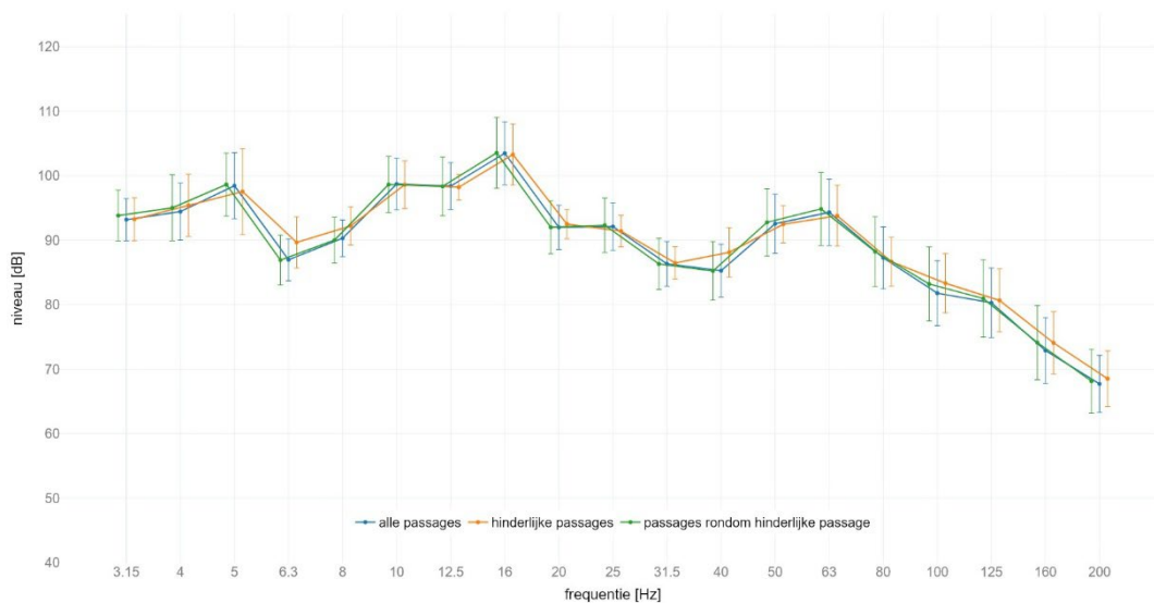
locatie Schalkwijk : gemiddeld spectrum passage met IC op spoor 1 meetlocatie: west 4m C | meetrichting: Z | foutbalk met +/- standaard afwijking
