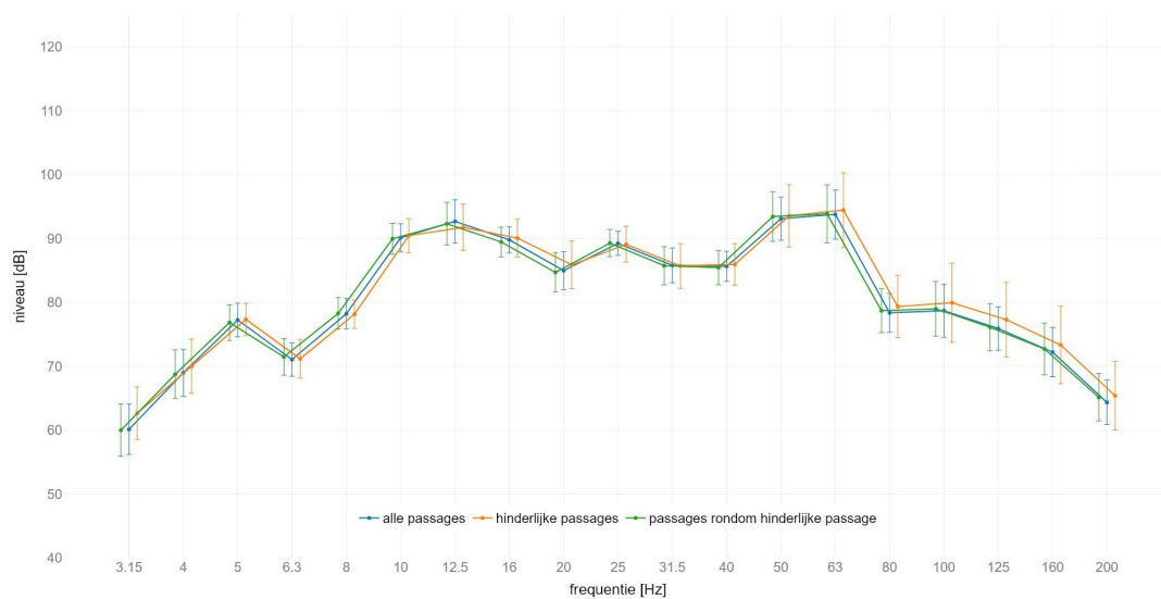
locatie Holten : gemiddeld spectrum passage met IC op spoor 1 meetlocatie: zuid 25m C | meetrichting: Z | foutbalk met +/- standaard afwijking
