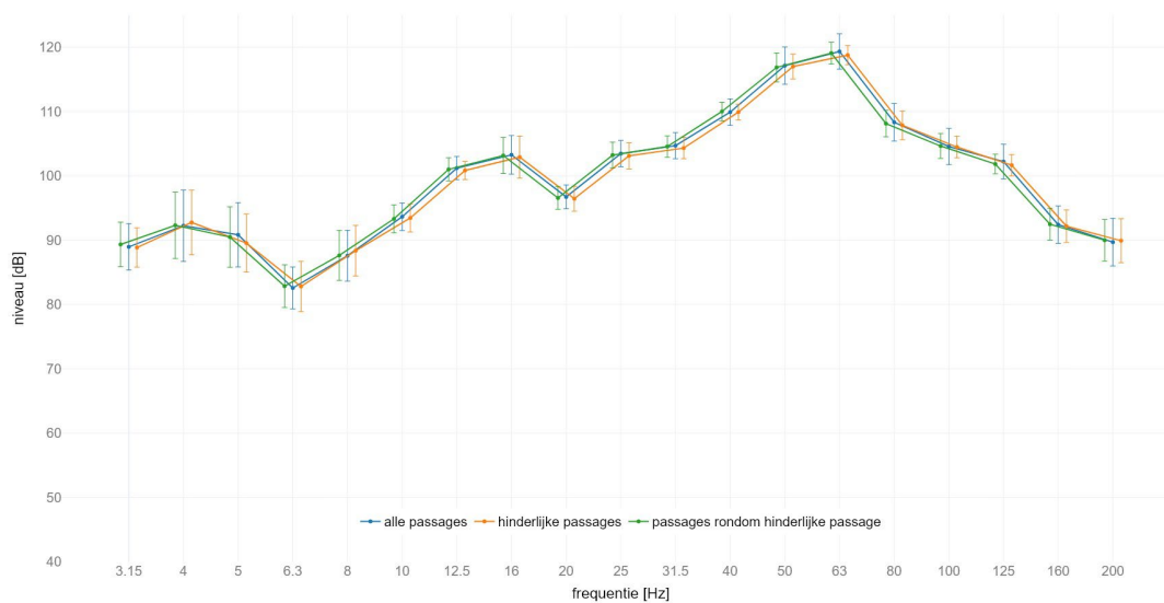
locatie Holten : gemiddeld spectrum passage met SPR op spoor 2 meetlocatie: zuid 4m C | meetrichting: Z | foutbalk met +/- standaard afwijking
