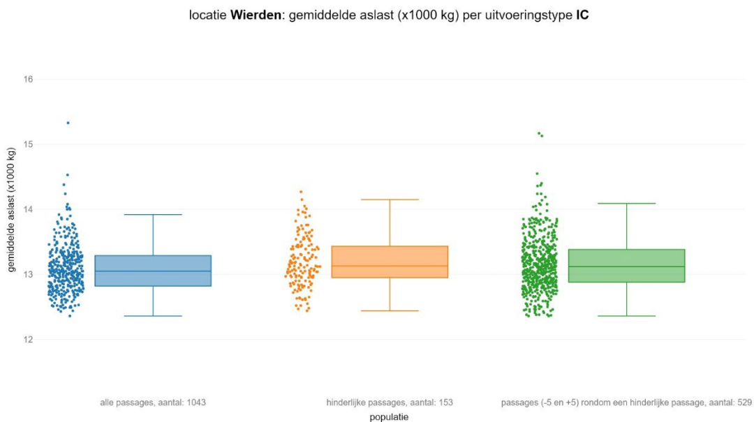
figuur 143 Gemiddelde aslast voor intercity's per populatie
