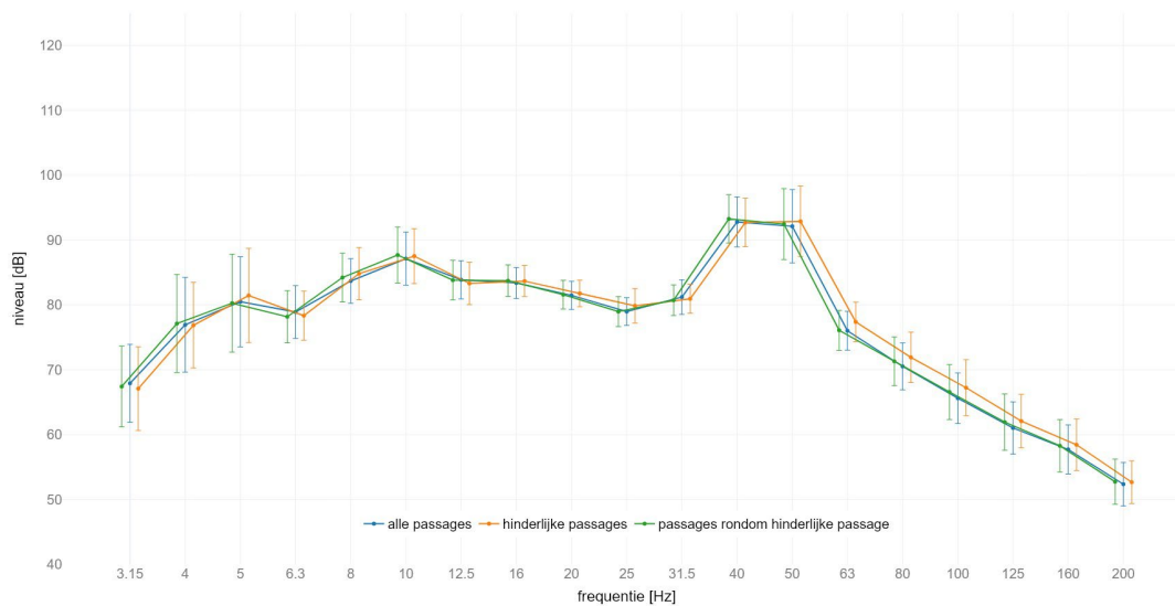
locatie America : gemiddeld spectrum passage met IC op spoor 1 meetlocatie: noord 4m B | meetrichting: Z | foutbalk met +/- standaard afwijking
