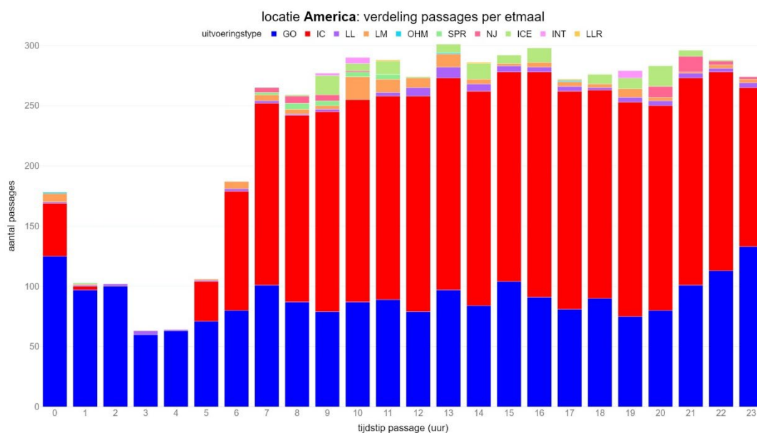
figuur 33 Verspreiding van passages van treinen over het etmaal
