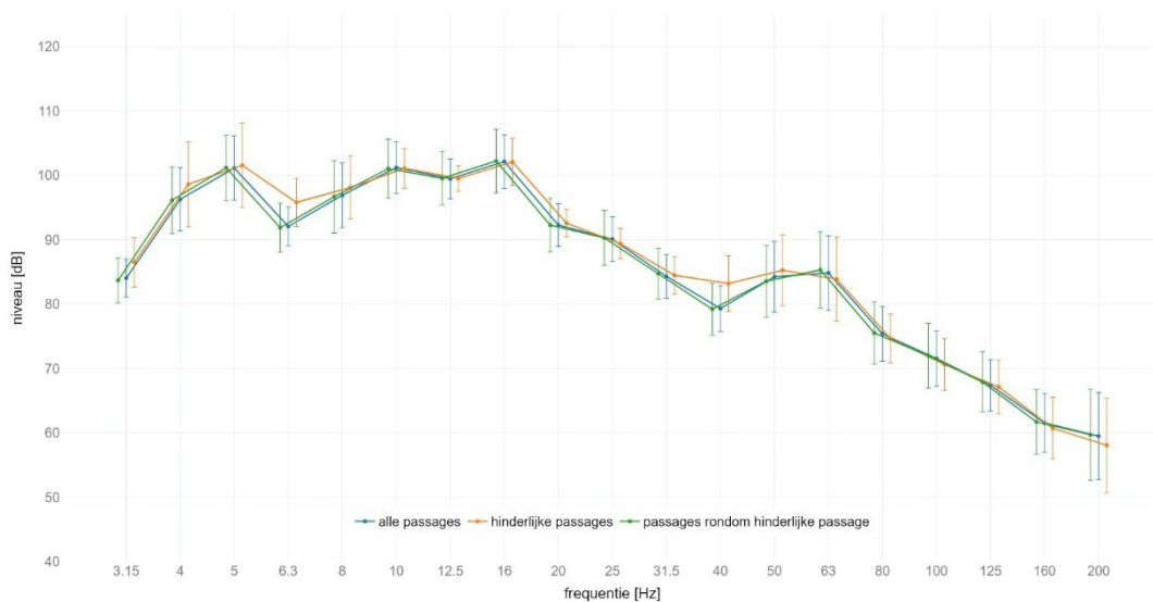
locatie Schalkwijk : gemiddeld spectrum passage met IC op spoor 1 meetlocatie: west 25m C | meetrichting: X | foutbalk met +/- standaard afwijking
