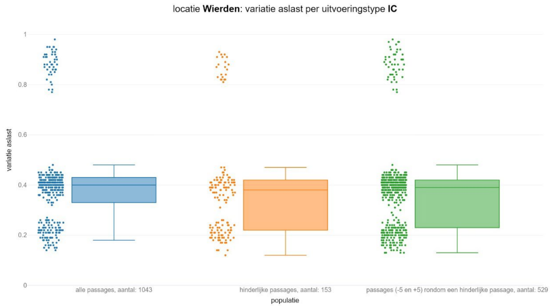
figuur 145 Variatie aslast voor intercity's per populatie
