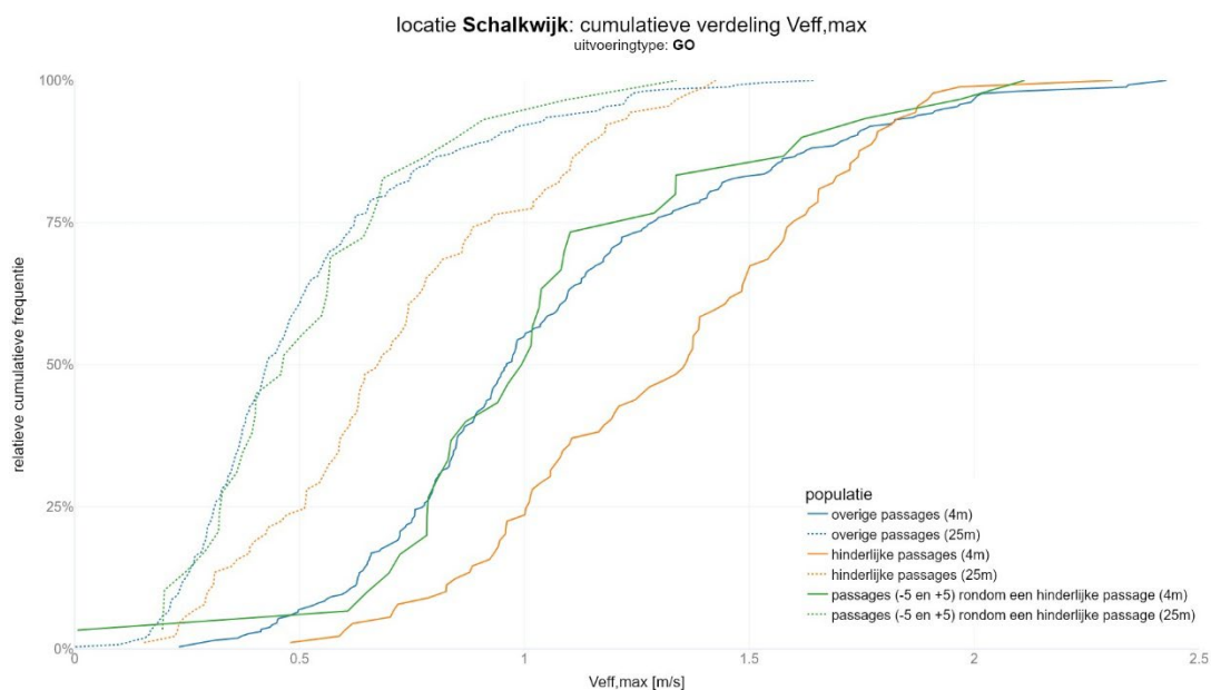
figuur 118 Cumulatieve verdeling van V_{eff,max} waarden voor goederentreinen
