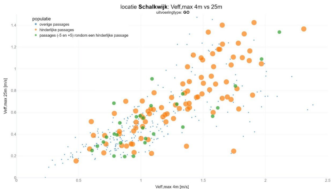
figuur 117 Verband tussen V_{eff,max} waarden op 4m en 25m voor goederentreinen en relatie met hinder
