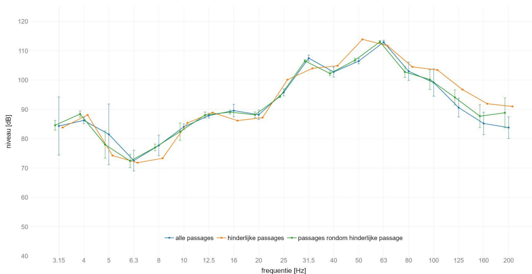
locatie America : gemiddeld spectrum passage met SPR op spoor 1 meetlocatie: zuid 4m B | meetrichting: Z | foutbalk met +/- standaard afwijking
