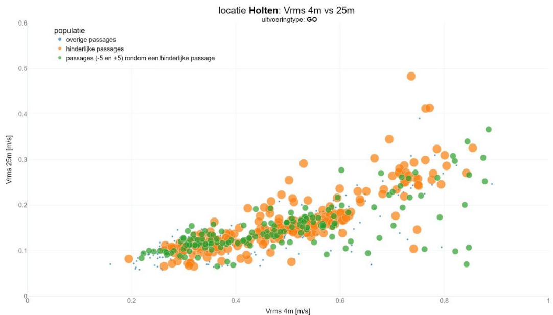
figuur 74 Verband tussen V_{rms} waardes voor goederentreinen op 4m en 25m en relatie met hinder
