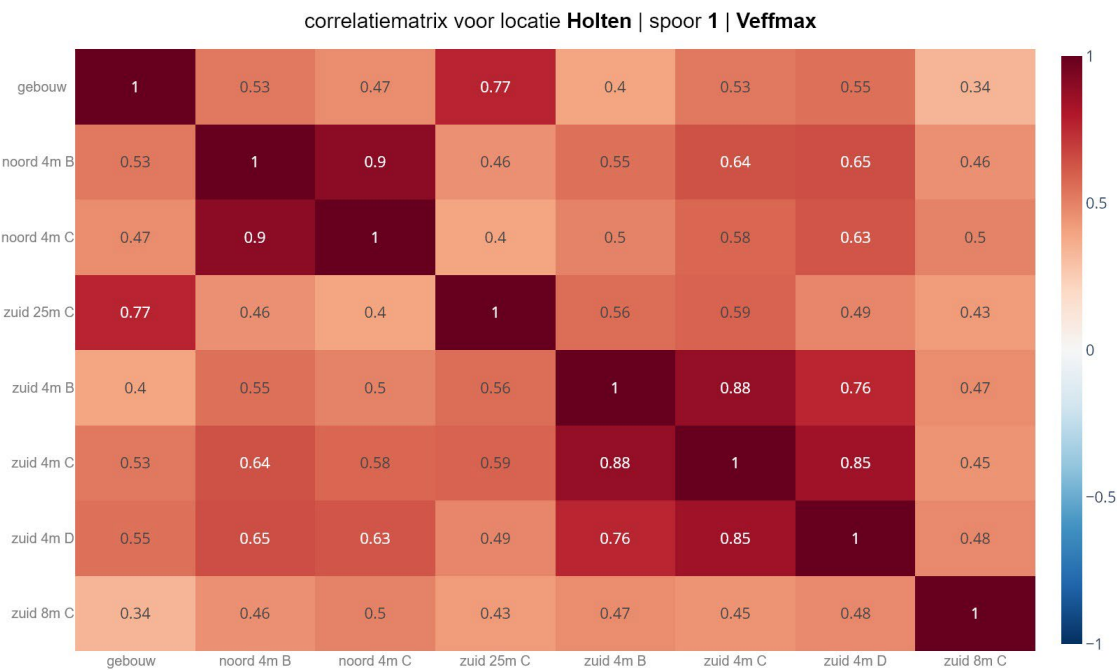
figuur 139 Correlatie matrix V_{eff,max} spoor 1
