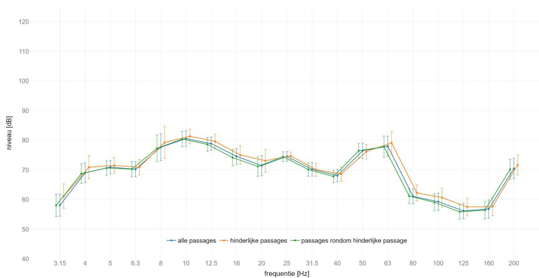
locatie Holten : gemiddeld spectrum passage met IC op spoor 1 meetlocatie: gebouw | meetrichting: Z | voetbalk met +/- standaard afwijking
