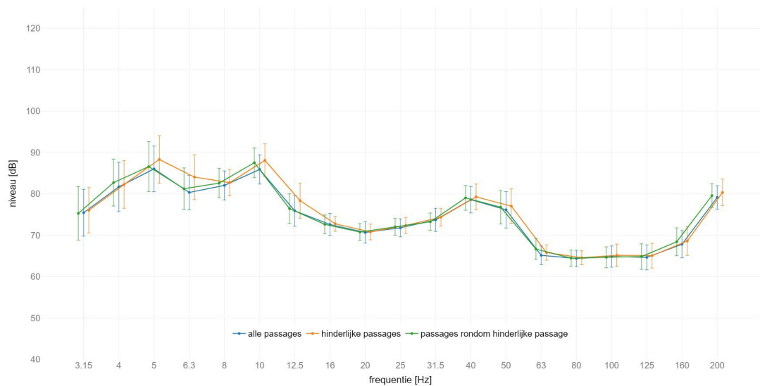
locatie Holten : gemiddeld spectrum passage met GO op spoor 2 meetlocatie: gebouw | meetrichting: X | foutbalk met +/- standaard afwijking
