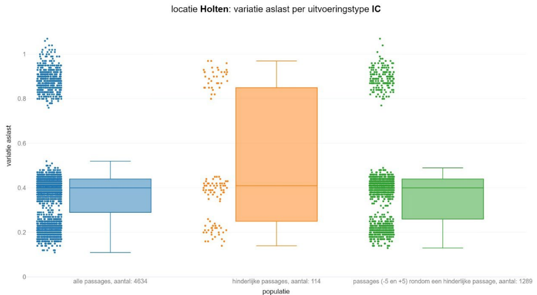
figuur 67 Variatie aslast voor intercity's per populatie
