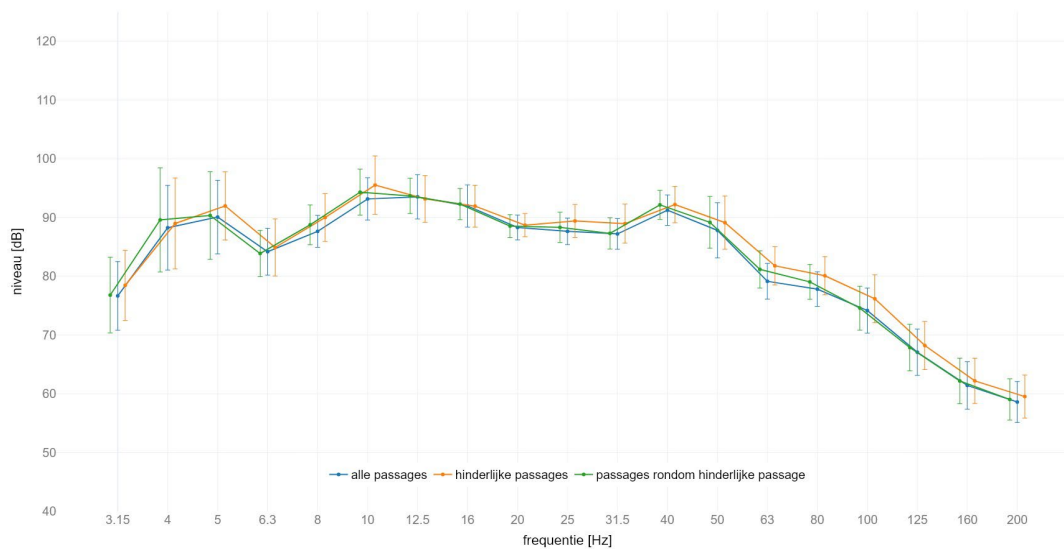
locatie Holten : gemiddeld spectrum passage met IC op spoor 1 meetlocatie: gebouw | meetrichting: X | foutebalk met +/- standaard afwijking
