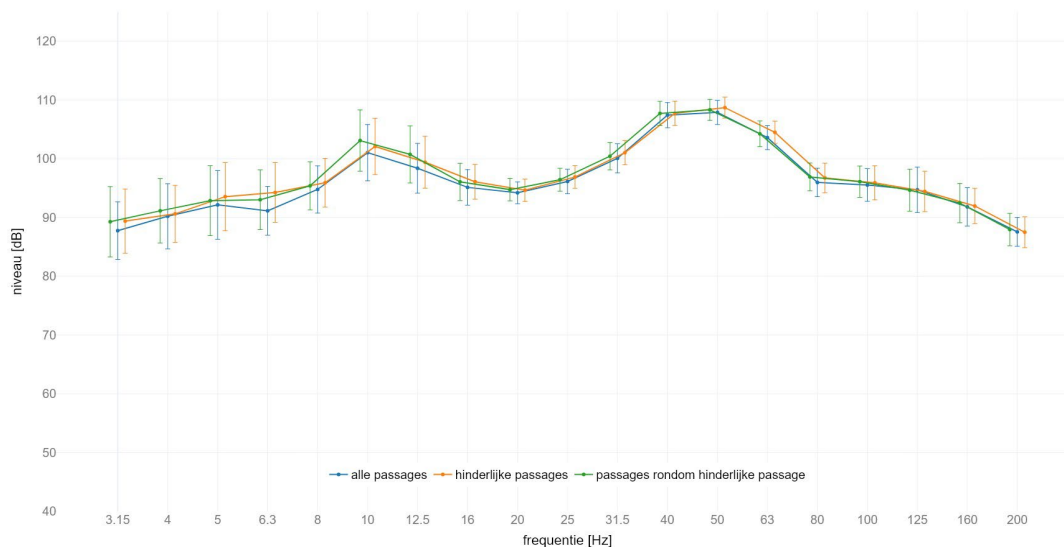
locatie Holten : gemiddeld spectrum passage met GO op spoor 2 meetlocatie: zuid 4m C | meetrichting: X | foutbalk met +/- standaard afwijking
