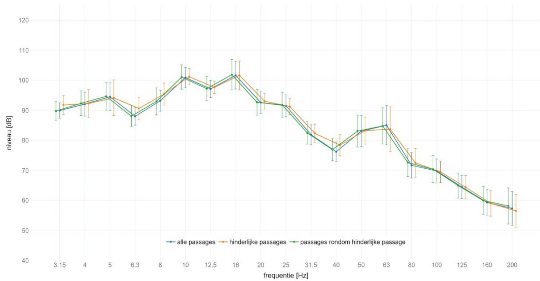
locatie Schalkwijk : gemiddeld spectrum passage met IC op spoor 1 meetlocatie: west 8m C | meetrichting: Y | voetbalk met +/- standaard afwijking
