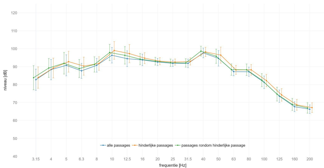
locatie Holten : gemiddeld spectrum passage met GO op spoor 2 meetlocatie: zuid 25m C | meetrichting: Z | foutbalk met +/- standaard afwijking
