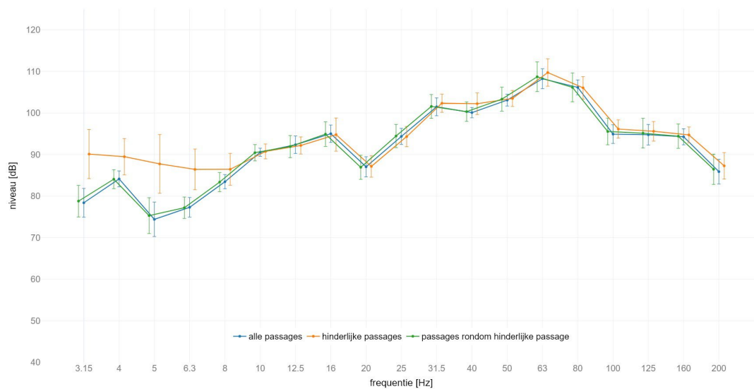
locatie America : gemiddeld spectrum passage met IC op spoor 2 meetlocatie: zuid 4m B | meetrichting: Z | foutbalk met +/- standaard afwijking
