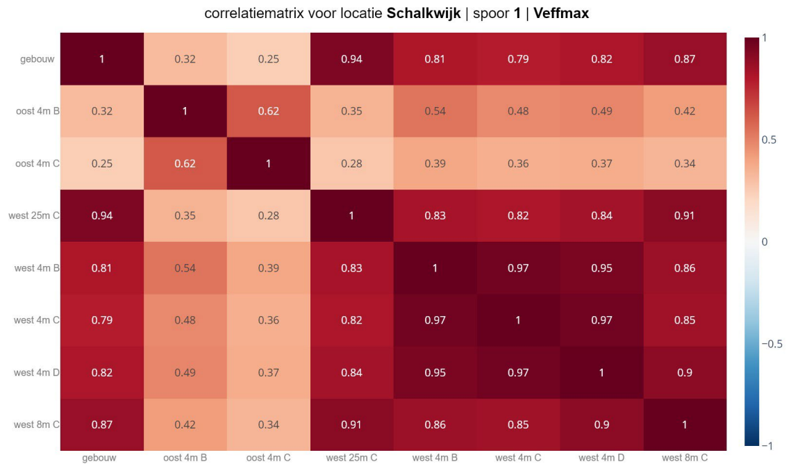
Correlatie matrix V_{eff,max} spoor 1
