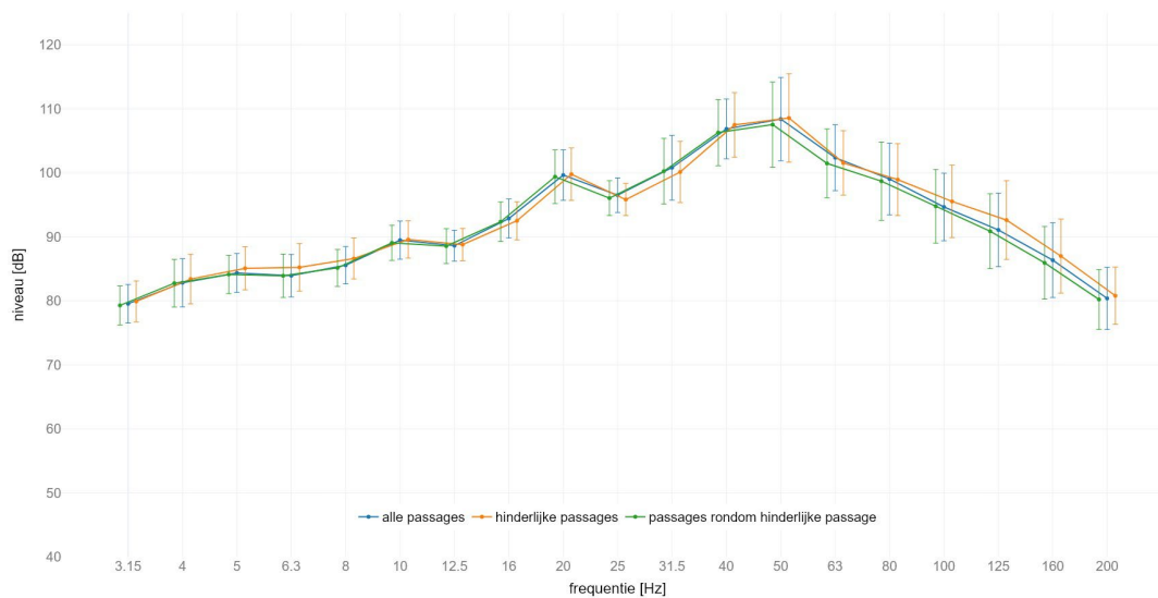
locatie America : gemiddeld spectrum passage met GO op spoor 2 meetlocatie: noord 4m C | meetrichting: Z | foutebalk met +/- standaard afwijking
