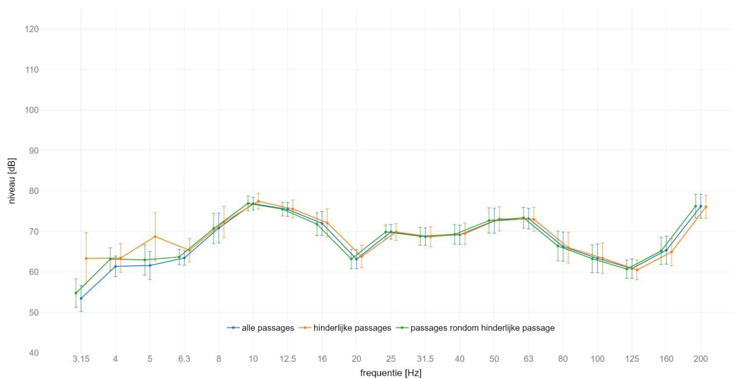
locatie Holten : gemiddeld spectrum passage met SPR op spoor 2 meetlocatie: gebouw | meetrichting: X | foutbalk met +/- standaard afwijking
