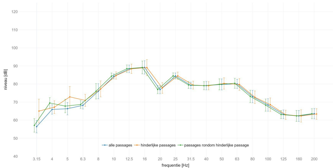
locatie Holten : gemiddeld spectrum passage met SPR op spoor 2 meetlocatie: gebouw | meetrichting: Z | foutbalk met +/- standaard afwijking
