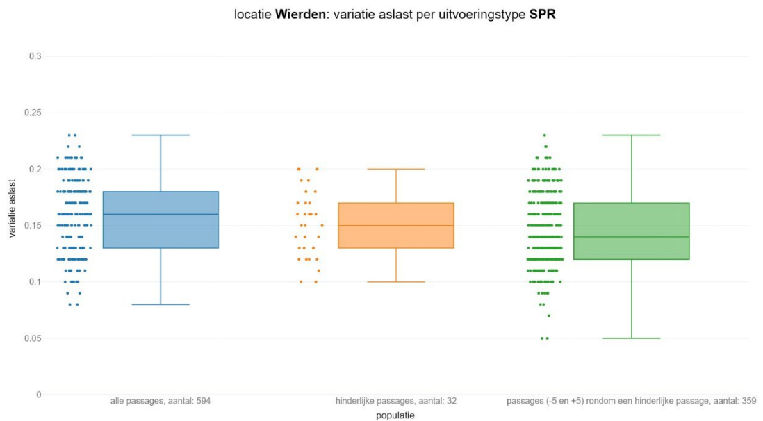
figuur 146 Variatie aslast voor sprinters per populatie
