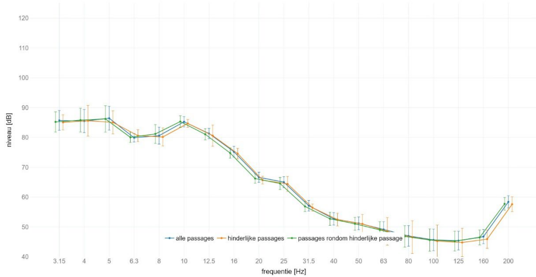
locatie Schalkwijk : gemiddeld spectrum passage met SPR op spoor 2 meetlocatie: gebouw | meetrichting: X | foutbalk met +/- standaard afwijking
