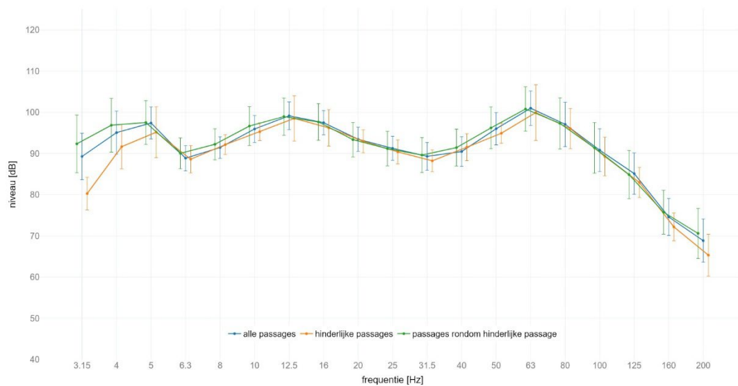
locatie Schalkwijk : gemiddeld spectrum passage met SPR op spoor 2 meetlocatie: oost 4m C | meetrichting: Z | foutelek met +/- standaard afwijking
