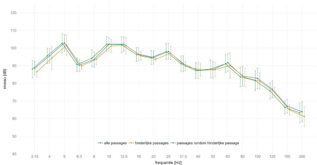
locatie Schalkwijk : gemiddeld spectrum passage met SPR op spoor 2 meetlocatie: west 25m C | meetrichting: X | foutelek met +/- standaard afwijking
