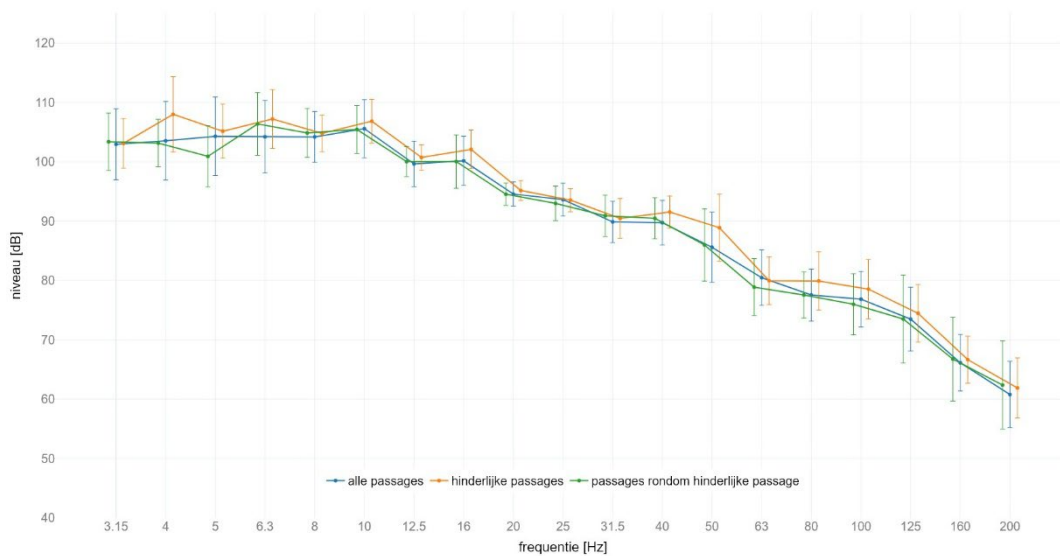
locatie Schalkwijk : gemiddeld spectrum passage met GO op spoor 2 meetlocatie: west 8m C | meetrichting: Y | foutbalk met +/- standaard afwijking
