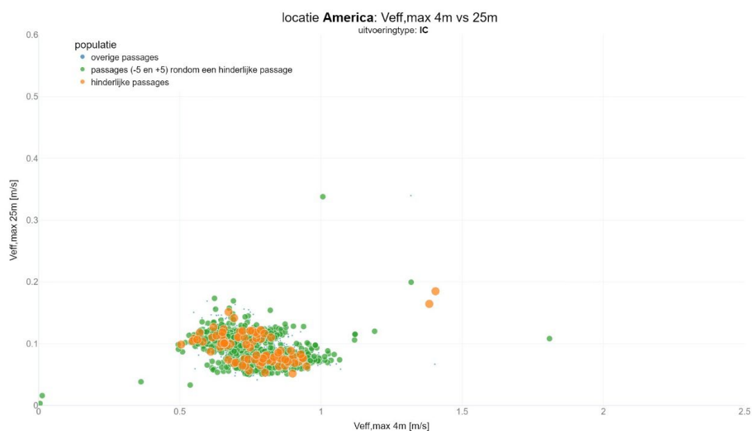
figuur 130 Verband tussen V_{eff,max} waardes op 4m en 25m voor intercity's en relatie met hinder
