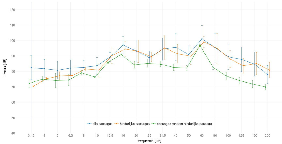
locatie America : gemiddeld spectrum passage met SPR op spoor 2 meetlocatie: noord 4m C | meetrichting: Z | foutbalk met +/- standaard afwijking
