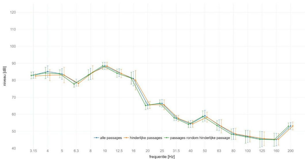
locatie Schalkwijk : gemiddeld spectrum passage met IC op spoor 1 meetlocatie: gebouw | meetrichting: Z | foutbalk met +/- standaard afwijking
