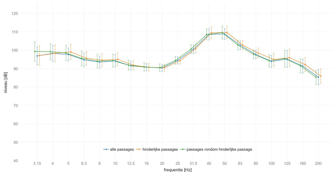
locatie America : gemiddeld spectrum passage met GO op spoor 2 meetlocatie: zuid 4m C | meetrichting: Y | foutbalk met +/- standaard afwijking
