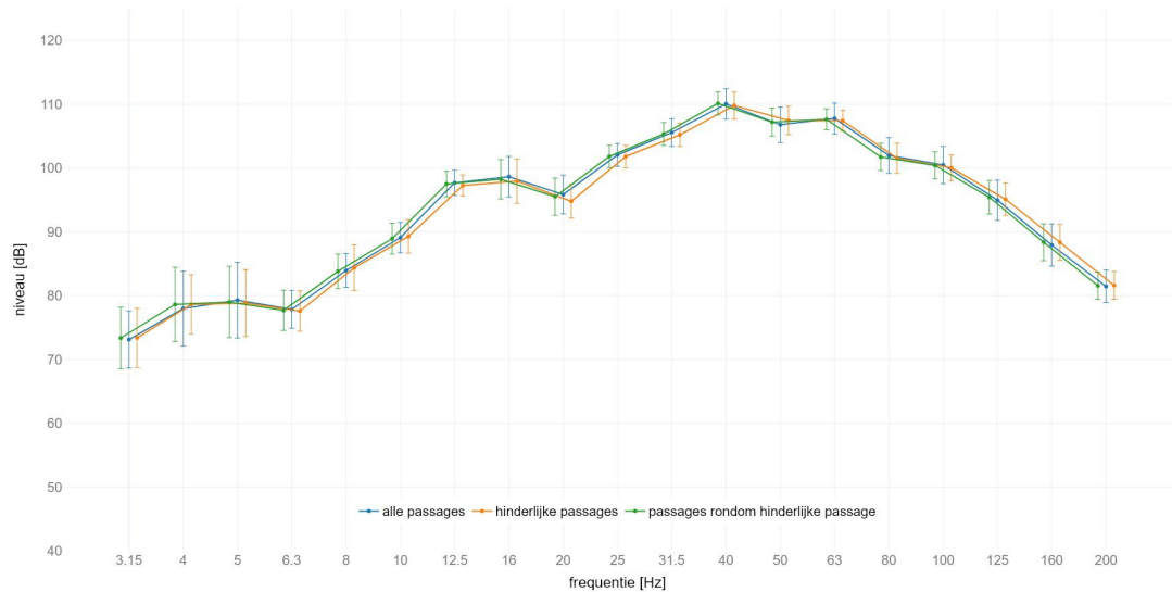
locatie Holten : gemiddeld spectrum passage met SPR op spoor 2 meetlocatie: zuid 8m C | meetrichting: Y | foutbalk met +/- standaard afwijking
