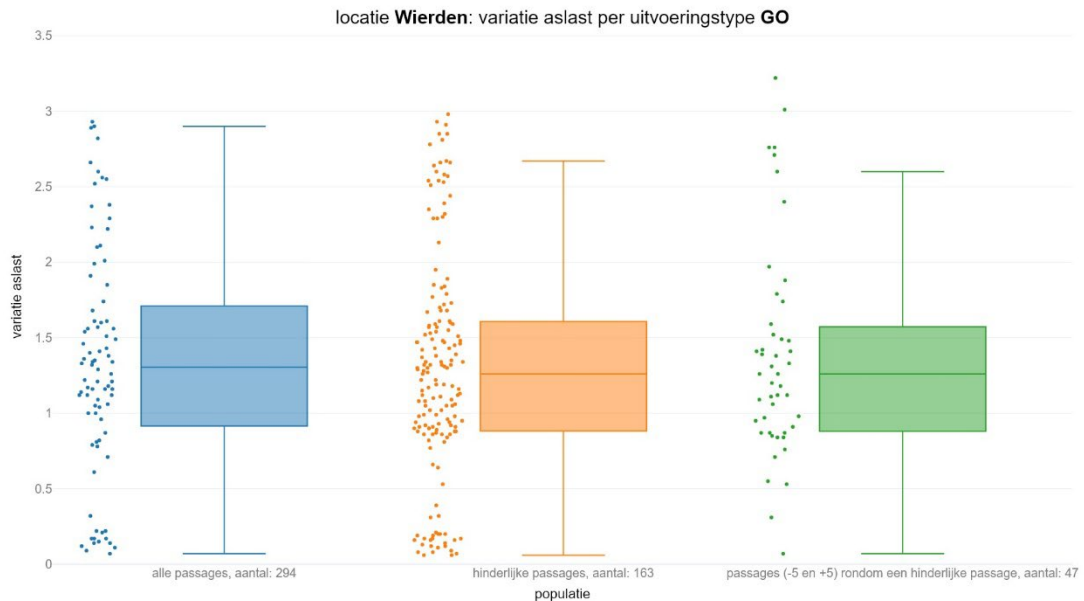
figuur 97 Variatie aslast per voor goederentreinen populatie
