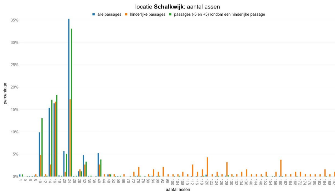
figuur 7 Aantal assen per populatie
