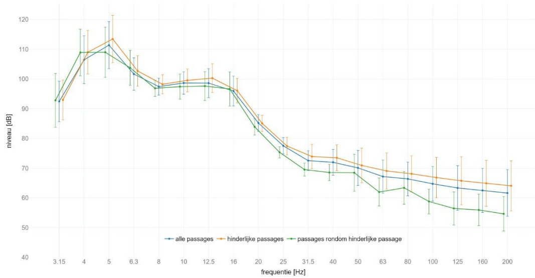
locatie Schalkwijk : gemiddeld spectrum passage met IC op spoor 1 meetlocatie: gebouw | meetrichting: X | foutbalk met +/- standaard afwijking
