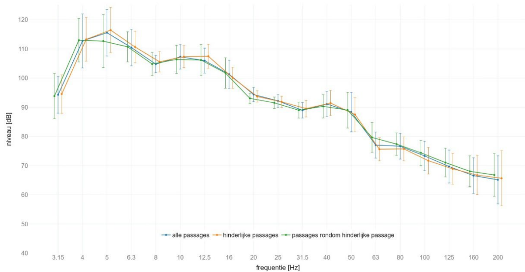
locatie Schalkwijk : gemiddeld spectrum passage met GO op spoor 1 meetlocatie: west 8m C | meetrichting: Z | foutbalk met +/- standaard afwijking
