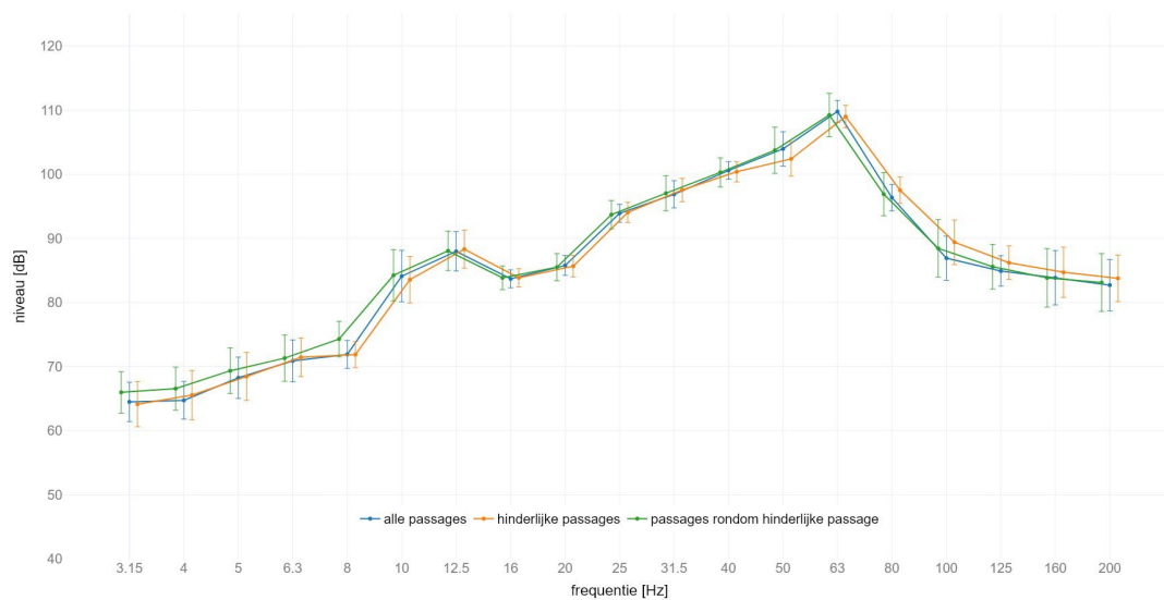
locatie America : gemiddeld spectrum passage met IC op spoor 1 meetlocatie: zuid 4m D | meetrichting: Z | foutbalk met +/- standaard afwijking
