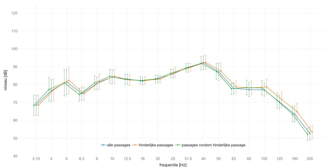
locatie America : gemiddeld spectrum passage met GO op spoor 1 meetlocatie: zuid 25m C | meetrichting: Y | foutbalk met +/- standaard afwijking
