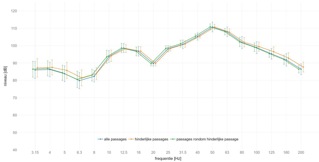
locatie Holten : gemiddeld spectrum passage met SPR op spoor 2 meetlocatie: zuid 4m C | meetrichting: X | foutbalk met +/- standaard afwijking
