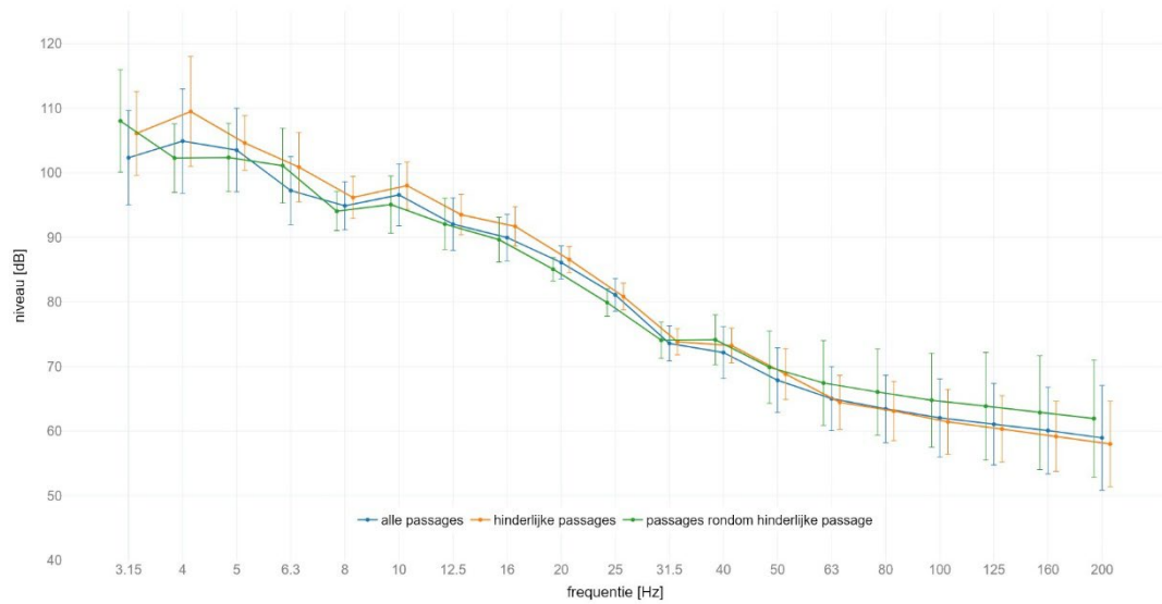
locatie Schalkwijk : gemiddeld spectrum passage met GO op spoor 2 meetlocatie: west 25m C | meetrichting: X | foutelek met +/- standaard afwijking
