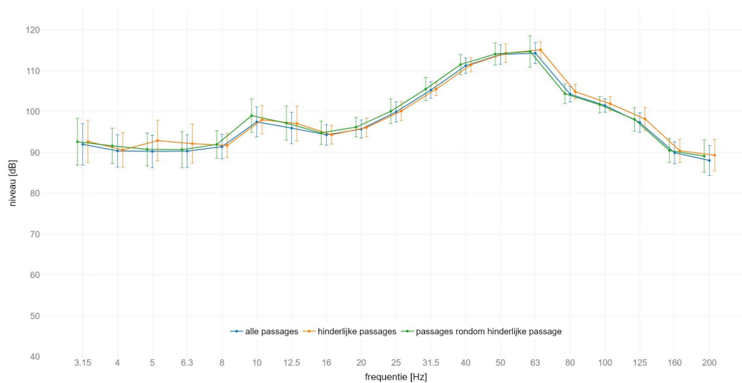
locatie Holten : gemiddeld spectrum passage met GO op spoor 2 meetlocatie: zuid 4m C | meetrichting: Z | foutbalk met +/- standaard afwijking
