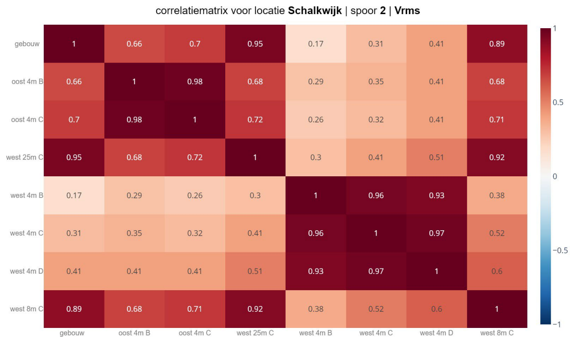
figuur 15 Correlatie matrix V_{rms} voor passage op spoor 2
