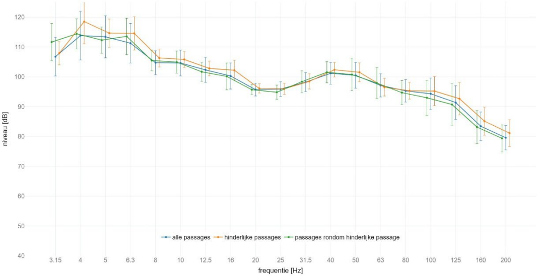
locatie Schalkwijk : gemiddeld spectrum passage met GO op spoor 2 meetlocatie: west 4m C | meetrichting: Z | foutbalk met +/- standaard afwijking
