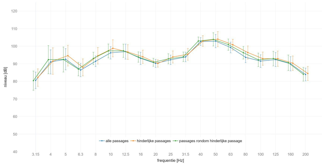
locatie Holten : gemiddeld spectrum passage met GO op spoor 1 meetlocatie: zuid 8m C | meetrichting: X | foutbalk met +/- standaard afwijking
