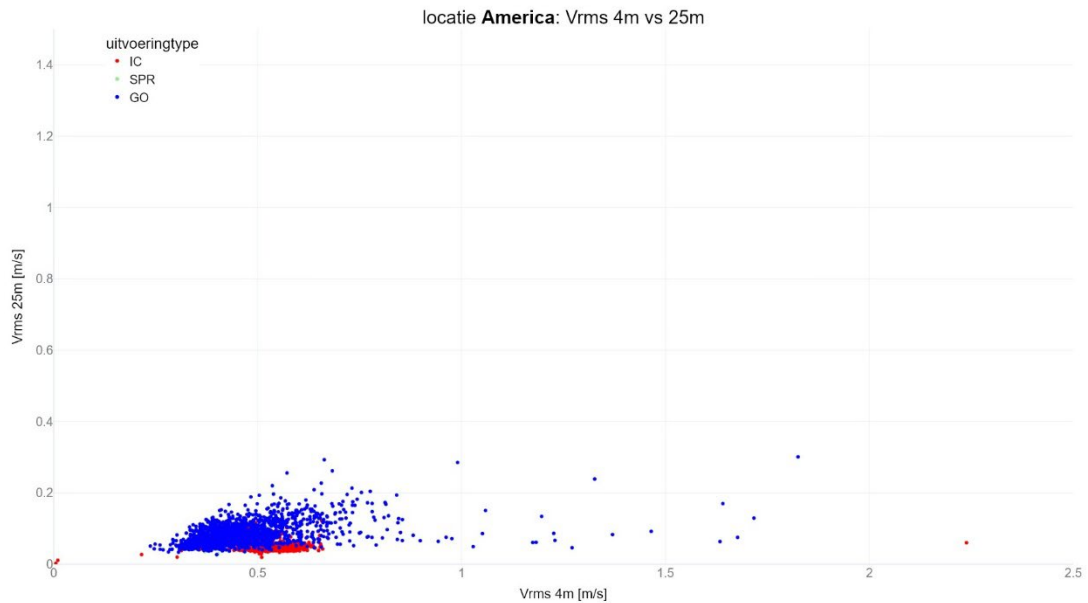
figuur 46 Verband tussen V_{rms} waarden op 4m en 25m per uitvoeringstype
