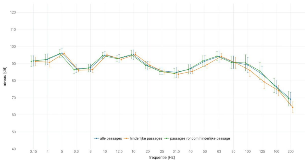
locatie Schalkwijk : gemiddeld spectrum passage met IC op spoor 2 meetlocatie: oost 4m C | meetrichting: Y | foutbalk met +/- standaard afwijking
