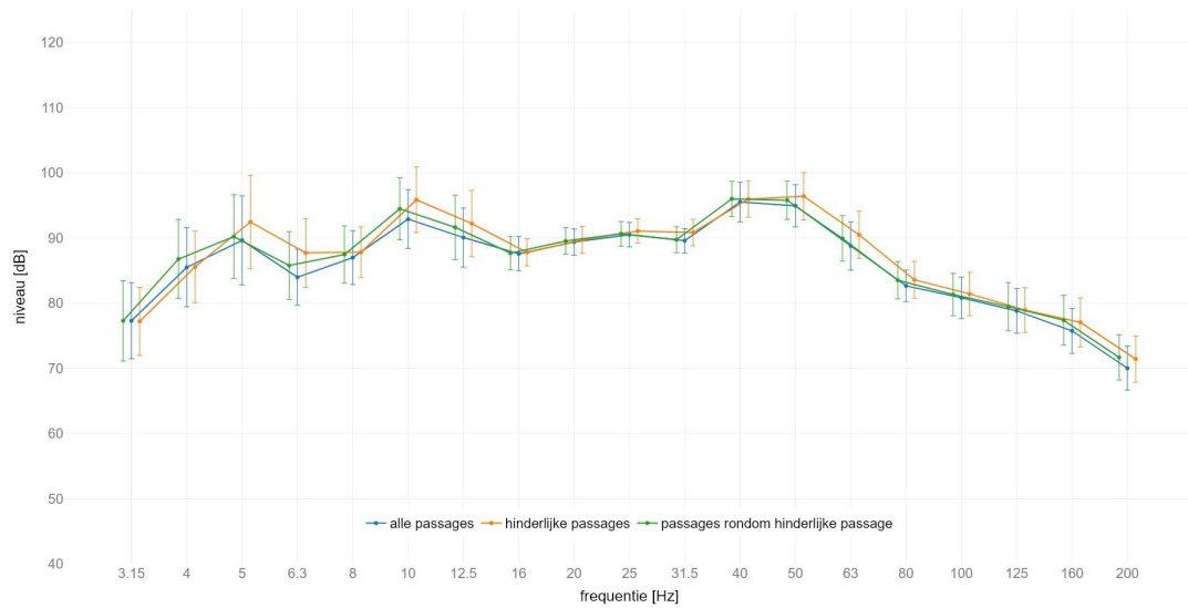
locatie Holten : gemiddeld spectrum passage met GO op spoor 2 meetlocatie: zuid 25m C | meetrichting: X | voetbalk met +/- standaard afwijking
