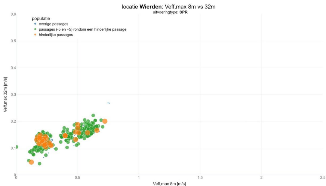
figuur 106 Verband tussen V_{eff,max} waarden voor sprinters op 8m en 32m en relatie met hinder
