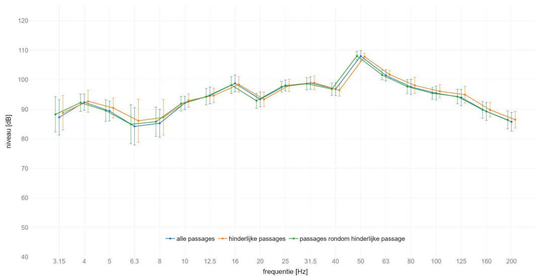
locatie Holten : gemiddeld spectrum passage met IC op spoor 1 meetlocatie: noord 4m C | meetrichting: Y | voetbalk met +/- standaard afwijking
