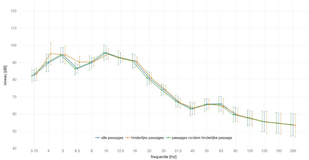
locatie Schalkwijk : gemiddeld spectrum passage met IC op spoor 1 meetlocatie: west 25m C | meetrichting: Z | foutbalk met +/- standaard afwijking
