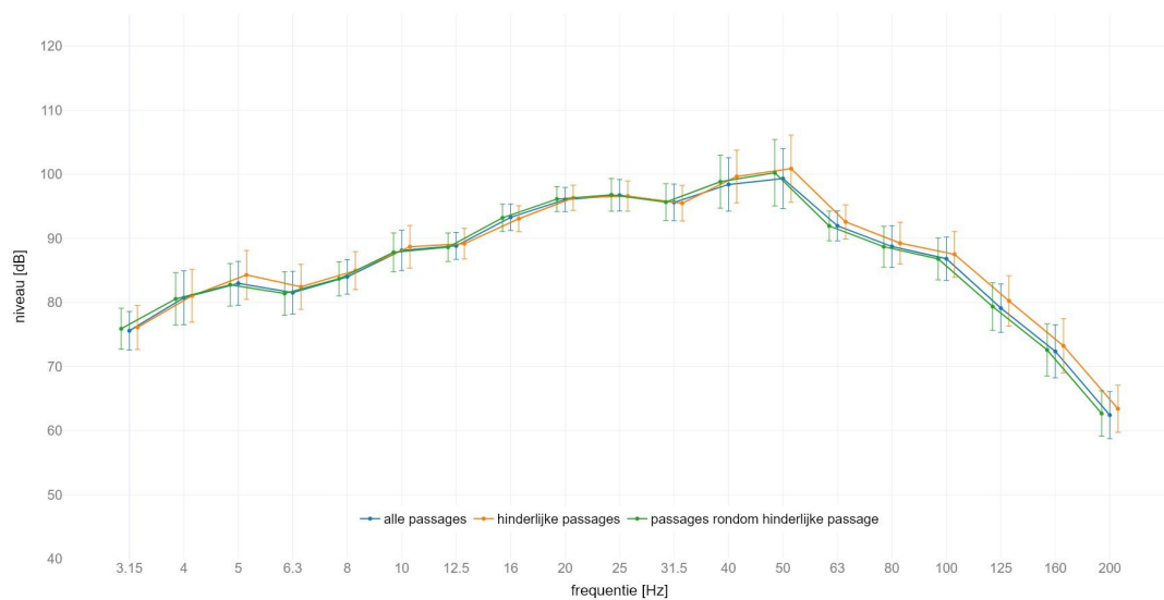
locatie America : gemiddeld spectrum passage met GO op spoor 2 meetlocatie: zuid 8m C | meetrichting: Y | foutbalk met +/- standaard afwijking
