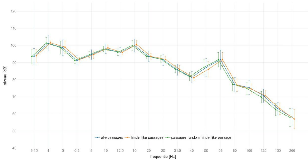
locatie Schalkwijk : gemiddeld spectrum passage met IC op spoor 2 meetlocatie: west 8m C | meetrichting: Z | foutbalk met +/- standaard afwijking
