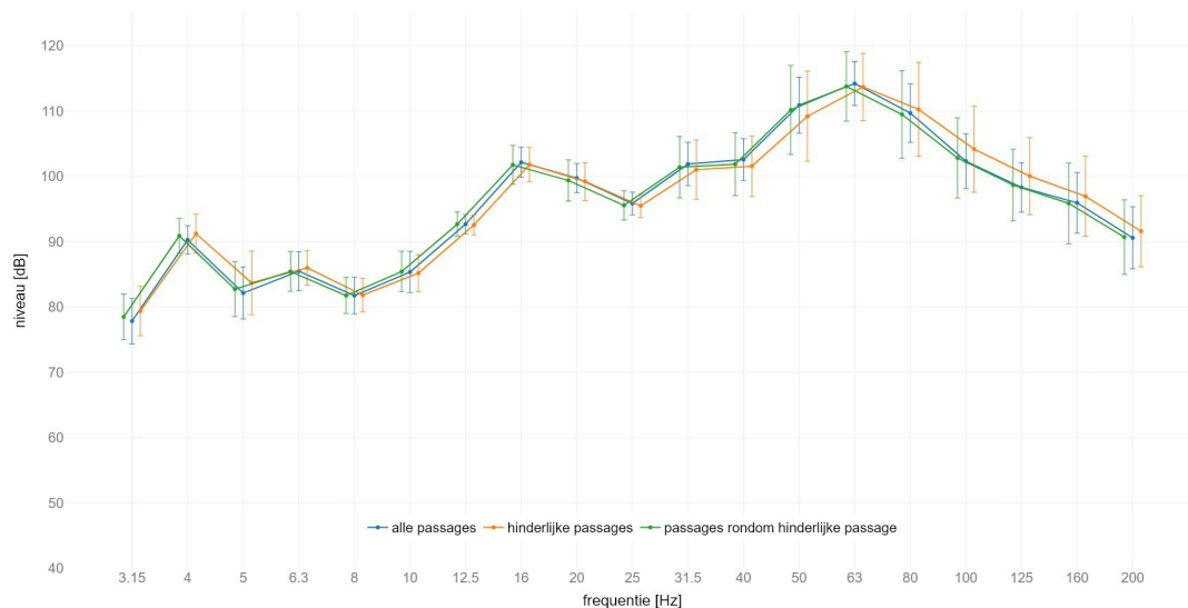
locatie America : gemiddeld spectrum passage met IC op spoor 1 meetlocatie: noord 4m C | meetrichting: Z | foutbalk met +/- standaard afwijking
