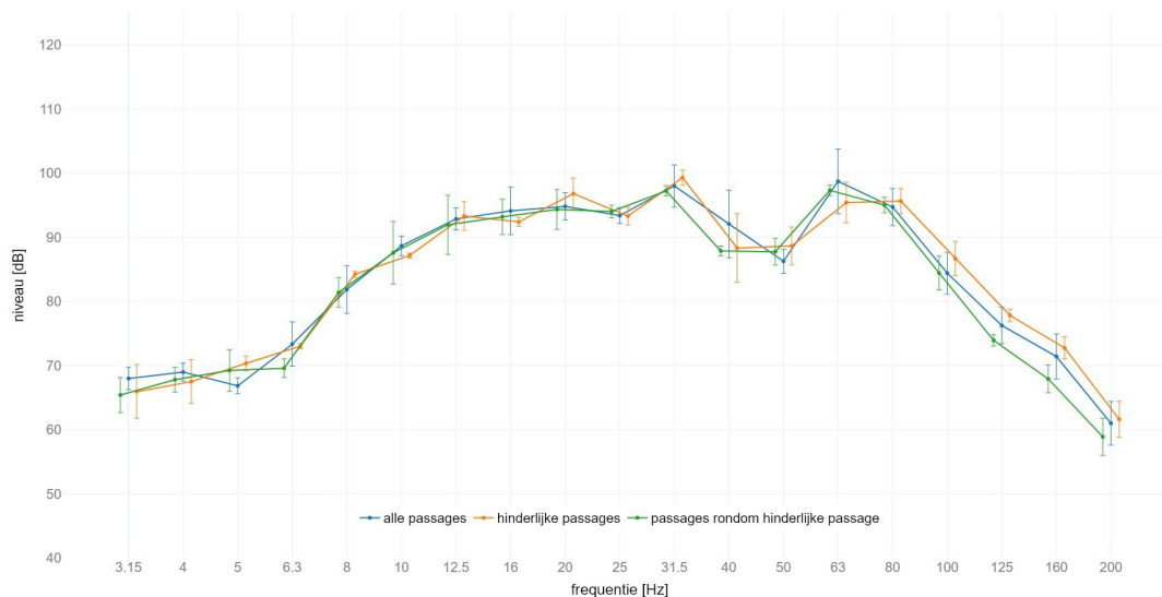
locatie America : gemiddeld spectrum passage met SPR op spoor 2 meetlocatie: zuid 8m C | meetrichting: Y | foutbalk met +/- standaard afwijking
