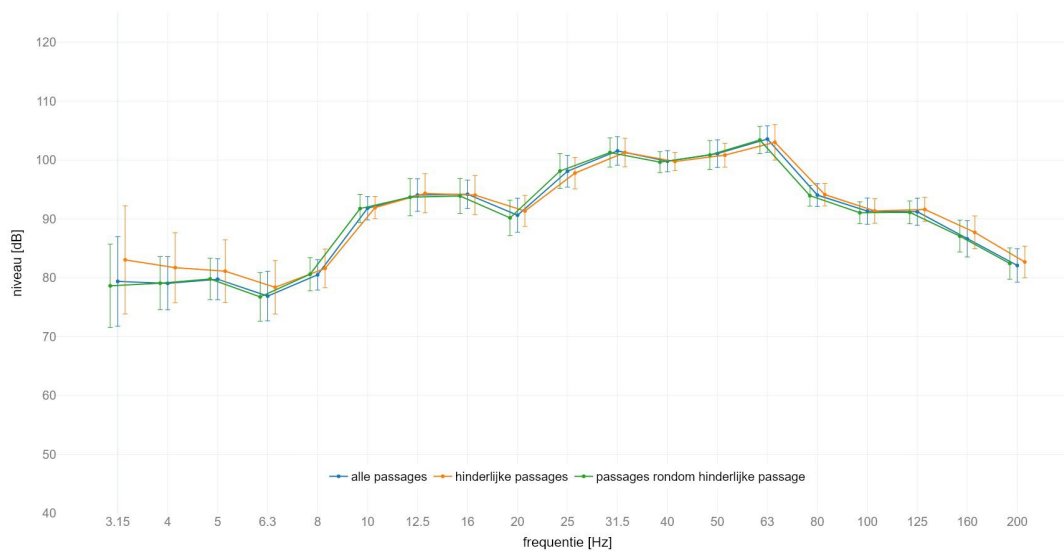
locatie Holten : gemiddeld spectrum passage met IC op spoor 2 meetlocatie: noord 4m C | meetrichting: X | voetbalk met +/- standaard afwijking
