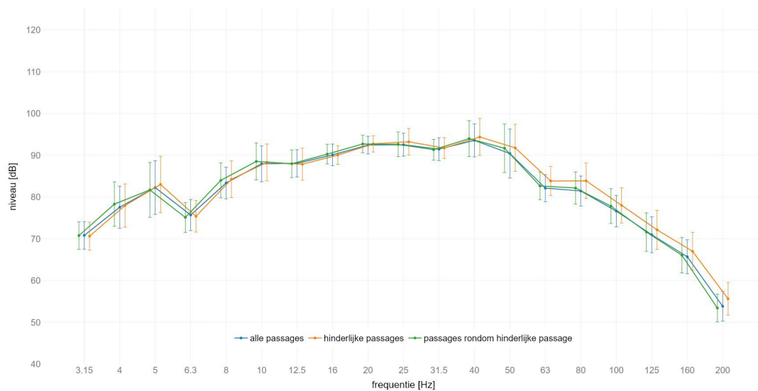
locatie America : gemiddeld spectrum passage met GO op spoor 1 meetlocatie: zuid 8m C | meetrichting: X | voetbalk met +/- standaard afwijking
