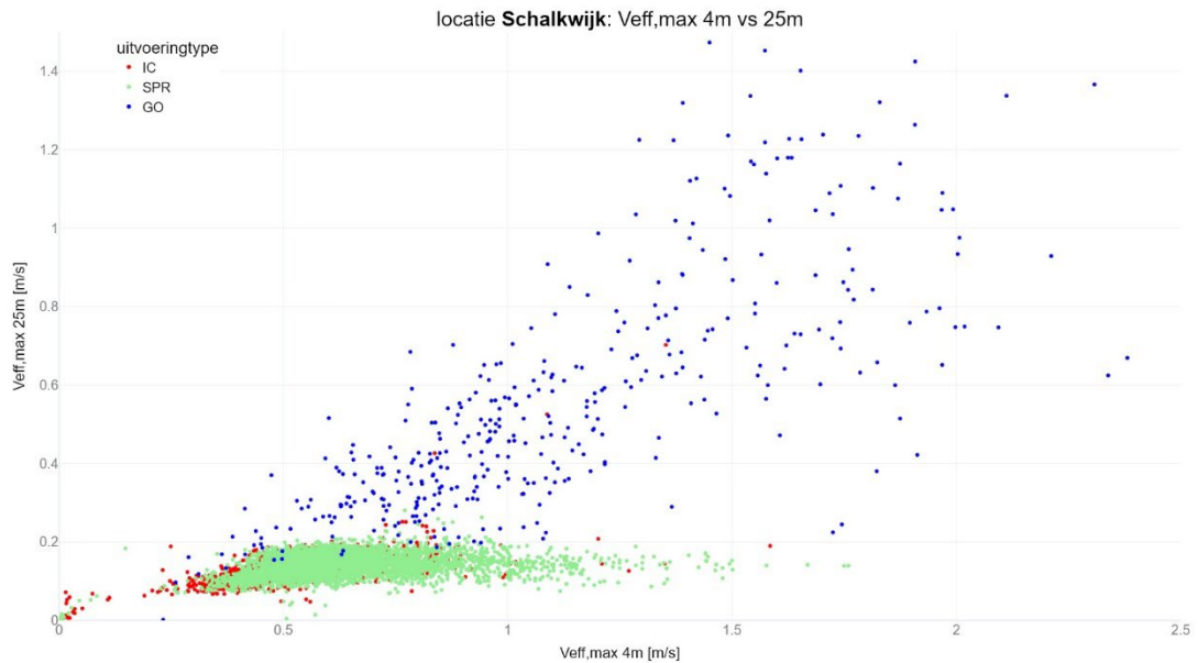
figuur 17 Verband tussen V_{eff,max} waardes op 4m en 25m
