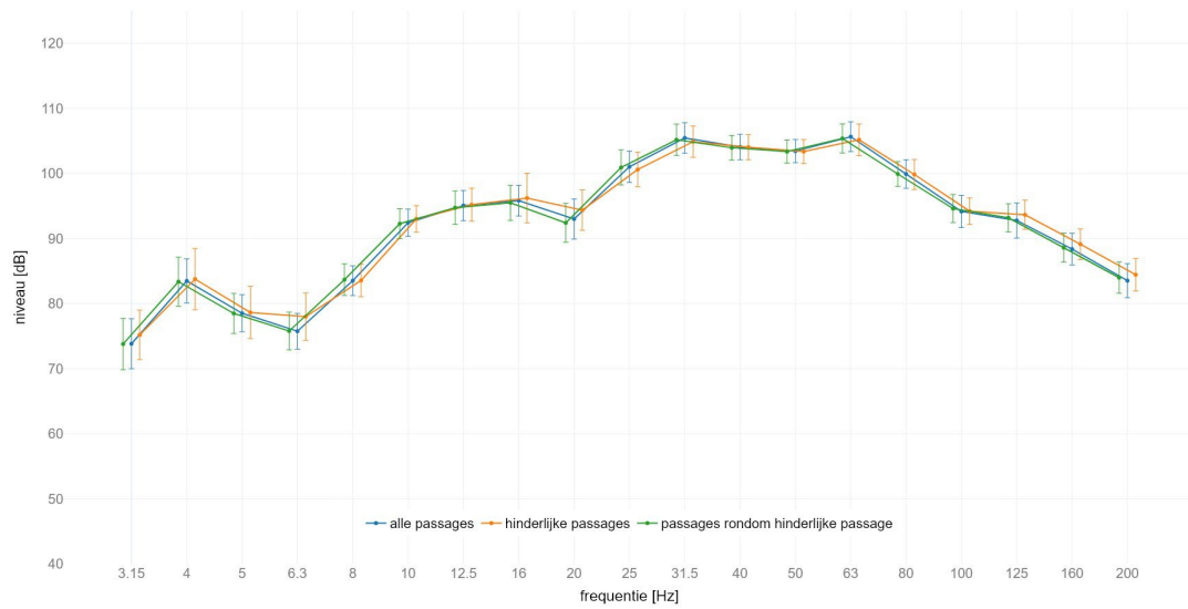
locatie Holten : gemiddeld spectrum passage met IC op spoor 2 meetlocatie: noord 4m C | meetrichting: Z | foutebalk met +/- standaard afwijking
