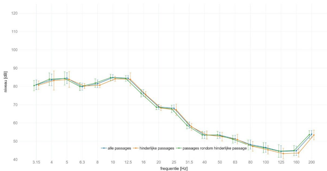
locatie Schalkwijk : gemiddeld spectrum passage met SPR op spoor 2 meetlocatie: gebouw | meetrichting: Z | foutbalk met +/- standaard afwijking
