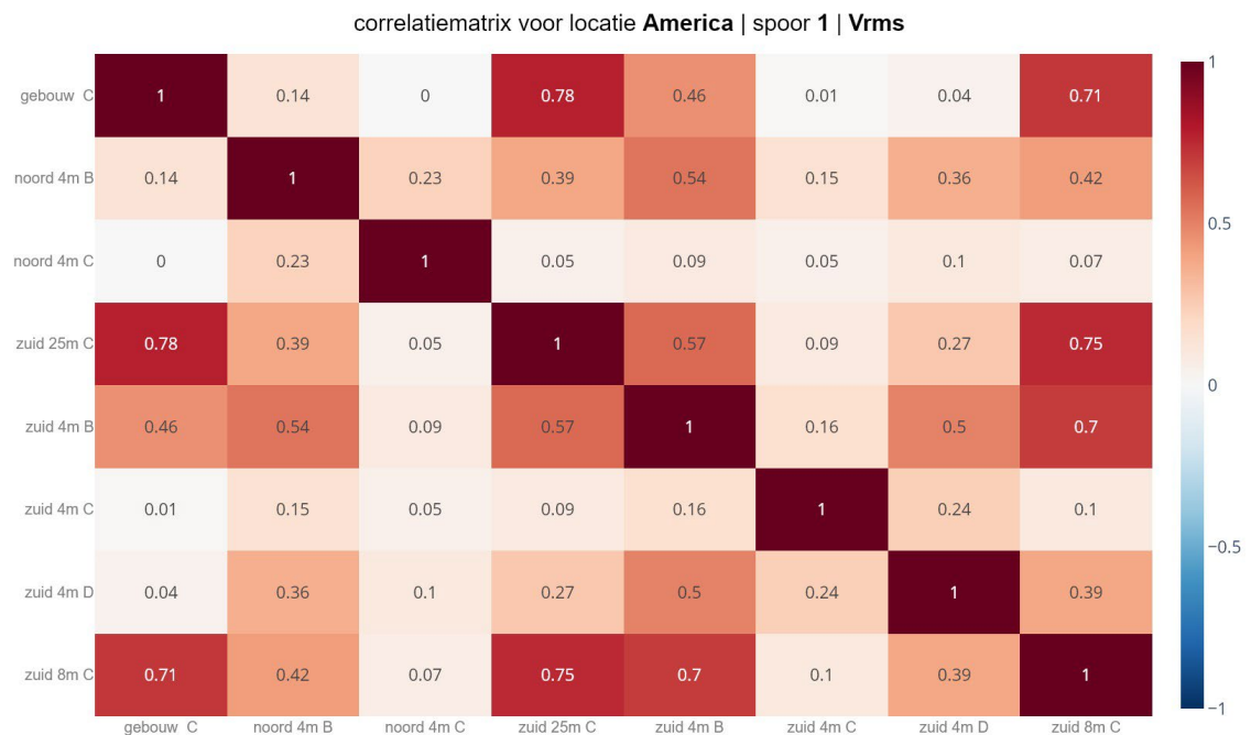
figuur 44 Correlatie matrix V_{rms} voor passage op spoor 1
