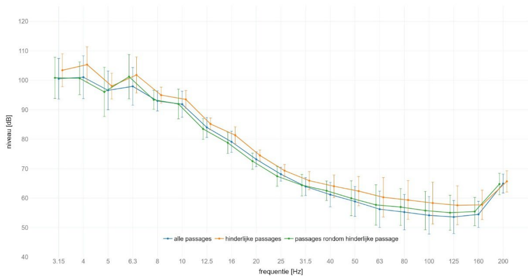
locatie Schalkwijk : gemiddeld spectrum passage met GO op spoor 2 meetlocatie: gebouw | meetrichting: X | foutbalk met +/- standaard afwijking
