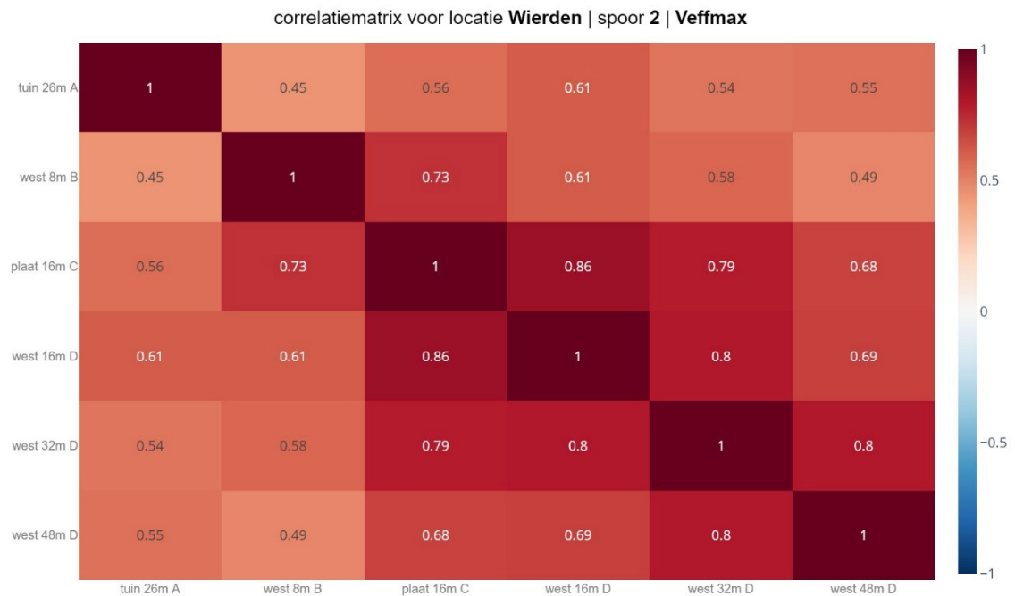
figuur 101 Correlatie matrix V_{eff,max} voor passage op spoor 2
