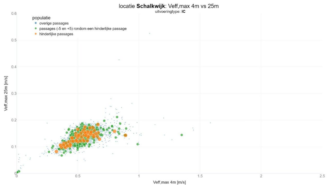
figuur 119 Verband tussen V_{eff,max} waarden op 4m en 25m voor intercity's en relatie met hinder
