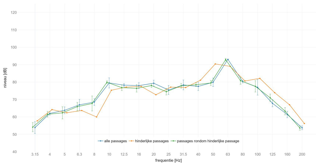
locatie America : gemiddeld spectrum passage met SPR op spoor 1 meetlocatie: zuid 25m C | meetrichting: Y | foutbalk met +/- standaard afwijking
