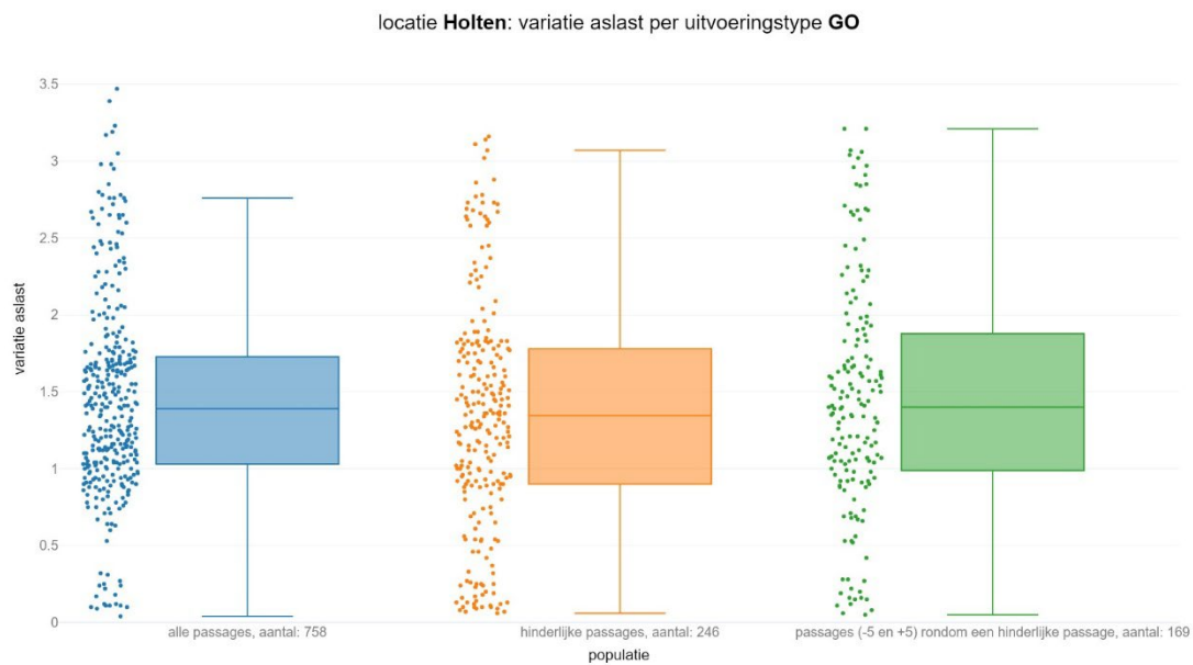
figuur 133 Variatie aslast voor goederentreinen per populatie
