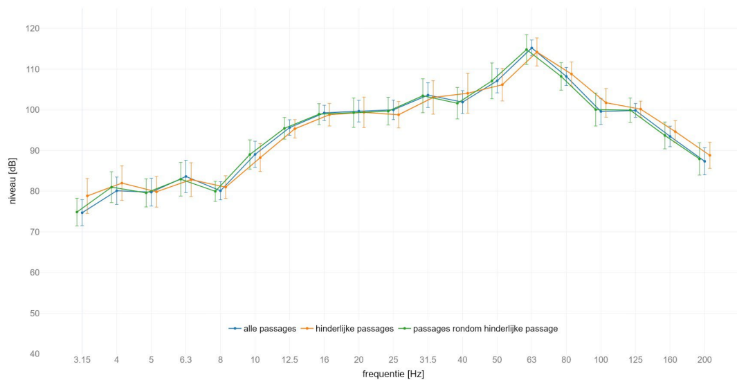
locatie America : gemiddeld spectrum passage met IC op spoor 2 meetlocatie: zuid 4m C | meetrichting: Z | foutbalk met +/- standaard afwijking
