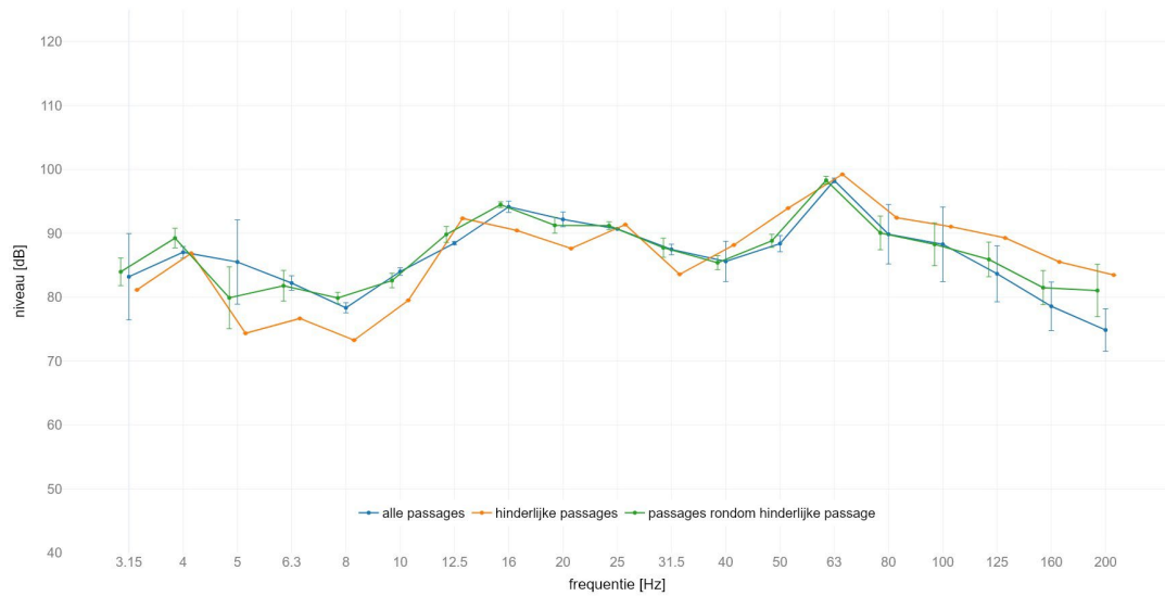
locatie America : gemiddeld spectrum passage met SPR op spoor 1 meetlocatie: noord 4m C | meetrichting: Y | foutbalk met +/- standaard afwijking
