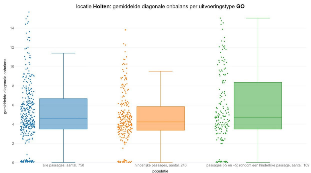
figuur 68 Gemiddelde diagonale onbalans voor goederentreinen per populatie
