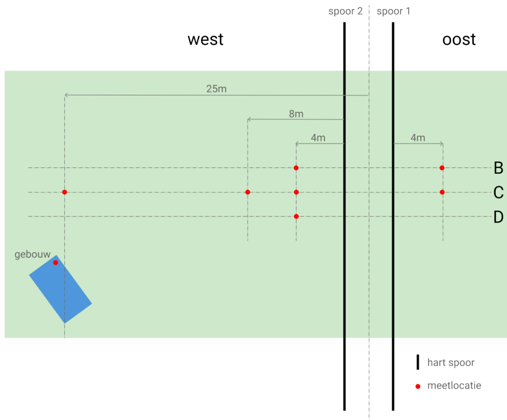
figuur 1 Meetlocaties op onderzoekslocatie Schalkwijk
