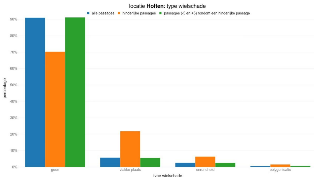
figuur 65 Type wielschade per populatie
