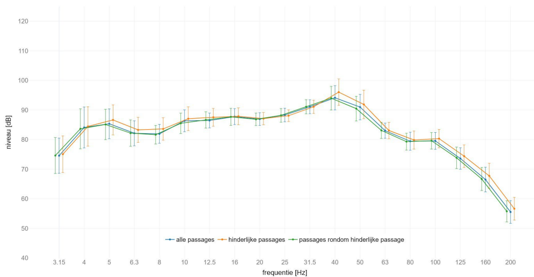
locatie America : gemiddeld spectrum passage met GO op spoor 2 meetlocatie: zuid 25m C | meetrichting: X | voetbalk met +/- standaard afwijking
