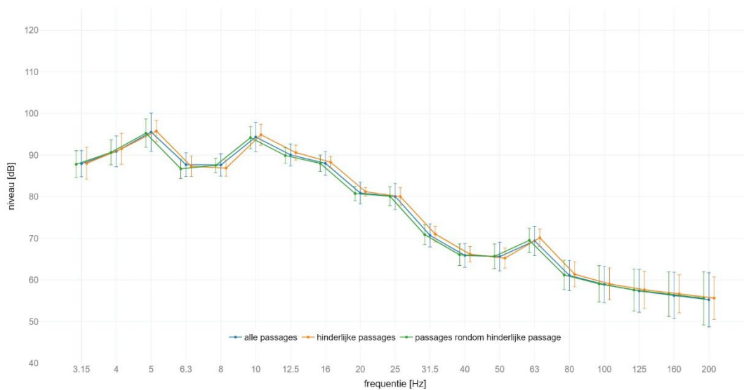
locatie Schalkwijk : gemiddeld spectrum passage met IC op spoor 2 meetlocatie: west 25m C | meetrichting: Y | voetbalk met +/- standaard afwijking
