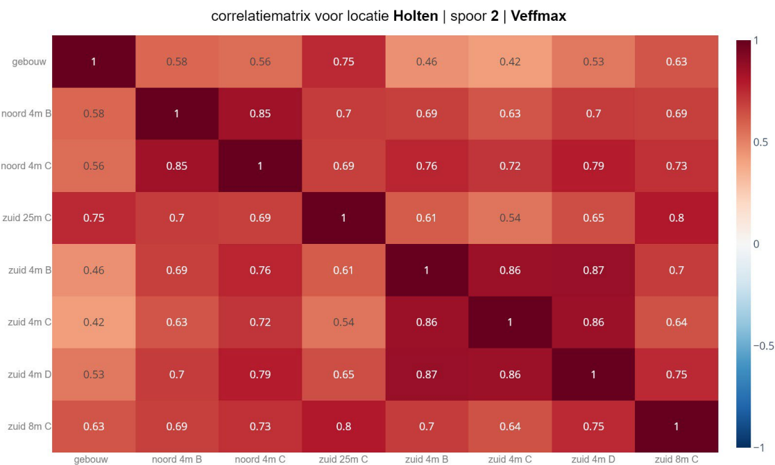
figuur 140 Correlatie matrix V_{eff,max} spoor 2
