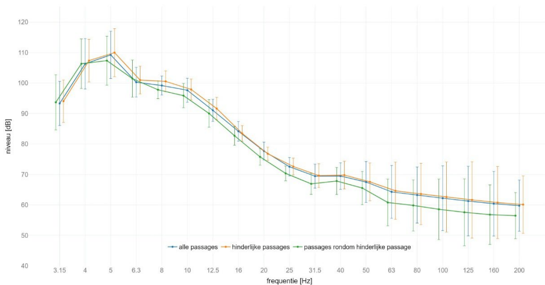
locatie Schalkwijk : gemiddeld spectrum passage met GO op spoor 1 meetlocatie: oost 4m C | meetrichting: Y | foute balk met +/- standaard afwijking
