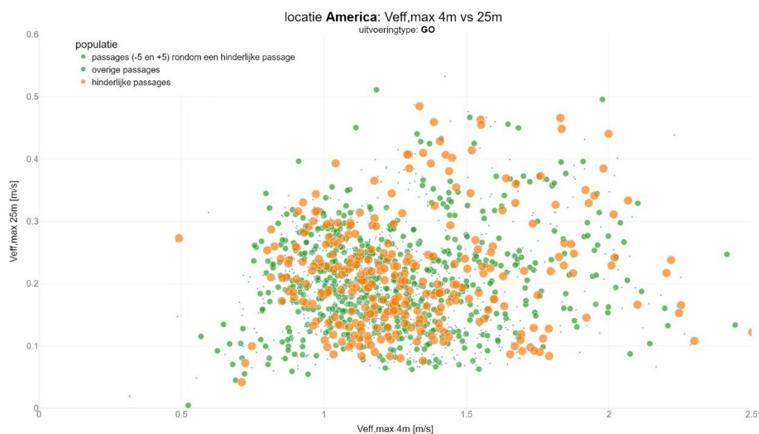
figuur 129 Verband tussen V_{eff,max} waardes op 4m en 25m voor goederentreinen en relatie met hinder
