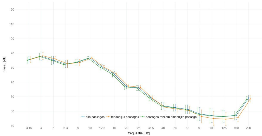
locatie Schalkwijk : gemiddeld spectrum passage met IC op spoor 2 meetlocatie: gebouw | meetrichting: Y | foutbalk met +/- standaard afwijking
