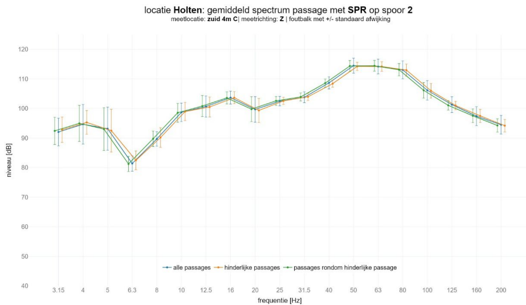
figuur 85 Gemiddeld spectrum 4m zuid, Z richting voor sprinters
