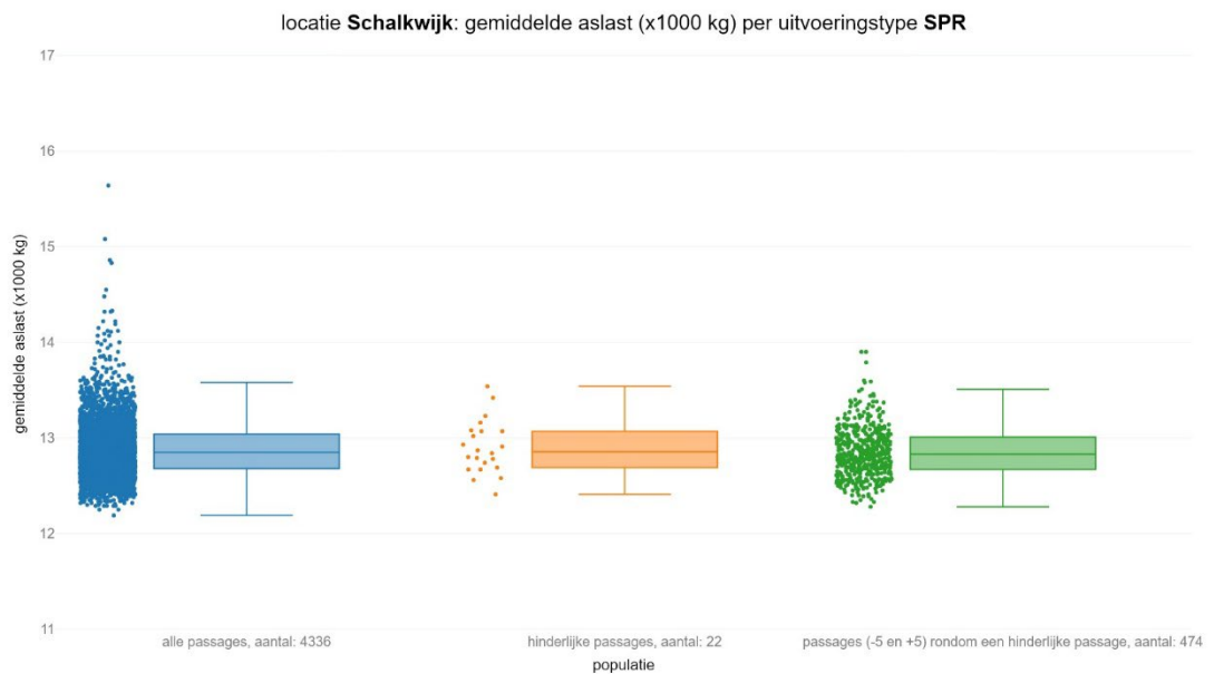
figuur 108 Gemiddelde aslast voor sprinters per populatie
