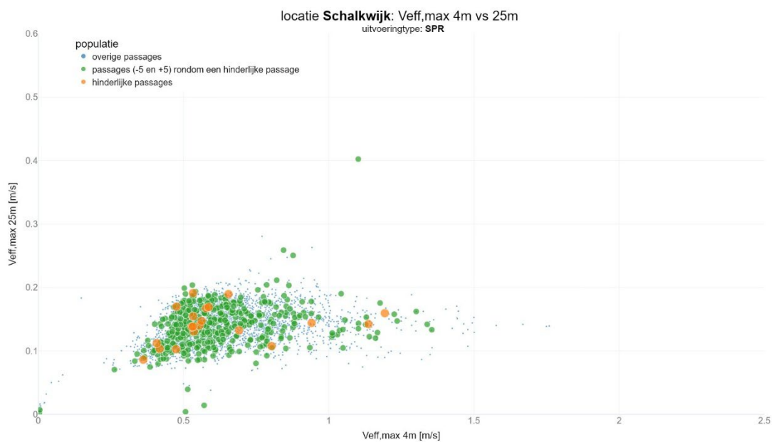
figuur 121 Verband tussen V_{eff,max} waarden op 4m en 25m voor sprinters en verband met hinder
