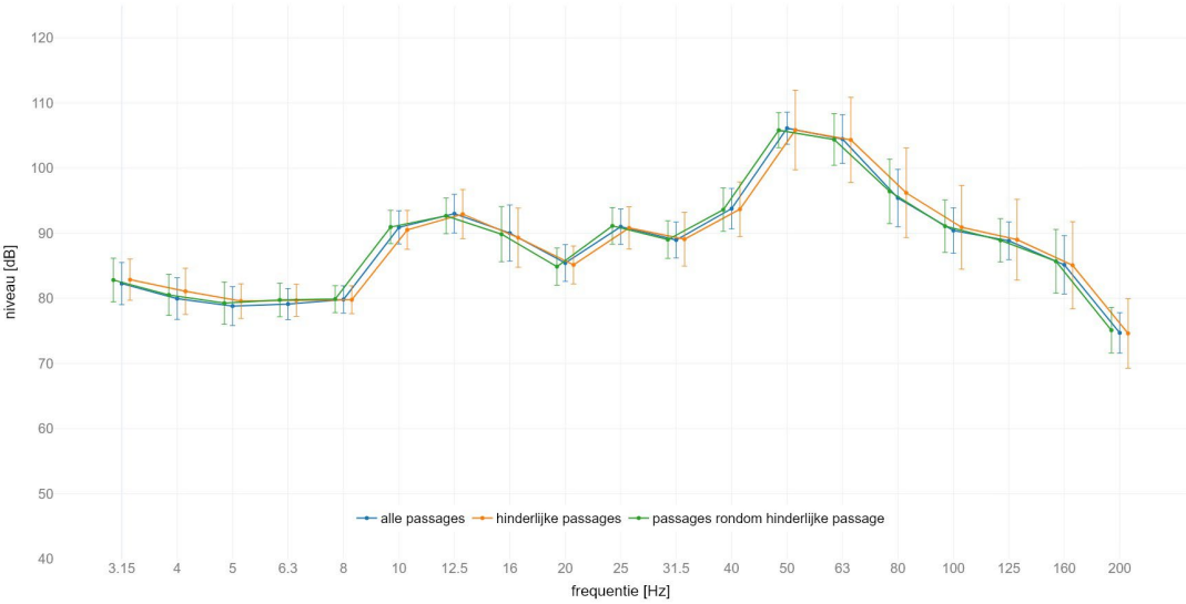
locatie Holten : gemiddeld spectrum passage met SPR op spoor 1 meetlocatie: zuid 4m C | meetrichting: Y | foutbalk met +/- standaard afwijking
