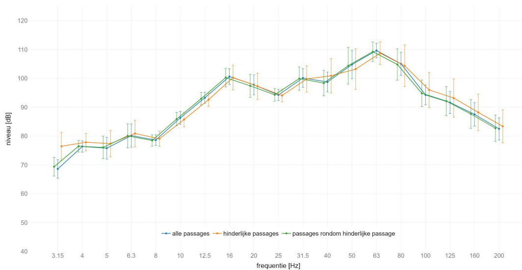
locatie America : gemiddeld spectrum passage met IC op spoor 2 meetlocatie: noord 4m C | meetrichting: Y | foutbalk met +/- standaard afwijking
