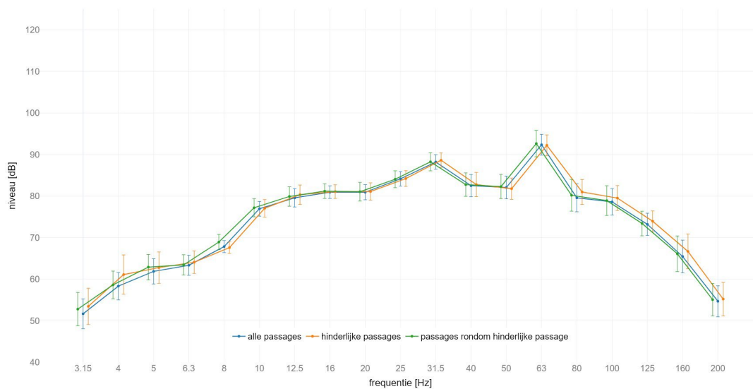
locatie America : gemiddeld spectrum passage met IC op spoor 1 meetlocatie: zuid 25m C | meetrichting: X | foutelek met +/- standaard afwijking
