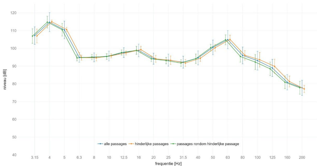
locatie Schalkwijk : gemiddeld spectrum passage met IC op spoor 2 meetlocatie: west 8m C | meetrichting: X | foutbalk met +/- standaard afwijking
