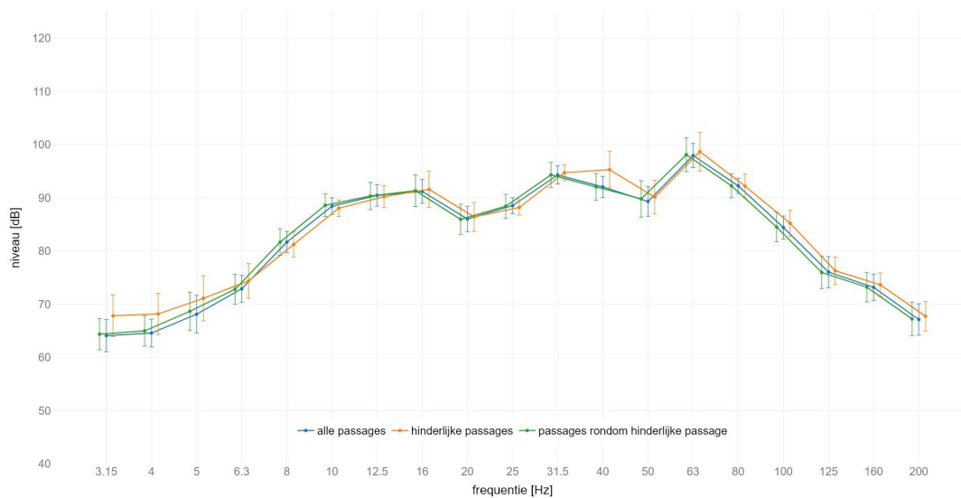
locatie America : gemiddeld spectrum passage met IC op spoor 2 meetlocatie: zuid 8m C | meetrichting: Z | foutbalk met +/- standaard afwijking
