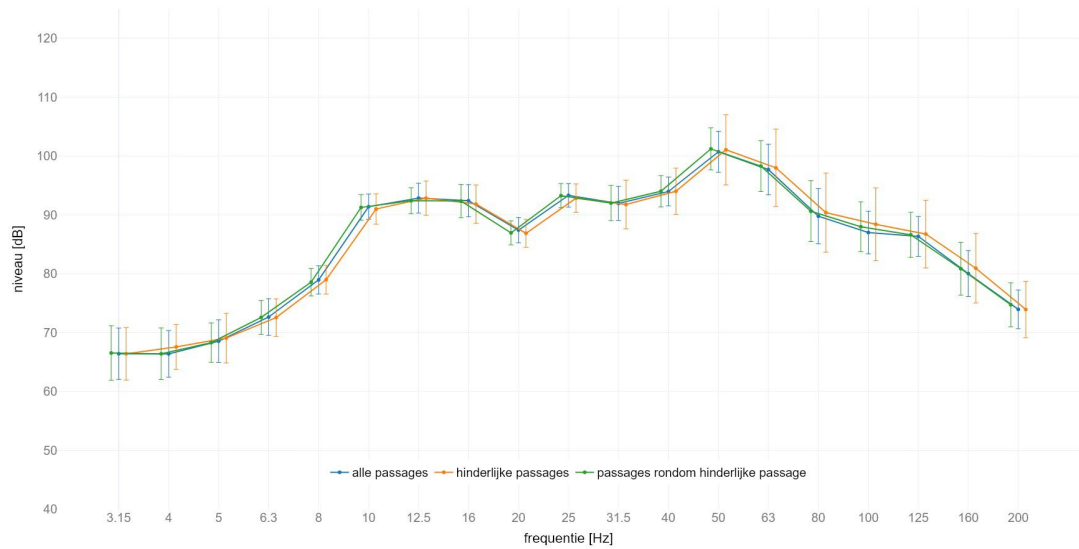
locatie Holten : gemiddeld spectrum passage met SPR op spoor 1 meetlocatie: zuid 8m C | meetrichting: Z | foutbalk met +/- standaard afwijking
