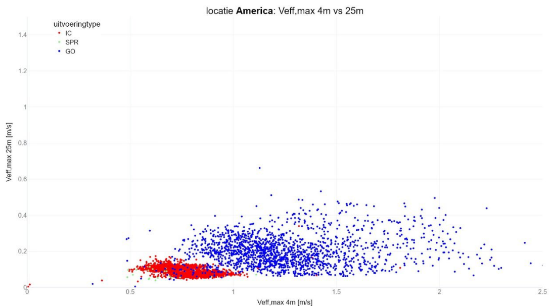
figuur 47 America: verband tussen V_{eff,max} waarden op 4m en 25m per uitvoeringstype
