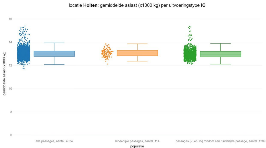
figuur 131 Gemiddelde aslast voor intercity's per populatie
