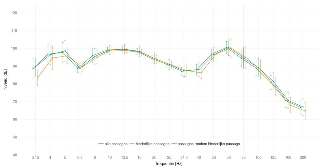
locatie Schalkwijk : gemiddeld spectrum passage met SPR op spoor 1 meetlocatie: west 8m C | meetrichting: X | foutbalk met +/- standaard afwijking
