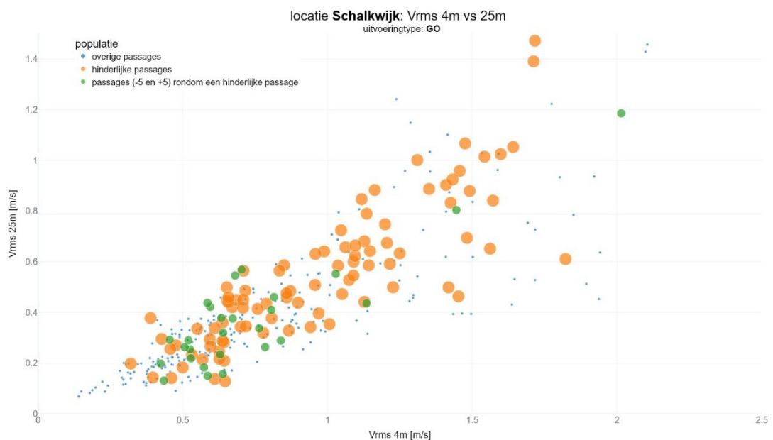
figuur 18 Verband tussen V_{rms} waardes voor goederentreinen op 4m en 25m en relatie met hinder
