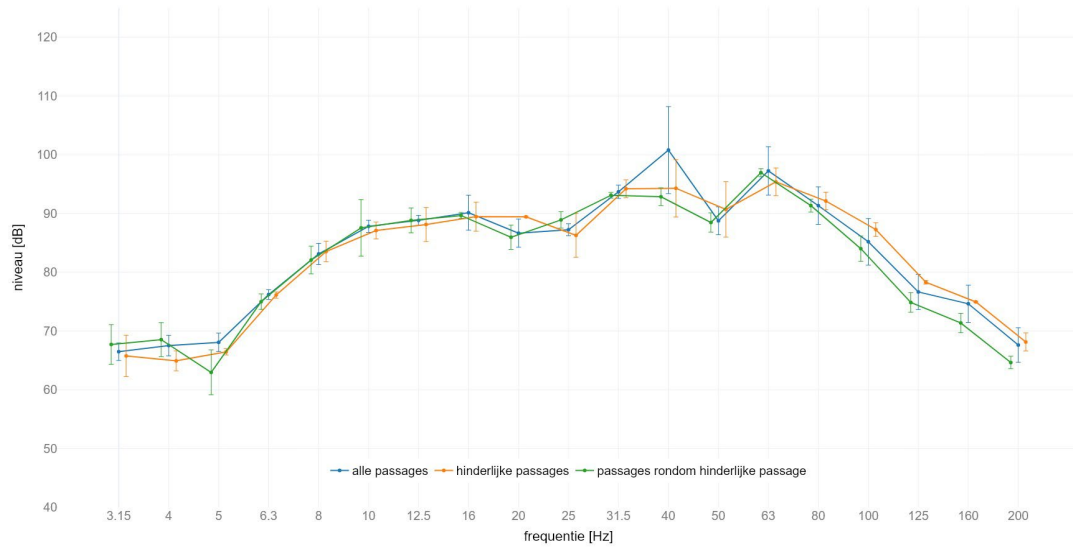
locatie America : gemiddeld spectrum passage met SPR op spoor 2 meetlocatie: zuid 25m C | meetrichting: X | foutbalk met +/- standaard afwijking
