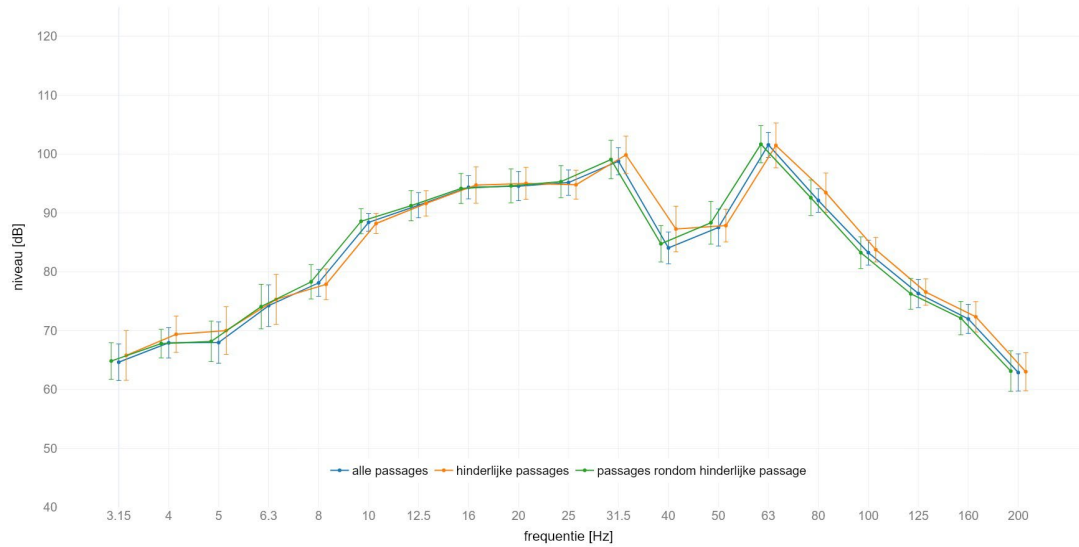
locatie America : gemiddeld spectrum passage met IC op spoor 2 meetlocatie: zuid 8m C | meetrichting: X | foutbalk met +/- standaard afwijking
