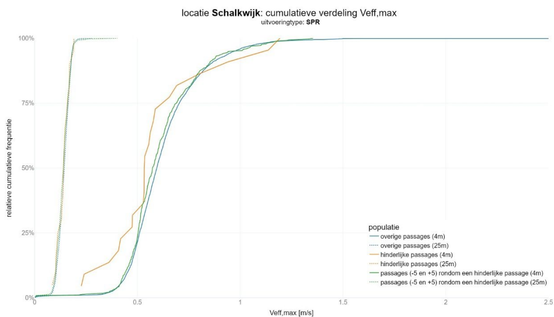
figuur 122 Cumulatieve verdeling van V_{eff,max} waarden voor sprinters
