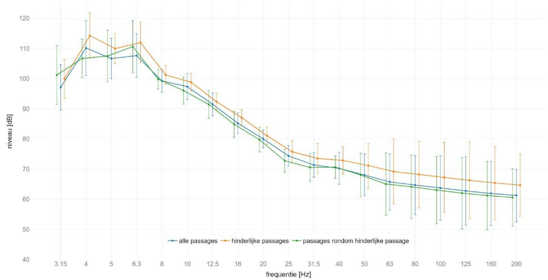
locatie Schalkwijk : gemiddeld spectrum passage met GO op spoor 2 meetlocatie: gebouw | meetrichting: Z | foutbalk met +/- standaard afwijking
