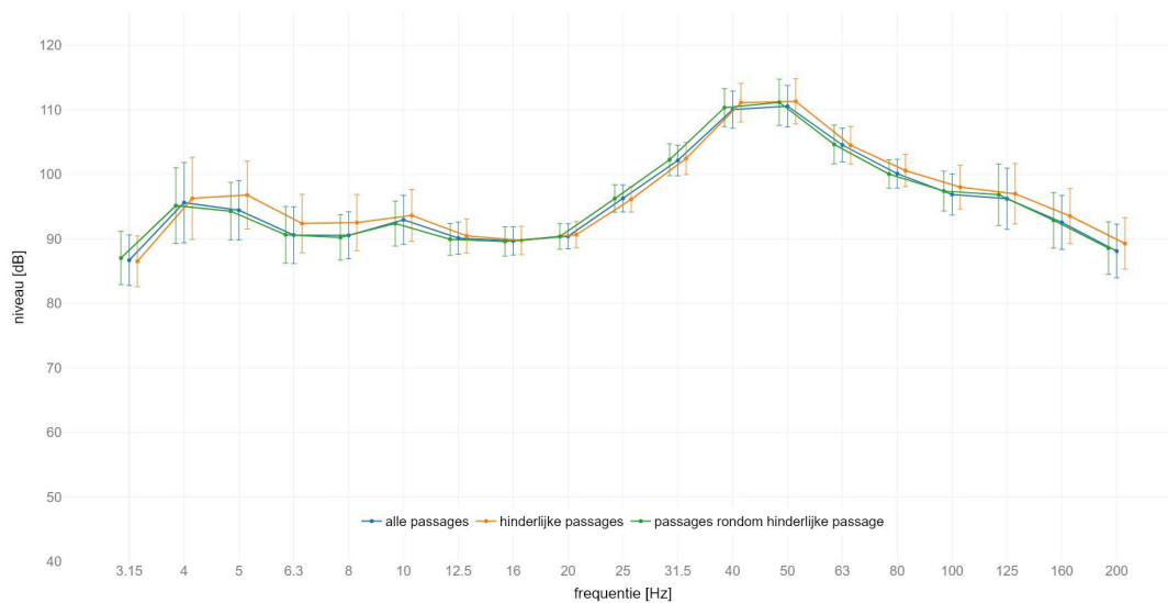
locatie America : gemiddeld spectrum passage met GO op spoor 2 meetlocatie: zuid 4m D | meetrichting: Z | voetbalk met +/- standaard afwijking
