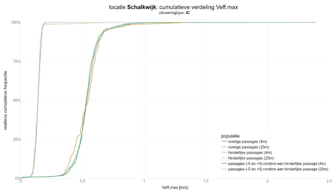
figuur 120 Cumulatieve verdeling van V_{eff,max} waarden voor intercity's
