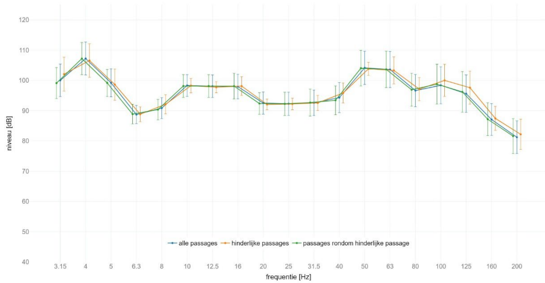
locatie Schalkwijk : gemiddeld spectrum passage met IC op spoor 1 meetlocatie: oost 4m C | meetrichting: Z | foutelek met +/- standaard afwijking
