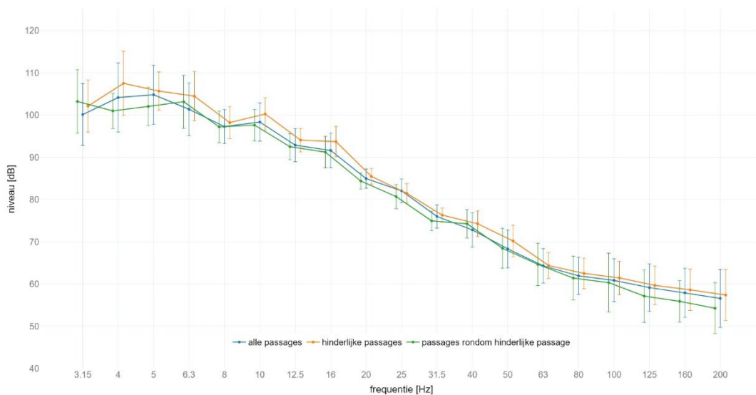
locatie Schalkwijk : gemiddeld spectrum passage met GO op spoor 2 meetlocatie: west 25m C | meetrichting: Z | voetbalk met +/- standaard afwijking
