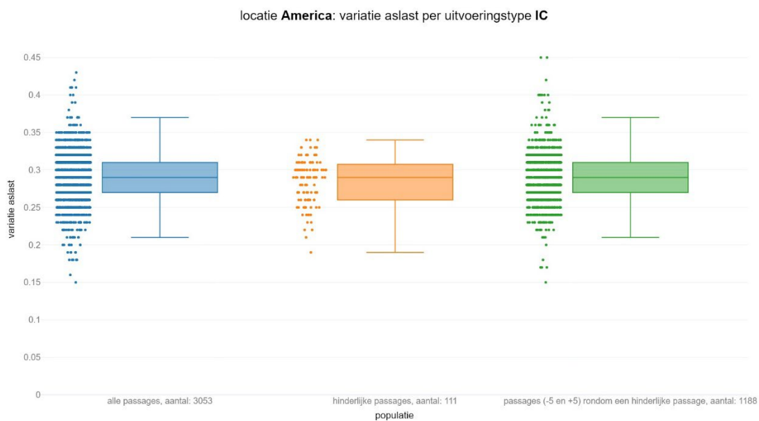
figuur 124 Variatie aslast voor intercity's per populatie
