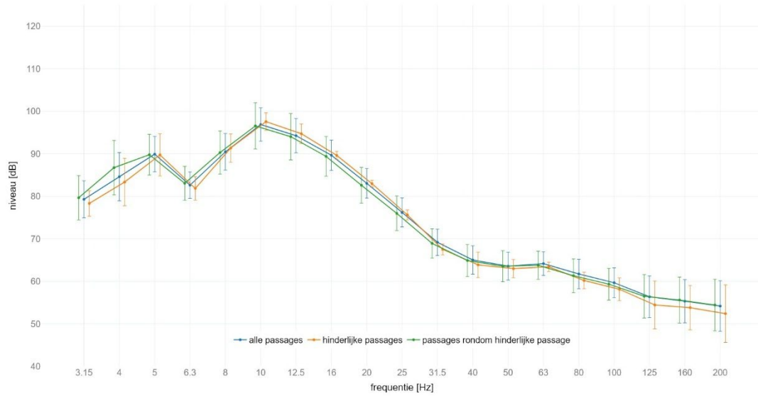
locatie Schalkwijk : gemiddeld spectrum passage met SPR op spoor 2 meetlocatie: west 25m C | meetrichting: Z | voetbalk met +/- standaard afwijking
