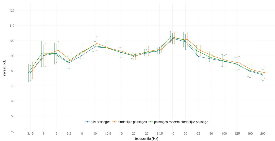
locatie Holten : gemiddeld spectrum passage met GO op spoor 1 meetlocatie: zuid 8m C | meetrichting: Z | foutbalk met +/- standaard afwijking
