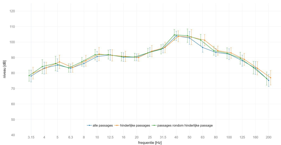
locatie Holten : gemiddeld spectrum passage met GO op spoor 1 meetlocatie: zuid 4m C | meetrichting: Y | voetbalk met +/- standaard afwijking
