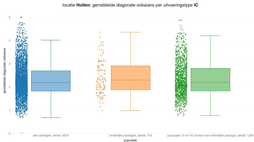
figuur 135 Gemiddelde diagonale onbalans voor intercity's per populatie
