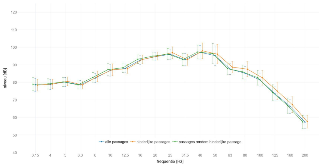
locatie America : gemiddeld spectrum passage met GO op spoor 1 meetlocatie: zuid 8m C | meetrichting: Z | foutbalk met +/- standaard afwijking
