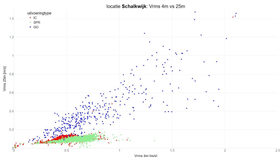
figuur 16 Verband tussen V_{rms} waarden op 4m en 25m
