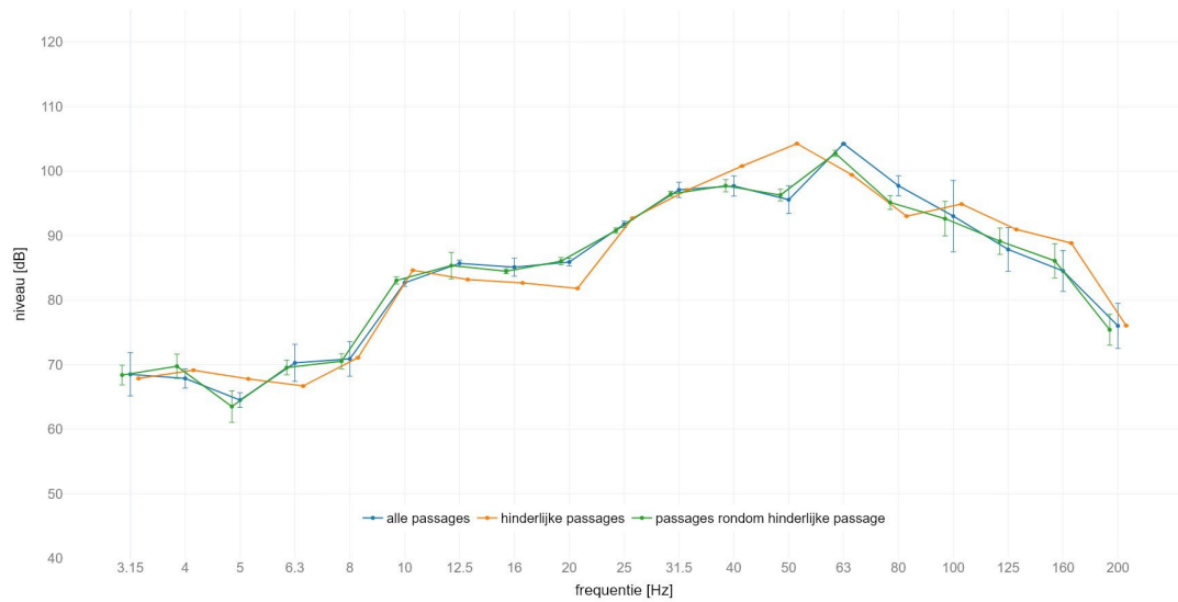
locatie America : gemiddeld spectrum passage met SPR op spoor 1 meetlocatie: zuid 4m C | meetrichting: Z | foutbalk met +/- standaard afwijking
