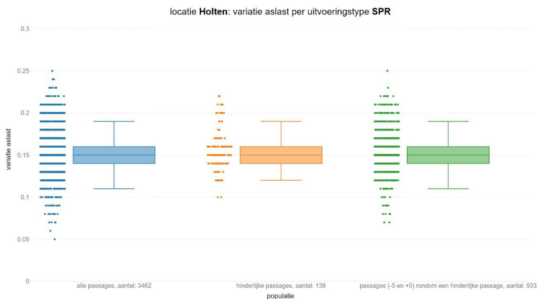
figuur 134 Variatie aslast voor sprinters per populatie
