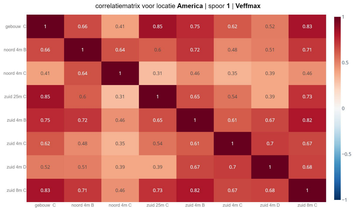
figuur 127 Correlatie matrix V_{eff,max} spoor 1
