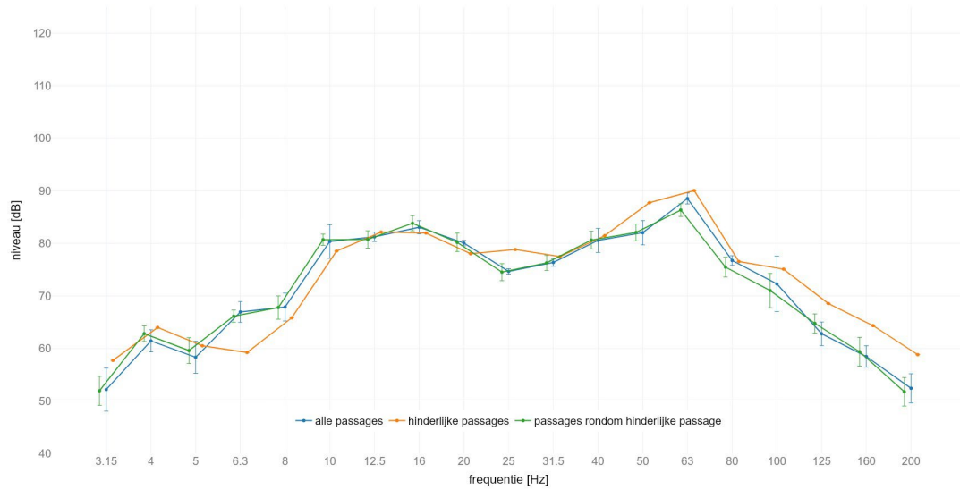
locatie America : gemiddeld spectrum passage met GO op spoor 2 meetlocatie: noord 4m B | meetrichting: Z | foutbalk met +/- standaard afwijking
