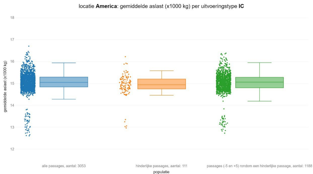
figuur 123 Gemiddelde aslast voor intercity's per populatie
