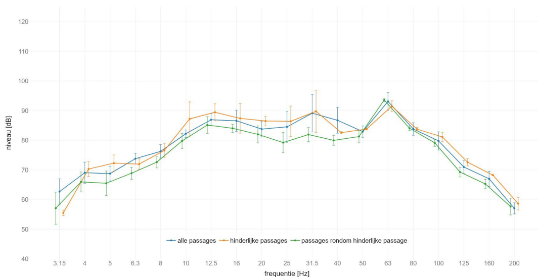
locatie America : gemiddeld spectrum passage met SPR op spoor 2 meetlocatie: zuid 25m C | meetrichting: Z | foutbalk met +/- standaard afwijking
