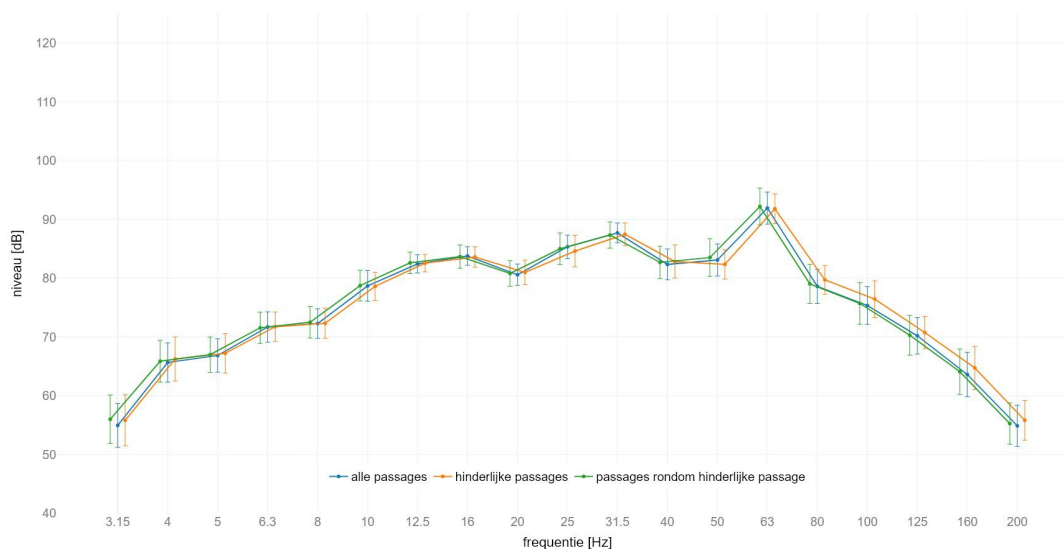
locatie America : gemiddeld spectrum passage met IC op spoor 1 meetlocatie: zuid 25m C | meetrichting: Z | foutebalk met +/- standaard afwijking
