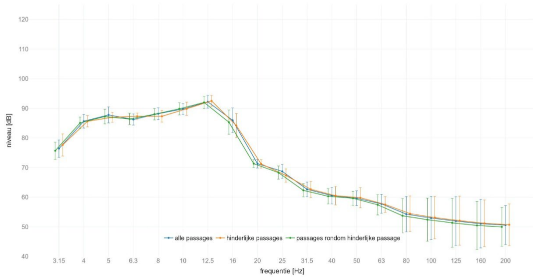
locatie Schalkwijk : gemiddeld spectrum passage met SPR op spoor 1 meetlocatie: oost 4m C | meetrichting: Y | foutbalk met +/- standaard afwijking
