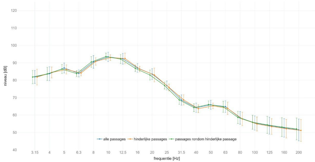
locatie Schalkwijk : gemiddeld spectrum passage met SPR op spoor 1 meetlocatie: west 25m C | meetrichting: Y | foutbalk met +/- standaard afwijking
