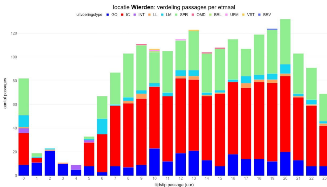
figuur 89 Verspreiding van passages van treinen over het etmaal
