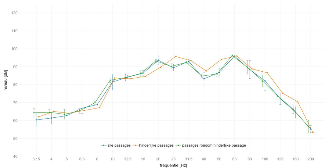
locatie America : gemiddeld spectrum passage met SPR op spoor 1 meetlocatie: zuid 8m C | meetrichting: X | foutbalk met +/- standaard afwijking
