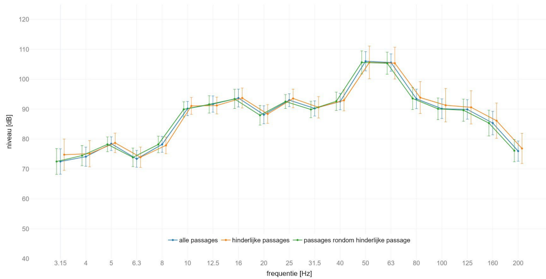
locatie Holten : gemiddeld spectrum passage met IC op spoor 1 meetlocatie: zuid 4m C | meetrichting: X | foutbalk met +/- standaard afwijking
