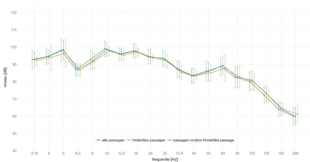
locatie Schalkwijk : gemiddeld spectrum passage met SPR op spoor 2 meetlocatie: west 8m C | meetrichting: Y | foutbalk met +/- standaard afwijking
