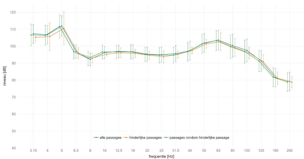
locatie Schalkwijk : gemiddeld spectrum passage met SPR op spoor 2 meetlocatie: west 4m C | meetrichting: Z | foutelek met +/- standaard afwijking
