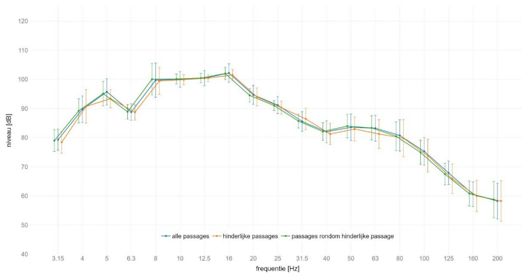
locatie Schalkwijk : gemiddeld spectrum passage met SPR op spoor 1 meetlocatie: west 8m C | meetrichting: Z | foutbalk met +/- standaard afwijking
