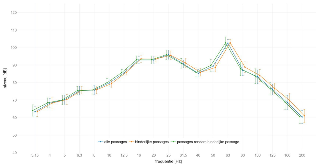
locatie America : gemiddeld spectrum passage met IC op spoor 1 meetlocatie: zuid 8m C | meetrichting: Y | foutbalk met +/- standaard afwijking
