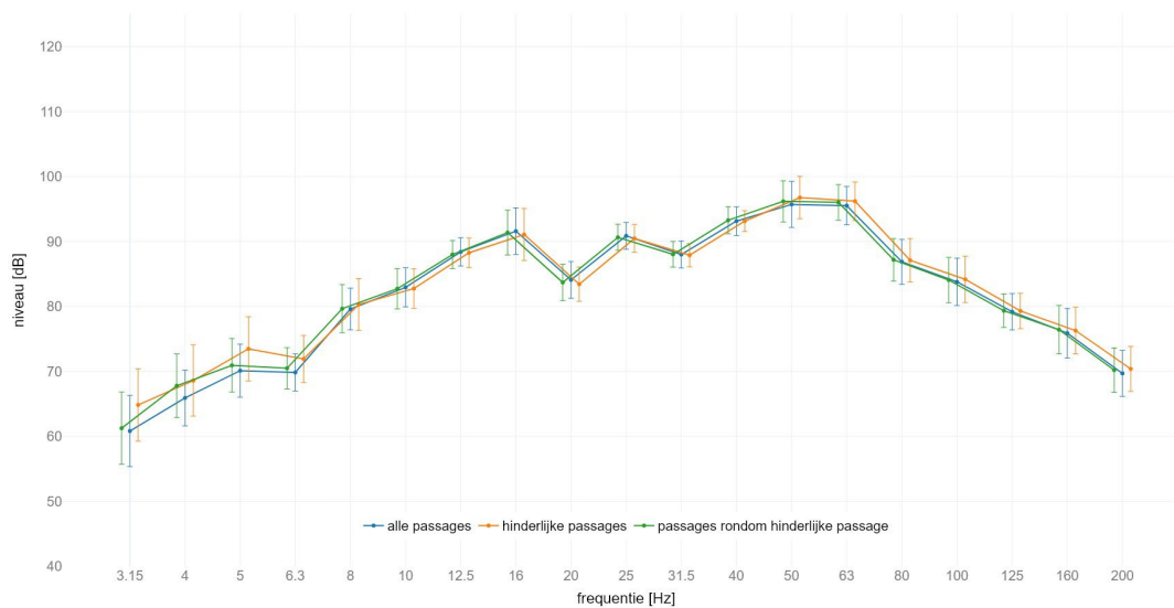
locatie Holten : gemiddeld spectrum passage met SPR op spoor 2 meetlocatie: zuid 25m C | meetrichting: X | voetbalk met +/- standaard afwijking
