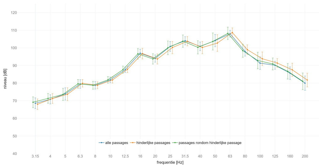
locatie America : gemiddeld spectrum passage met IC op spoor 1 meetlocatie: zuid 4m C | meetrichting: Y | foutbalk met +/- standaard afwijking
