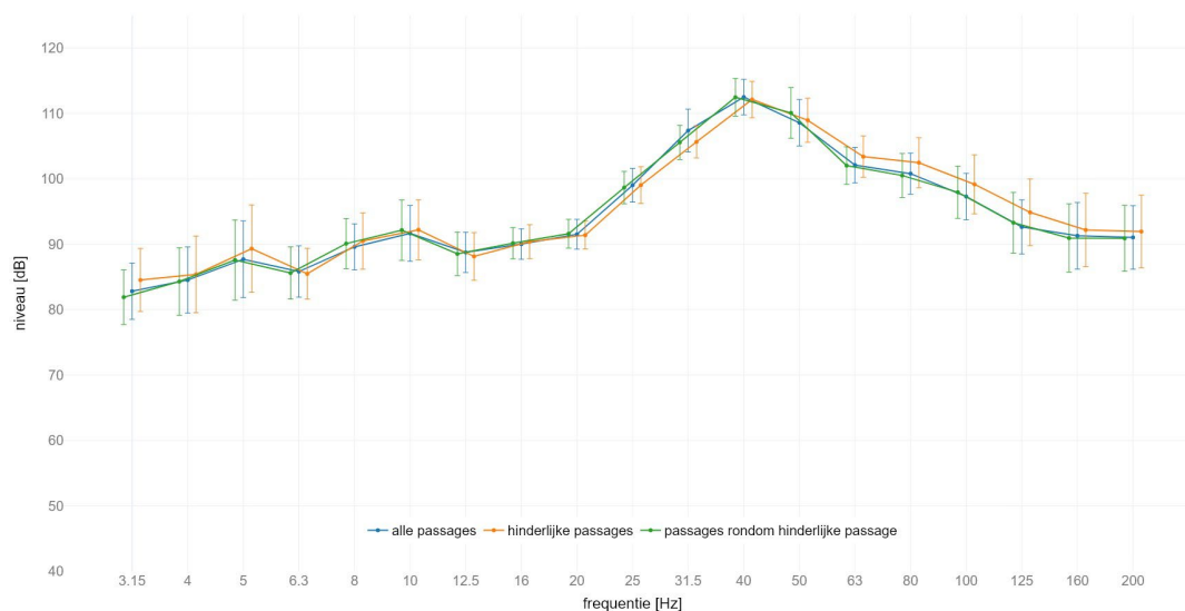
locatie America : gemiddeld spectrum passage met GO op spoor 1 meetlocatie: zuid 4m B | meetrichting: Z | foutbalk met +/- standaard afwijking
