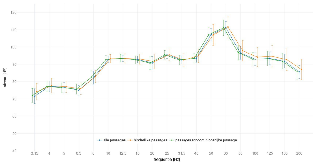
locatie Holten : gemiddeld spectrum passage met IC op spoor 1 meetlocatie: zuid 4m C | meetrichting: Z | voetbalk met +/- standaard afwijking
