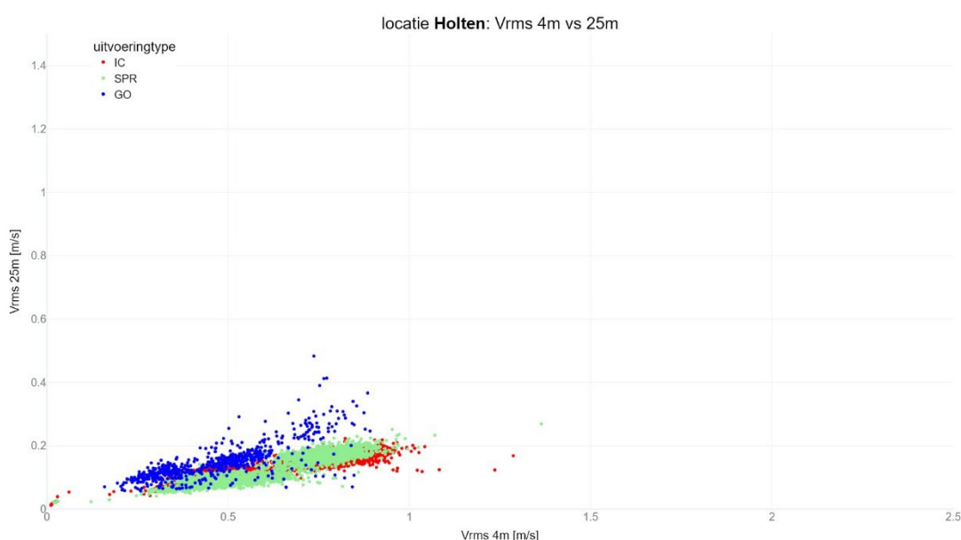
figuur 72 Verband tussen V_{rms} waarden op 4m en 25m
