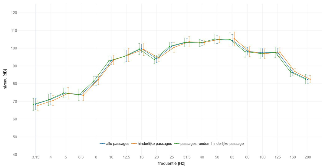
locatie Holten : gemiddeld spectrum passage met IC op spoor 2 meetlocatie: zuid 8m C | meetrichting: Z | voetbalk met +/- standaard afwijking
