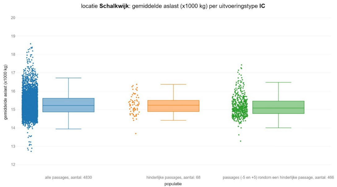
figuur 107 Gemiddelde aslast voor intercity's per populatie
