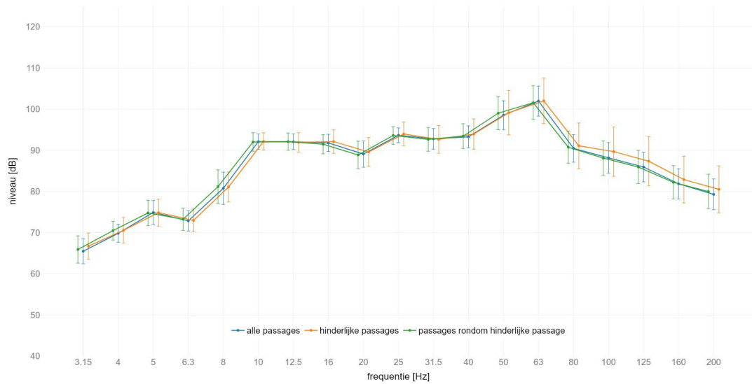
locatie Holten : gemiddeld spectrum passage met IC op spoor 1 meetlocatie: zuid 8m C | meetrichting: Y | voetbalk met +/- standaard afwijking
