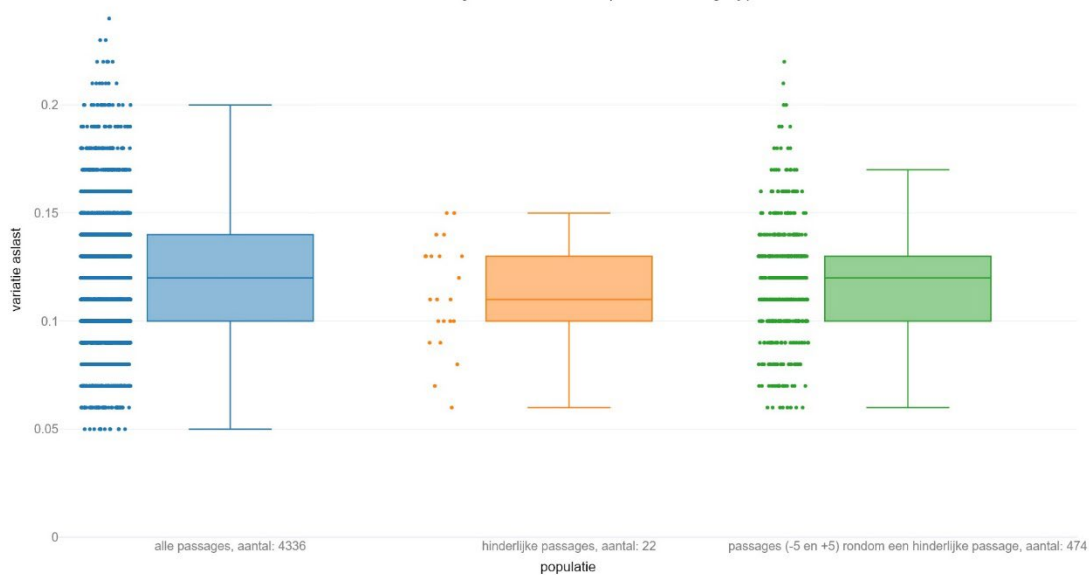
figuur 110 Variatie aslast voor sprinters per populatie
