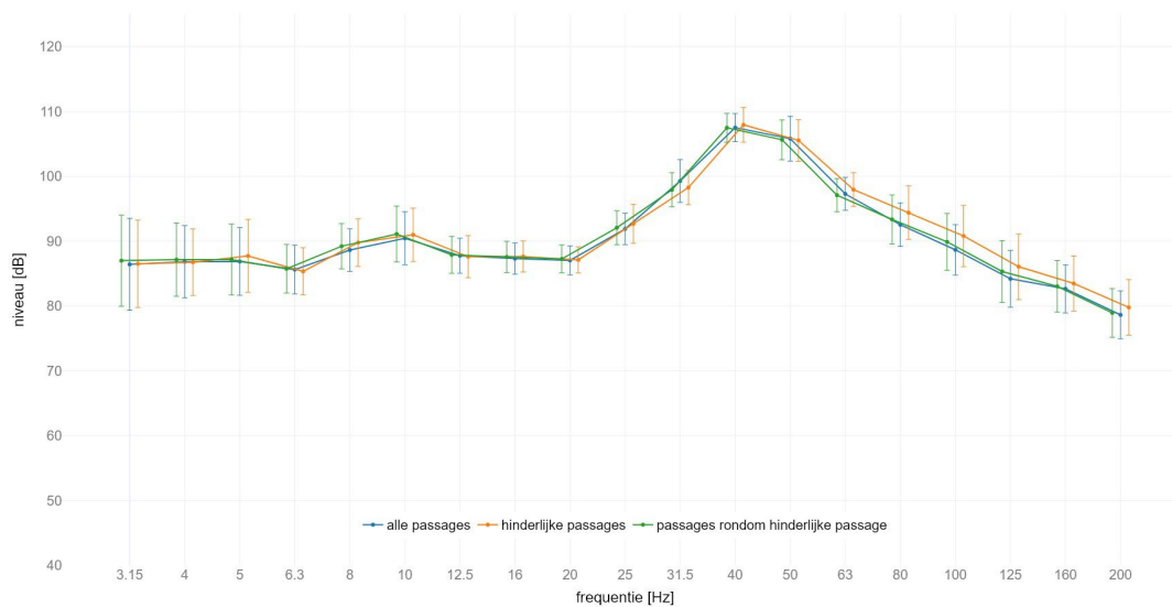
locatie America : gemiddeld spectrum passage met GO op spoor 1 meetlocatie: zuid 4m C | meetrichting: Z | foutbalk met +/- standaard afwijking
