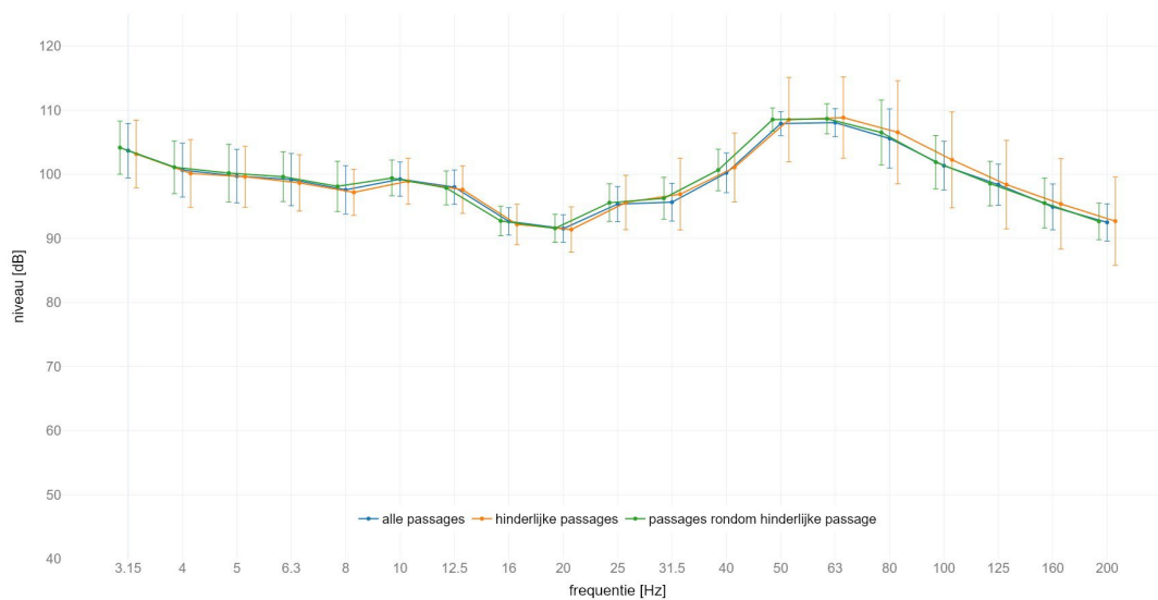
locatie Holten : gemiddeld spectrum passage met SPR op spoor 1 meetlocatie: noord 4m C meetrichting: Z | voetbalk met +/- standaard afwijking
