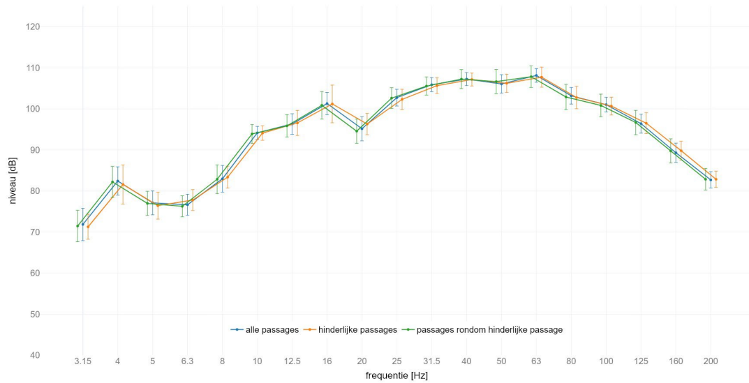
locatie Holten : gemiddeld spectrum passage met IC op spoor 2 meetlocatie: zuid 8m C | meetrichting: X | voetbalk met +/- standaard afwijking
