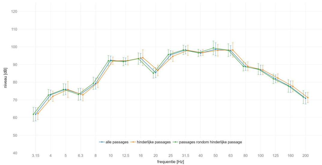
locatie Holten : gemiddeld spectrum passage met IC op spoor 2 meetlocatie: zuid 25m C | meetrichting: Y | foutbalk met +/- standaard afwijking
