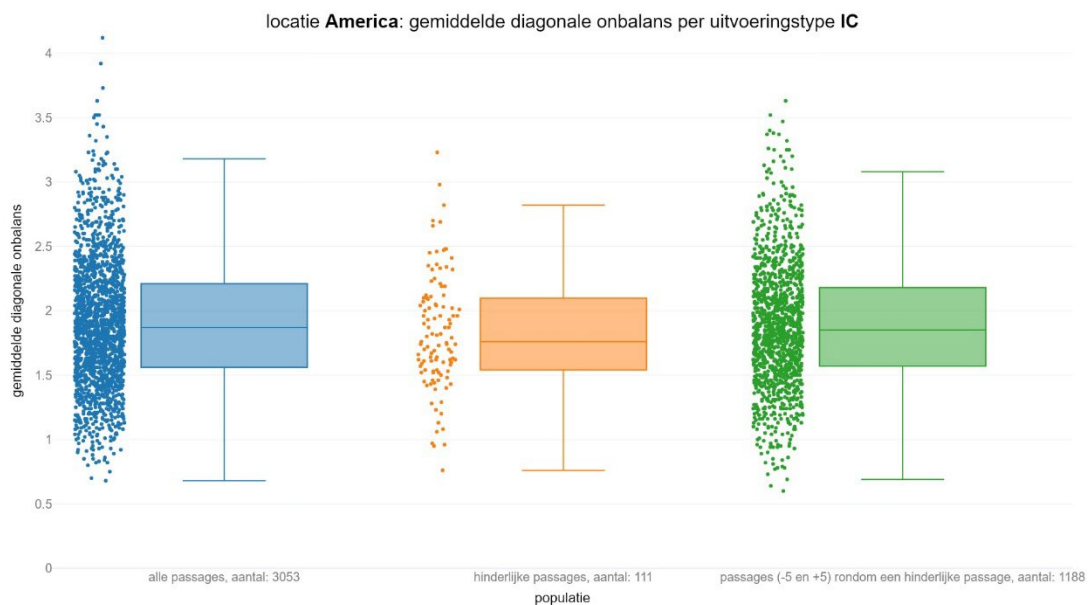
figuur 125 Gemiddelde diagonale onbalans voor intercity's per populatie
