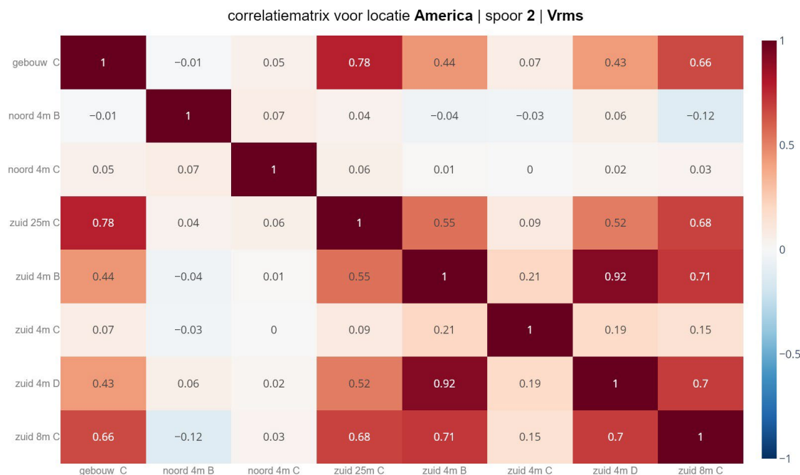
figuur 45 Correlatie matrix V_{rms} voor passage op spoor 2
