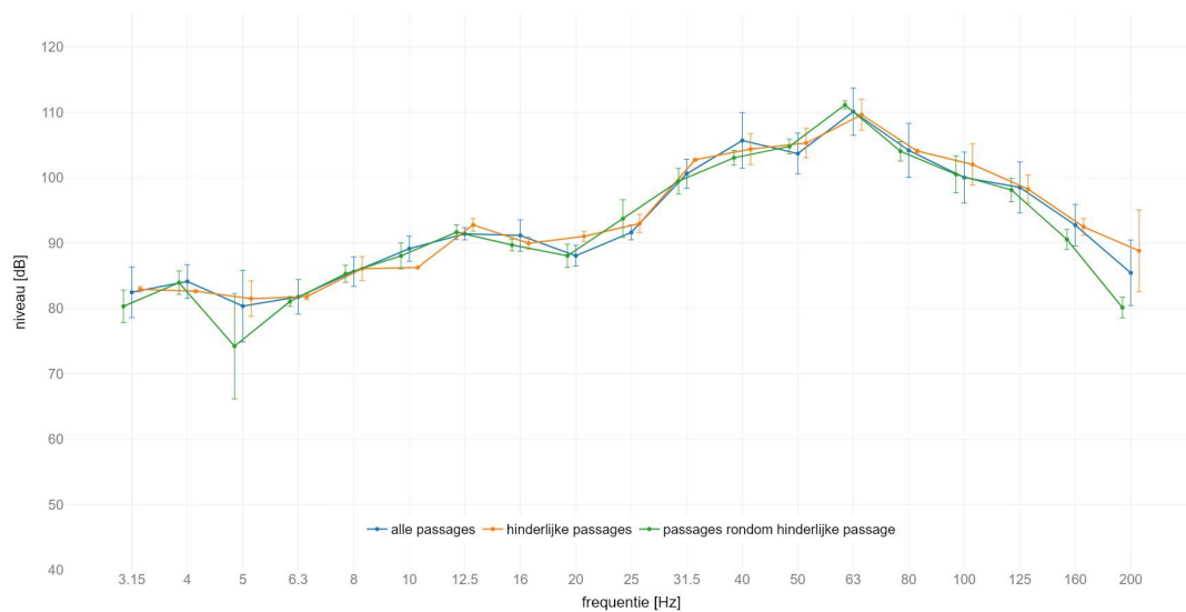
locatie America : gemiddeld spectrum passage met SPR op spoor 2 meetlocatie: zuid 4m D | meetrichting: Z | foutbalk met +/- standaard afwijking
