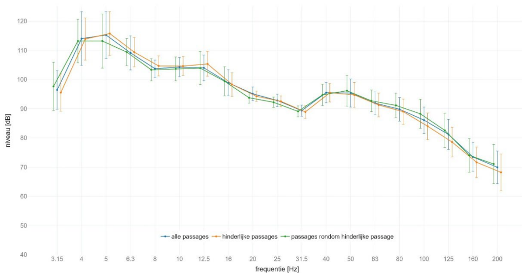
locatie Schalkwijk : gemiddeld spectrum passage met GO op spoor 1 meetlocatie: west 8m C | meetrichting: X | foutbalk met +/- standaard afwijking
