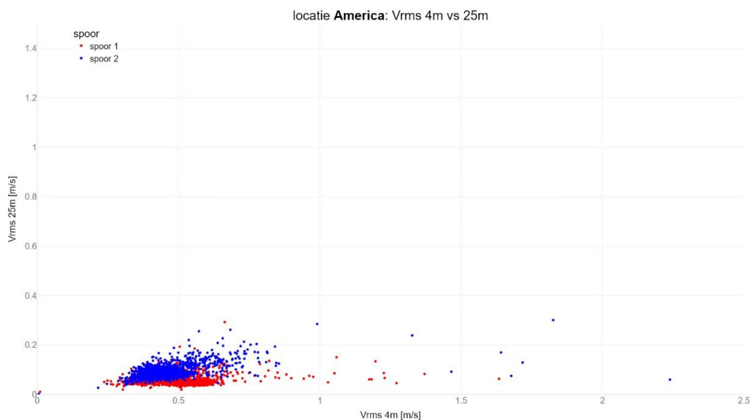
figuur 51 Verband tussen V_{rms} waarden op 4m en 25m voor passages over een bepaald spoor
