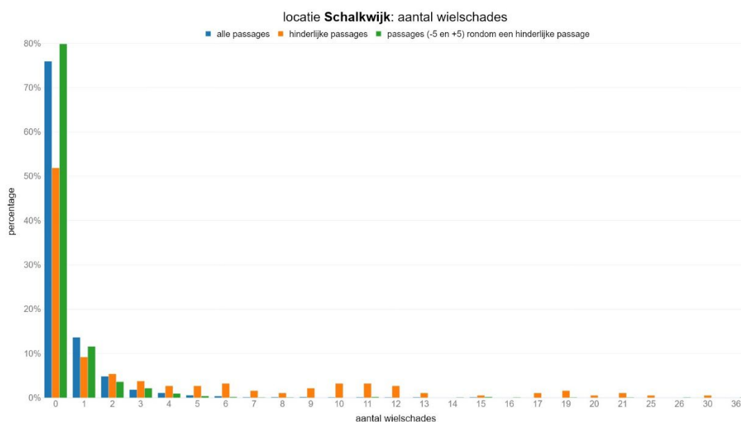
figuur 8 Aantal wielschades per populatie
