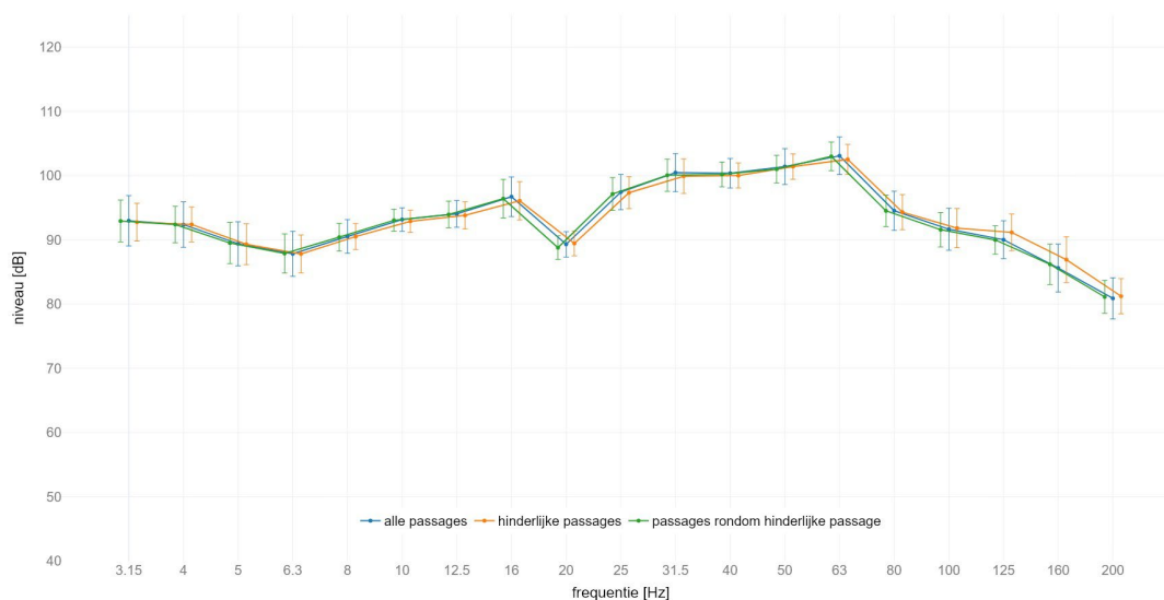
locatie Holten : gemiddeld spectrum passage met SPR op spoor 2 meetlocatie: noord 4m C | meetrichting: Y | voetbalk met +/- standaard afwijking
