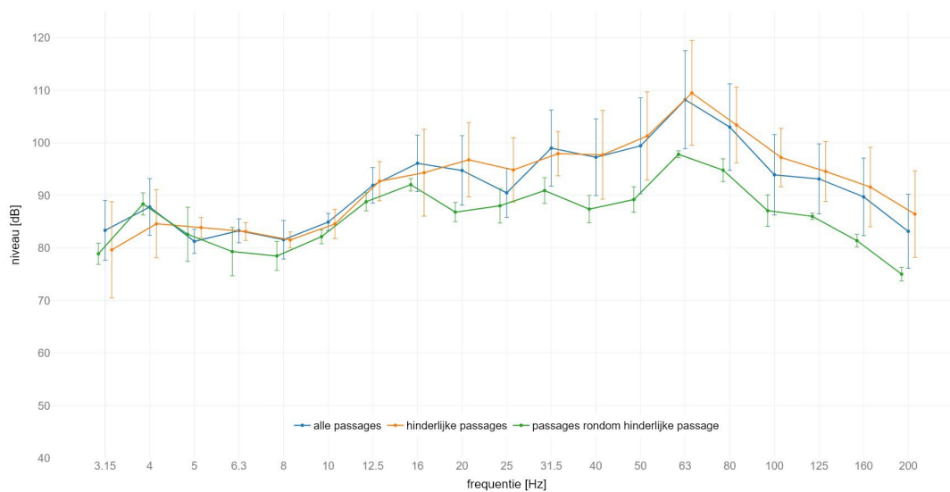
locatie America : gemiddeld spectrum passage met SPR op spoor 2 meetlocatie: zuid 4m C | meetrichting: Y | foutbalk met +/- standaard afwijking
