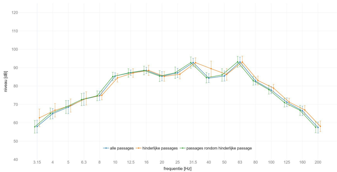
locatie America : gemiddeld spectrum passage met IC op spoor 2 meetlocatie: zuid 25m C | meetrichting: Y | foutbalk met +/- standaard afwijking
