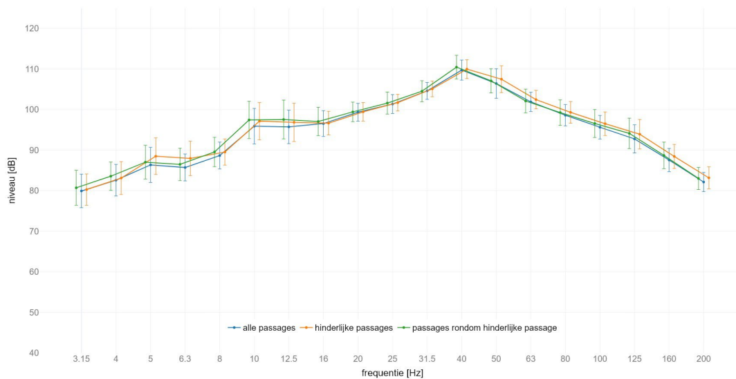
locatie Holten : gemiddeld spectrum passage met GO op spoor 2 meetlocatie: zuid 8m C | meetrichting: Y | foutbalk met +/- standaard afwijking
