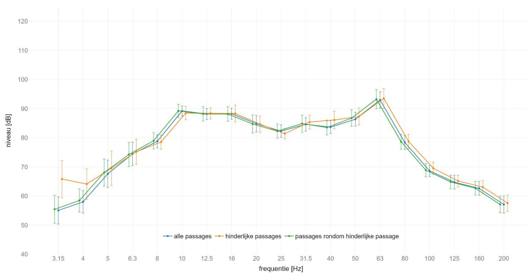
locatie America : gemiddeld spectrum passage met SPR op spoor 2 meetlocatie: noord 4m B | meetrichting: Z | foutbalk met +/- standaard afwijking
