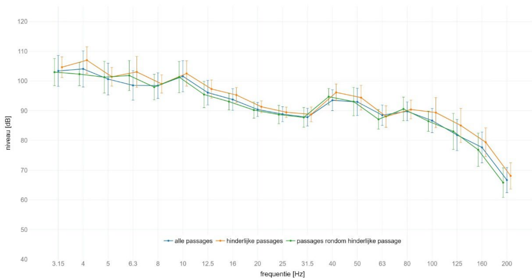
locatie Schalkwijk : gemiddeld spectrum passage met GO op spoor 2 meetlocatie: oost 4m C | meetrichting: Z | foute balk met +/- standaard afwijking
