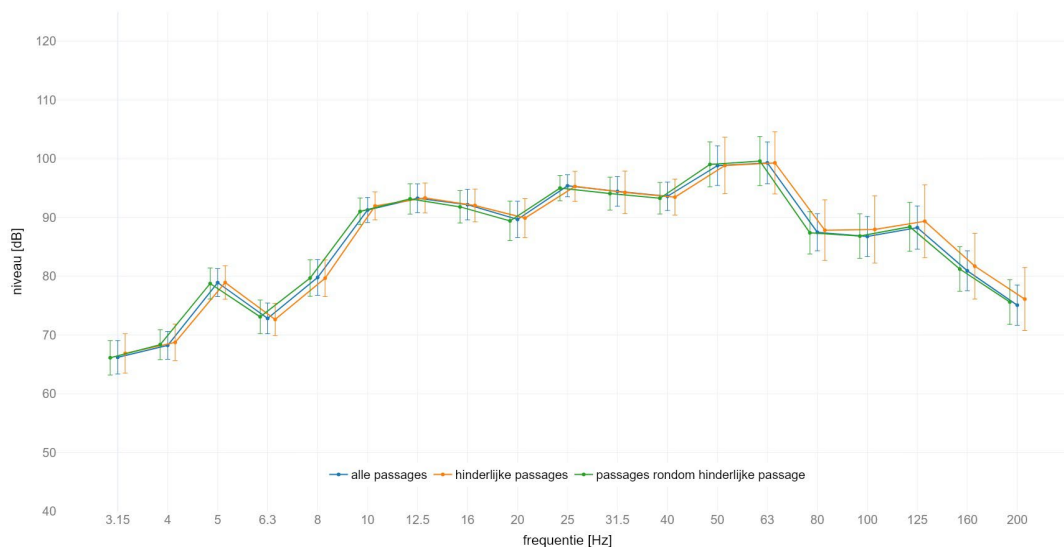
locatie Holten : gemiddeld spectrum passage met IC op spoor 1 meetlocatie: zuid 25m C | meetrichting: X | voetbalk met +/- standaard afwijking
