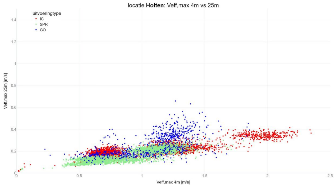
figuur 73 Verband tussen V_{eff,max} waardes op 4m en 25m
