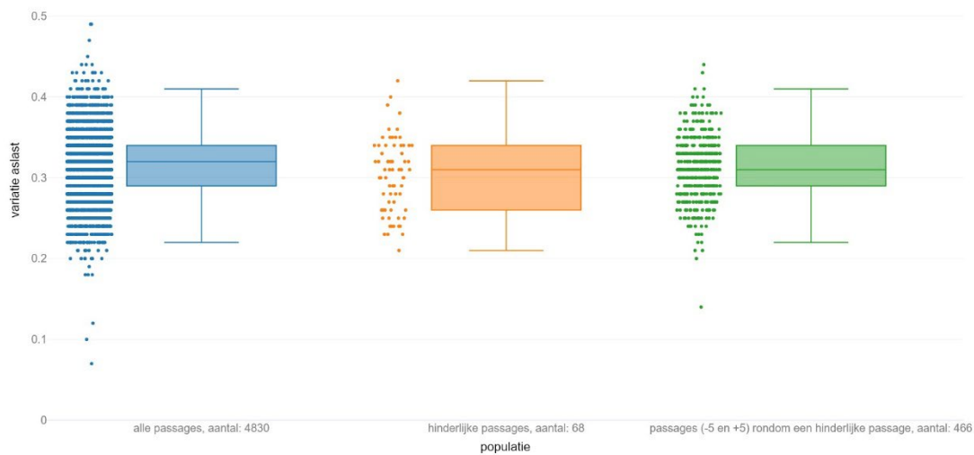
figuur 109 Variatie aslast voor intercity's per populatie
